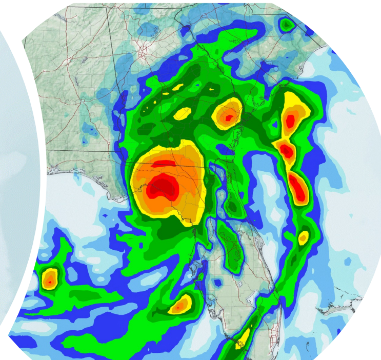
GEOS-FP 12km L72 963 hPa : 73 Kt
