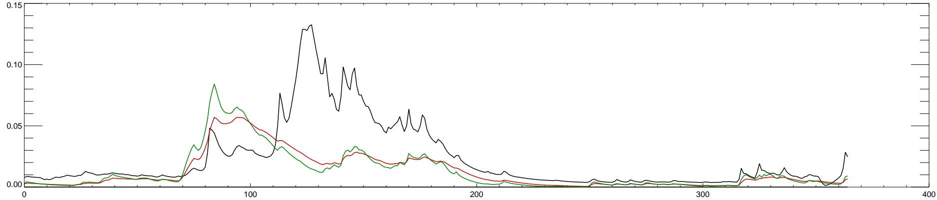
13337000 LOCHSA RIVER NR LOWELL ID : 1998
