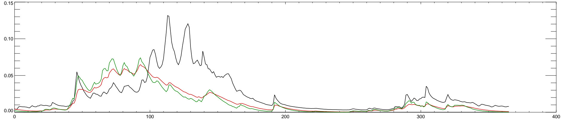
13337000 LOCHSA RIVER NR LOWELL ID : 2016
