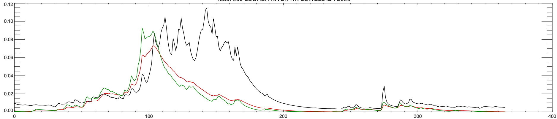
13337000 LOCHSA RIVER NR LOWELL ID : 2001
