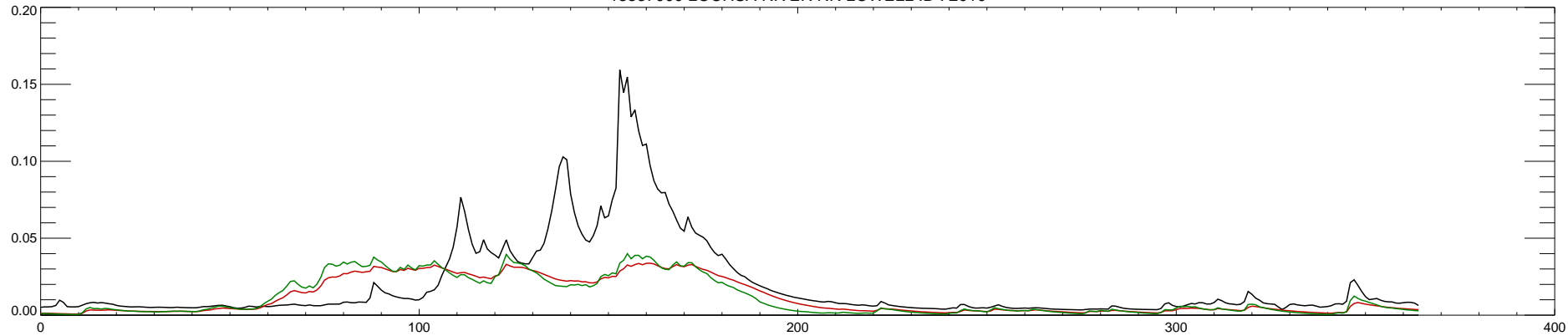
13337000 LOCHSA RIVER NR LOWELL ID : 2010
