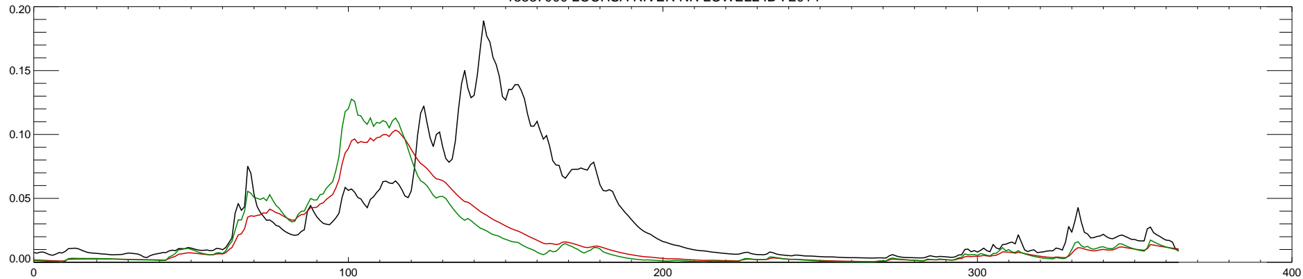
13337000 LOCHSA RIVER NR LOWELL ID : 2015
