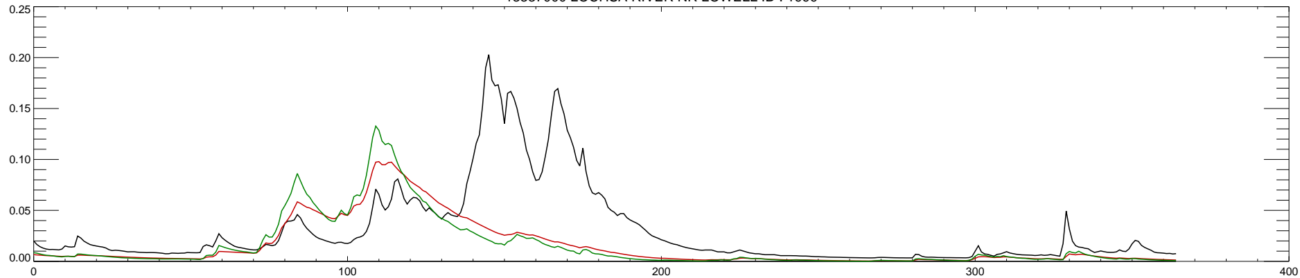
13337000 LOCHSA RIVER NR LOWELL ID : 2000
