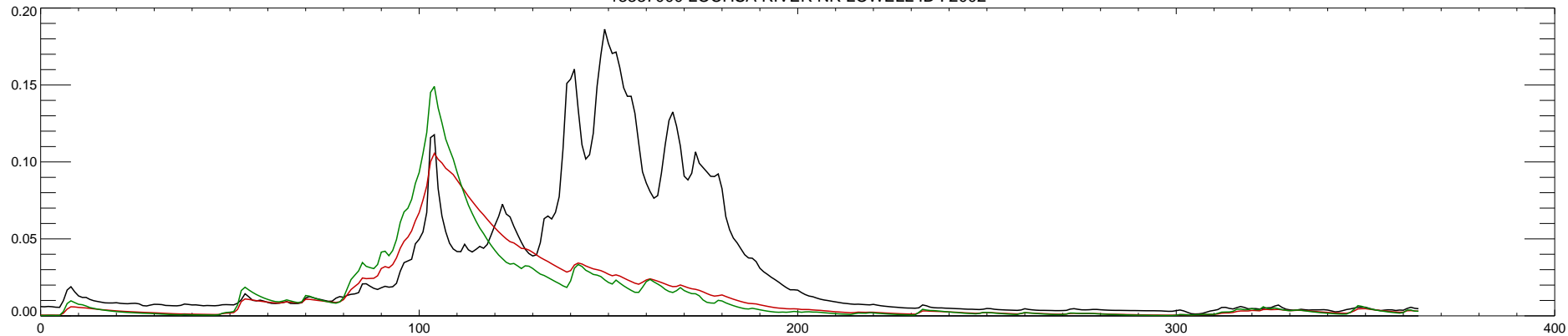
13337000 LOCHSA RIVER NR LOWELL ID : 2003
