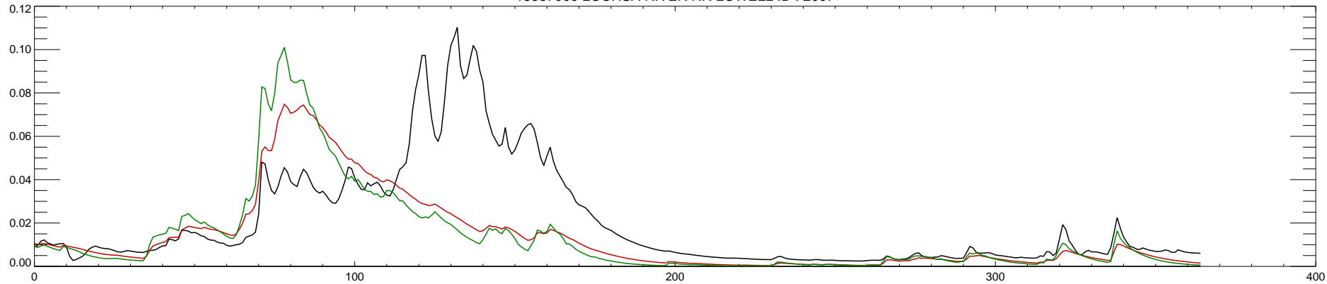
13337000 LOCHSA RIVER NR LOWELL ID : 2007
