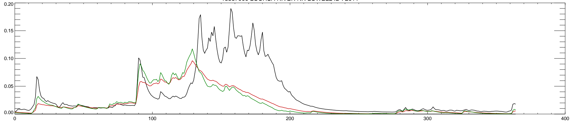
13337000 LOCHSA RIVER NR LOWELL ID : 2012
