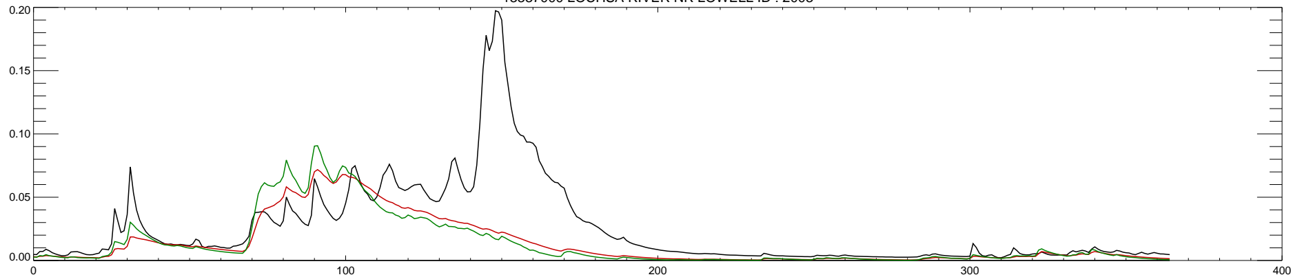
13337000 LOCHSA RIVER NR LOWELL ID : 2004
