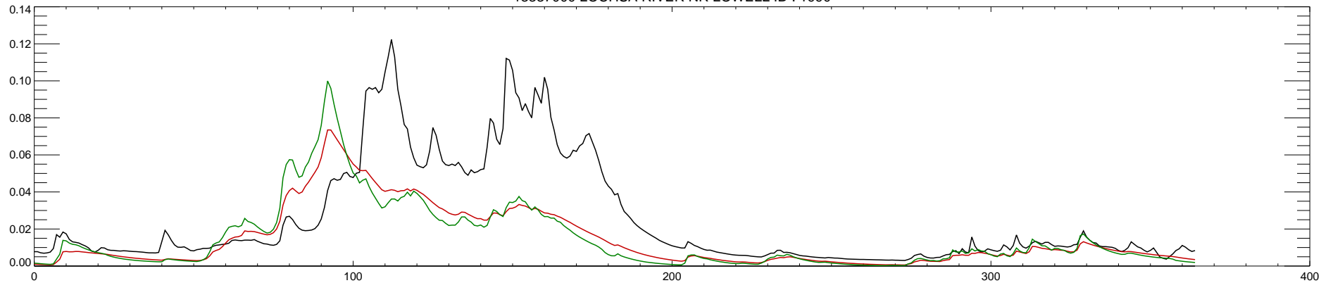
13337000 LOCHSA RIVER NR LOWELL ID : 1991
