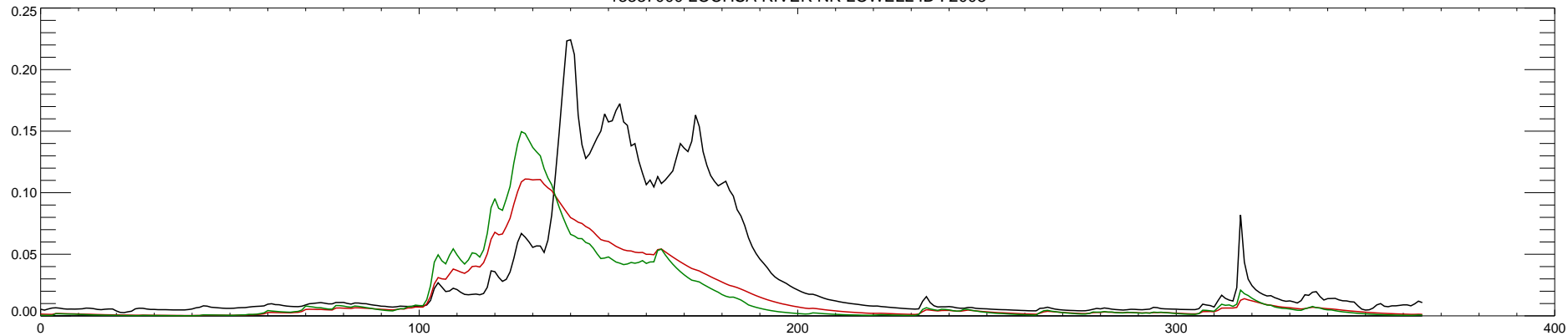
13337000 LOCHSA RIVER NR LOWELL ID : 2009
