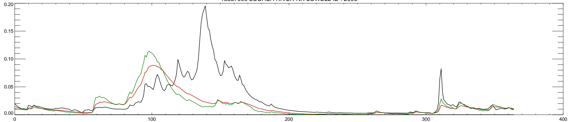
13337000 LOCHSA RIVER NR LOWELL ID : 2007
