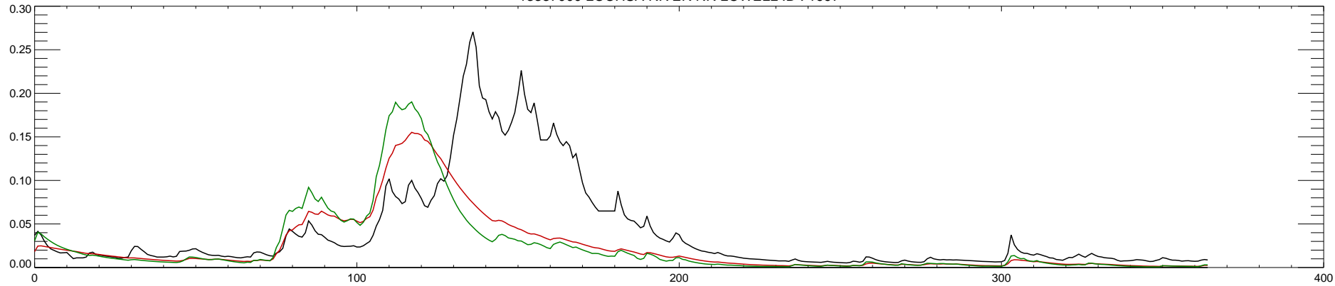
13337000 LOCHSA RIVER NR LOWELL ID : 1998
