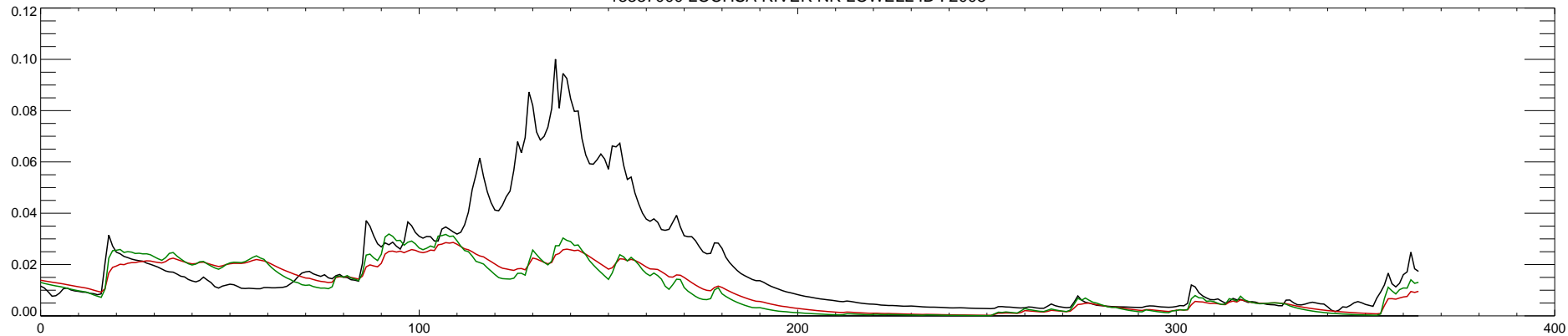
13337000 LOCHSA RIVER NR LOWELL ID : 2006
