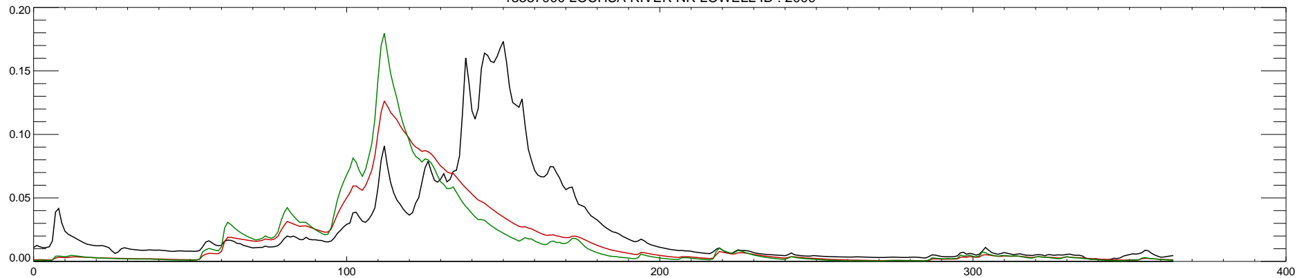
13337000 LOCHSA RIVER NR LOWELL ID : 2010
