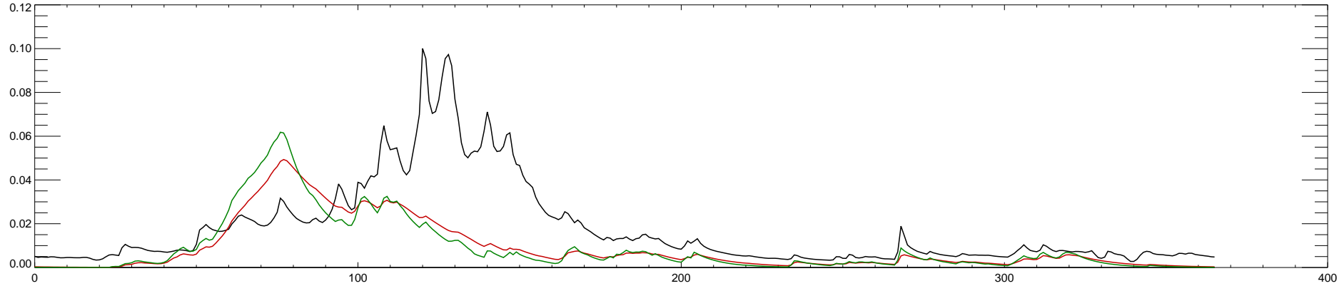
13337000 LOCHSA RIVER NR LOWELL ID : 1992
