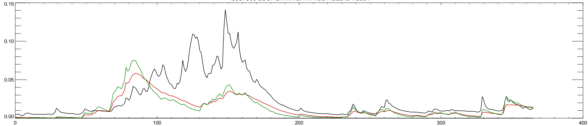
13337000 LOCHSA RIVER NR LOWELL ID : 2004
