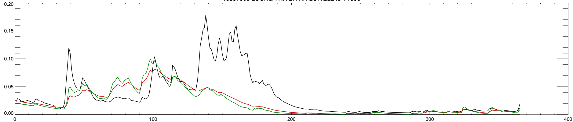
13337000 LOCHSA RIVER NR LOWELL ID : 1997
