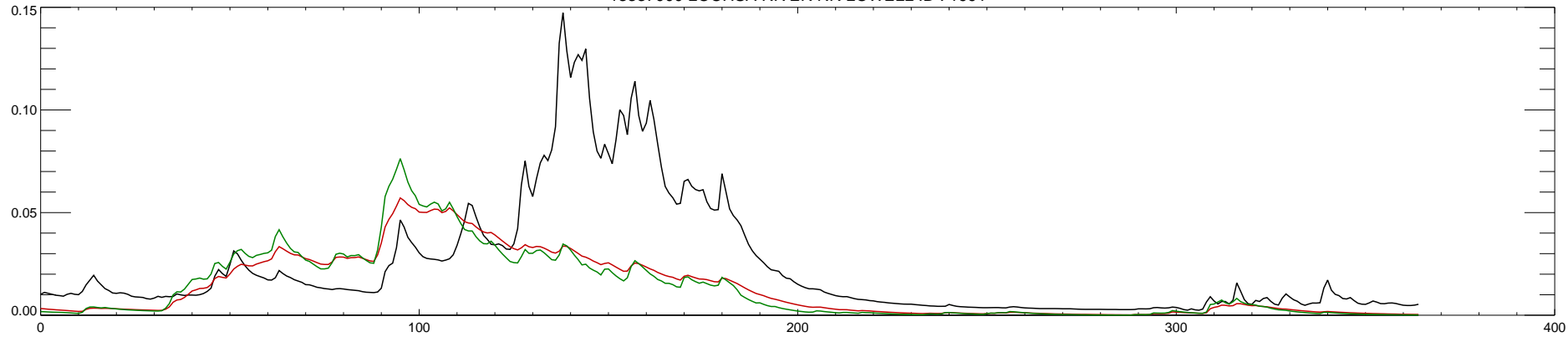
13337000 LOCHSA RIVER NR LOWELL ID : 1992
