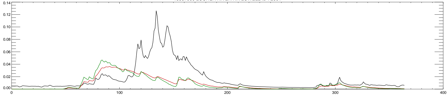
13337000 LOCHSA RIVER NR LOWELL ID : 2001
