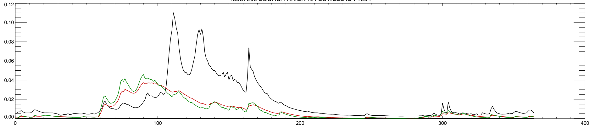
13337000 LOCHSA RIVER NR LOWELL ID : 1995
