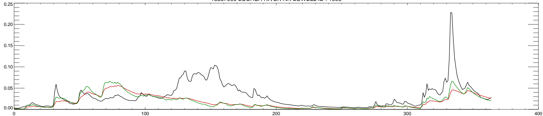
13337000 LOCHSA RIVER NR LOWELL ID : 1995
