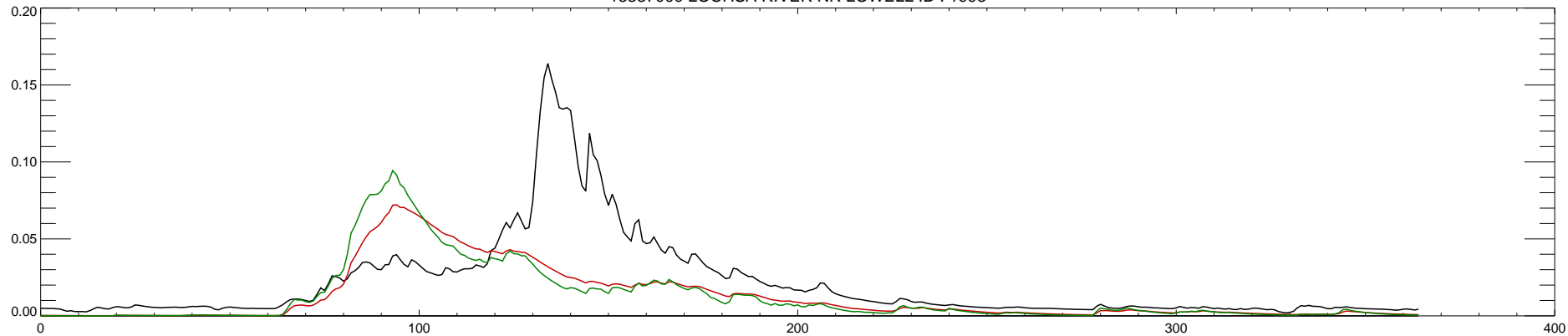
13337000 LOCHSA RIVER NR LOWELL ID : 1994
