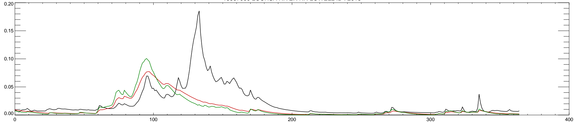
13337000 LOCHSA RIVER NR LOWELL ID : 2013
