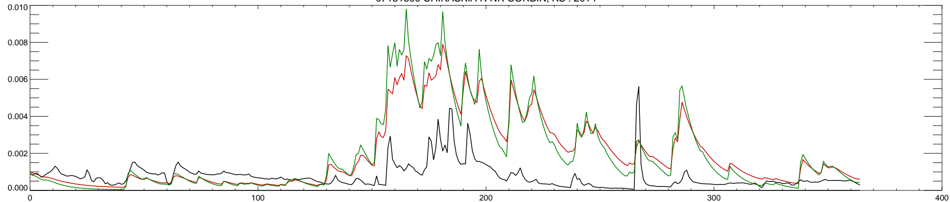
07151500 CHIKASKIA R NR CORBIN, KS : 2015
