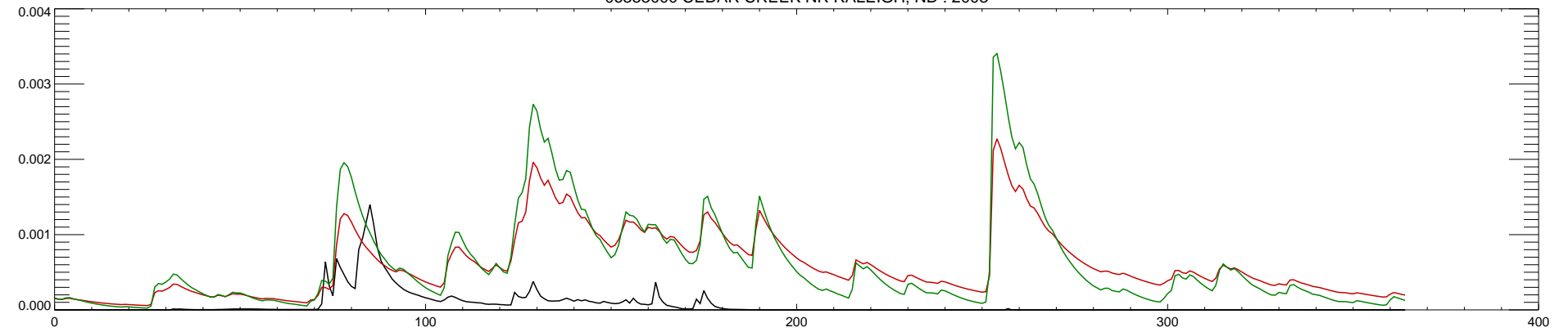
06353000 CEDAR CREEK NR RALEIGH, ND : 2004
