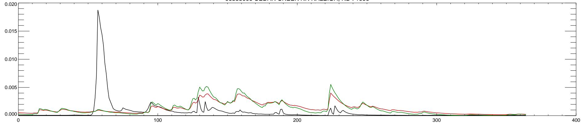
06353000 CEDAR CREEK NR RALEIGH, ND : 2000
