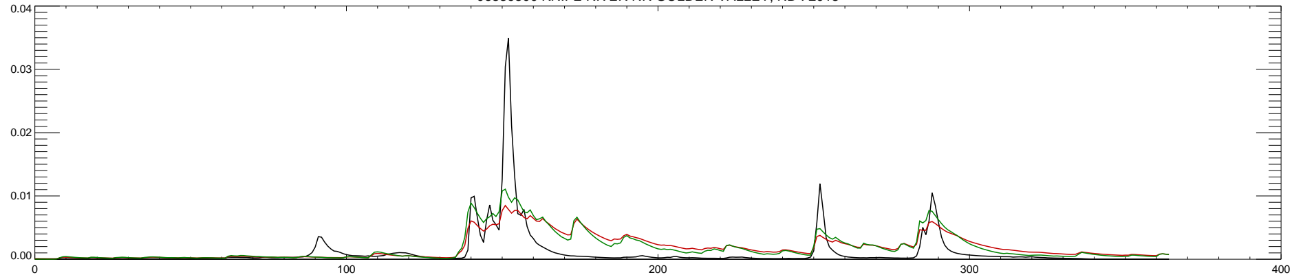
06339500 KNIFE RIVER NR GOLDEN VALLEY, ND : 2013
