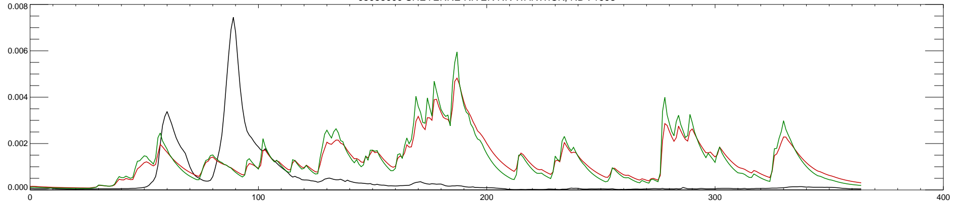
05056000 SHEYENNE RIVER NR WARWICK, ND : 1998
