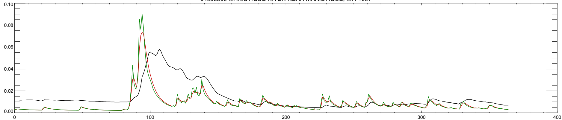
04056500 MANISTIQUE RIVER NEAR MANISTIQUE, MI : 1998
