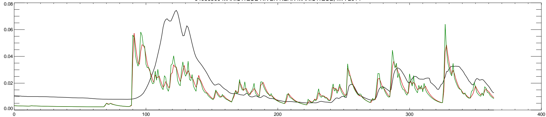
04056500 MANISTIQUE RIVER NEAR MANISTIQUE, MI : 2015
