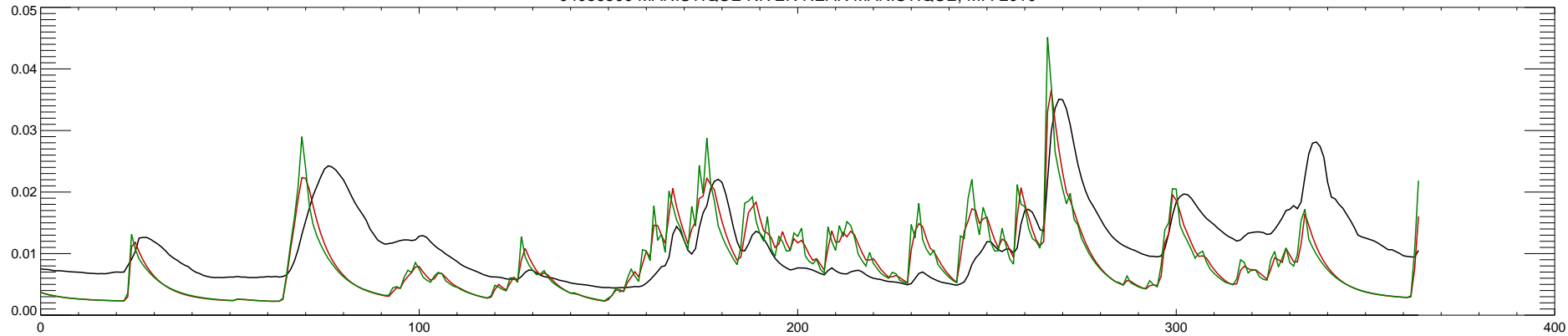
04056500 MANISTIQUE RIVER NEAR MANISTIQUE, MI : 2010
