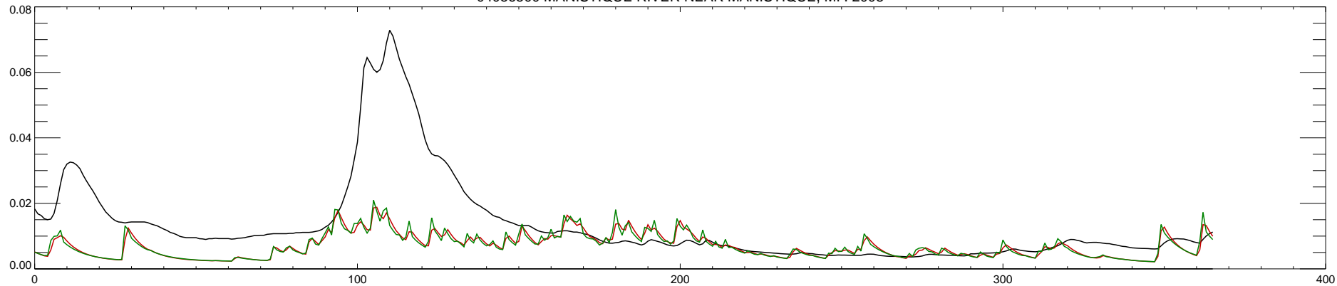
04056500 MANISTIQUE RIVER NEAR MANISTIQUE, MI : 2009
