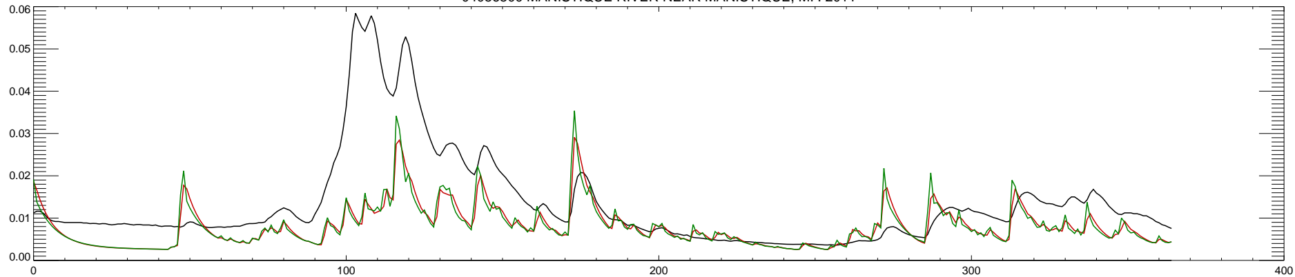
04056500 MANISTIQUE RIVER NEAR MANISTIQUE, MI : 2012
