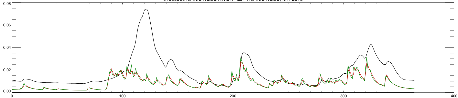
04056500 MANISTIQUE RIVER NEAR MANISTIQUE, MI : 2013
