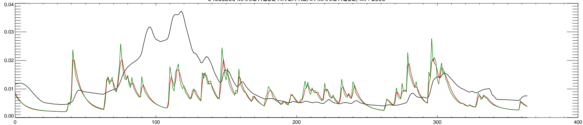
04056500 MANISTIQUE RIVER NEAR MANISTIQUE, MI : 2010
