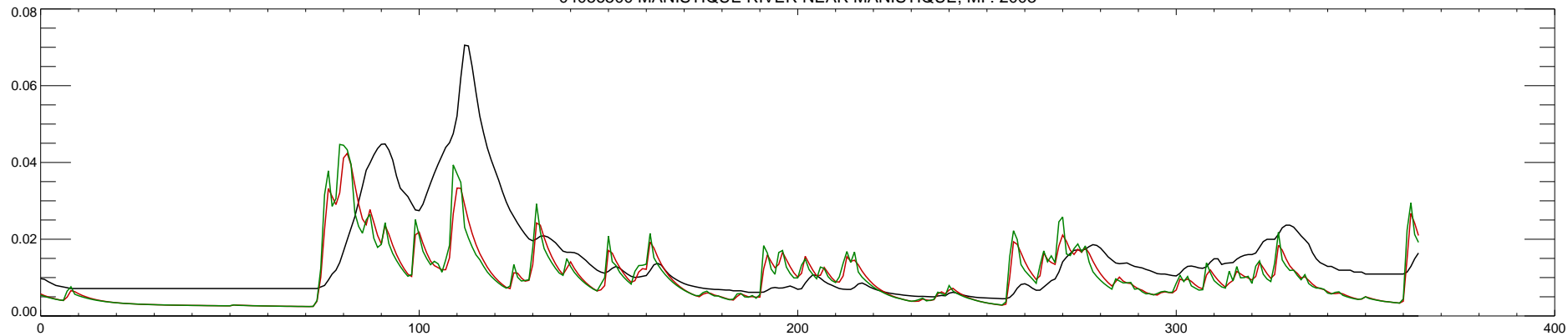
04056500 MANISTIQUE RIVER NEAR MANISTIQUE, MI : 2004
