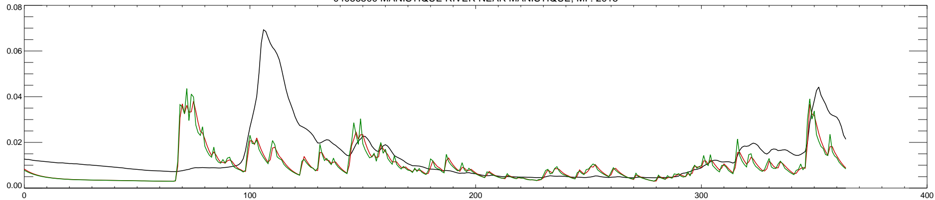
04056500 MANISTIQUE RIVER NEAR MANISTIQUE, MI : 2016
