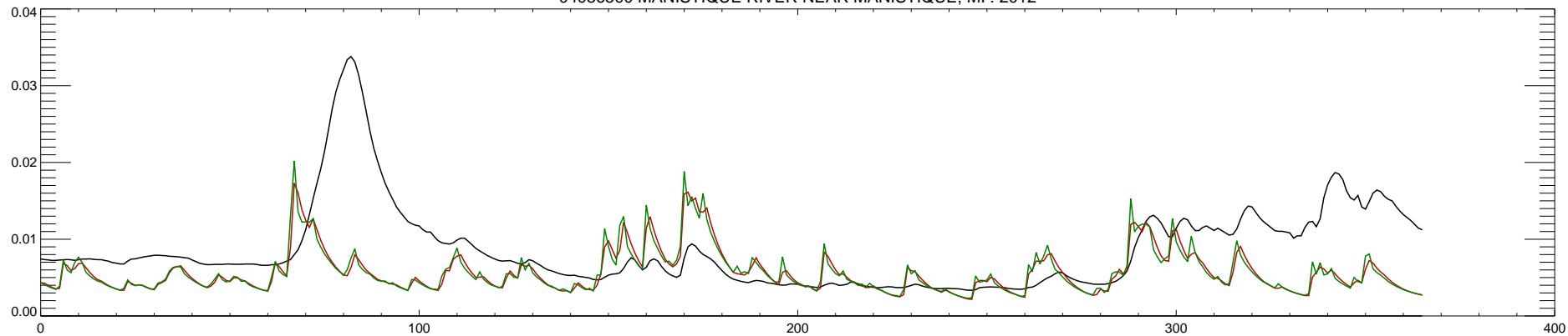
04056500 MANISTIQUE RIVER NEAR MANISTIQUE, MI : 2013
