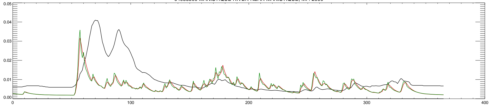
04056500 MANISTIQUE RIVER NEAR MANISTIQUE, MI : 2001
