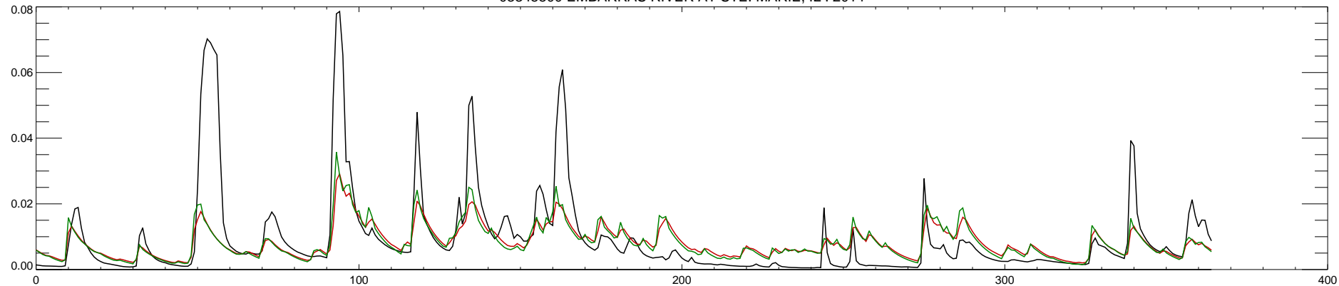
03345500 EMBARRAS RIVER AT STE. MARIE, IL : 2015
