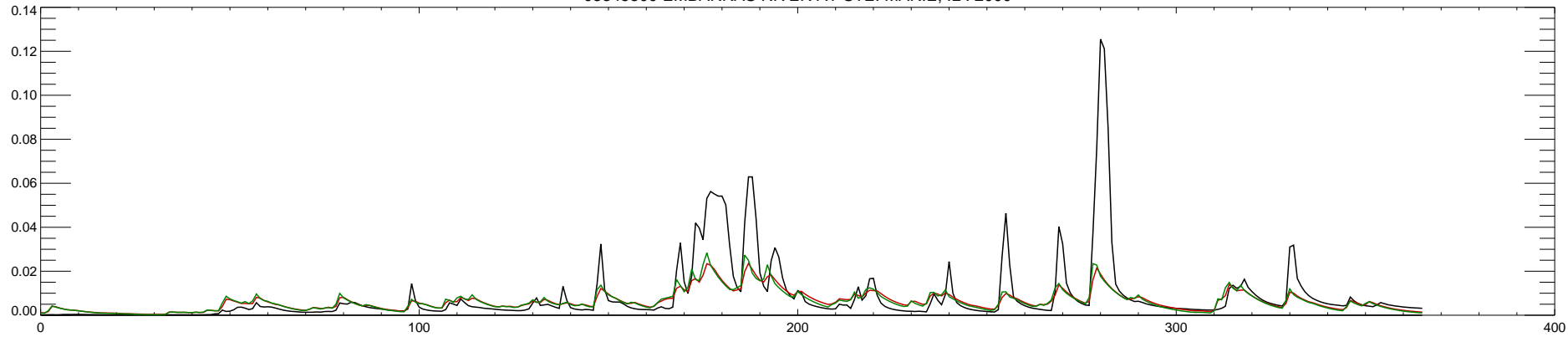
03345500 EMBARRAS RIVER AT STE. MARIE, IL : 2001
