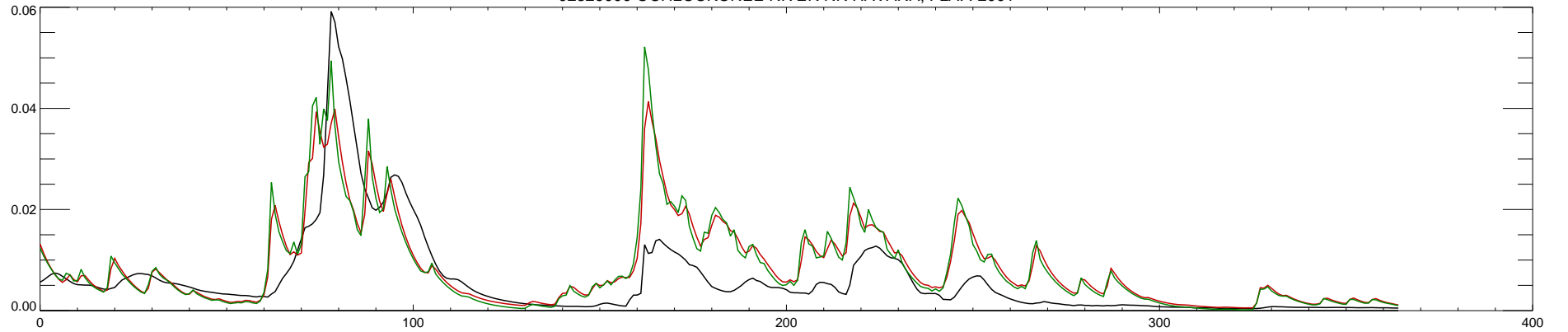
02329000 OCHLOCKONEE RIVER NR HAVANA, FLA. : 2001
