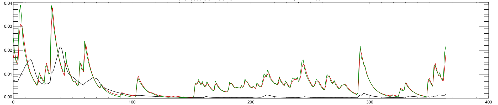
02329000 OCHLOCKONEE RIVER NR HAVANA, FLA. : 2007
