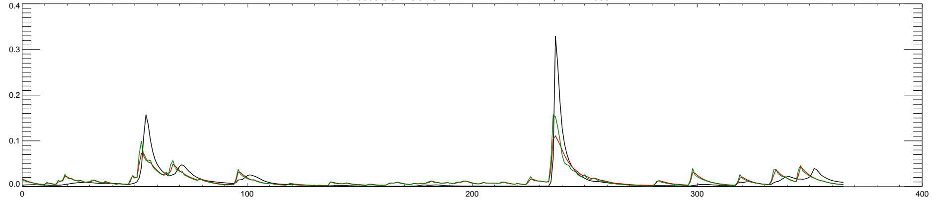
02329000 OCHLOCKONEE RIVER NR HAVANA, FLA. : 2009
