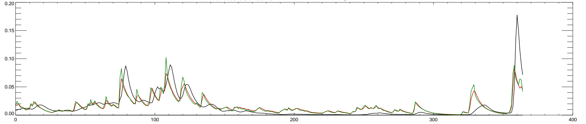
02329000 OCHLOCKONEE RIVER NR HAVANA, FLA. : 2015
