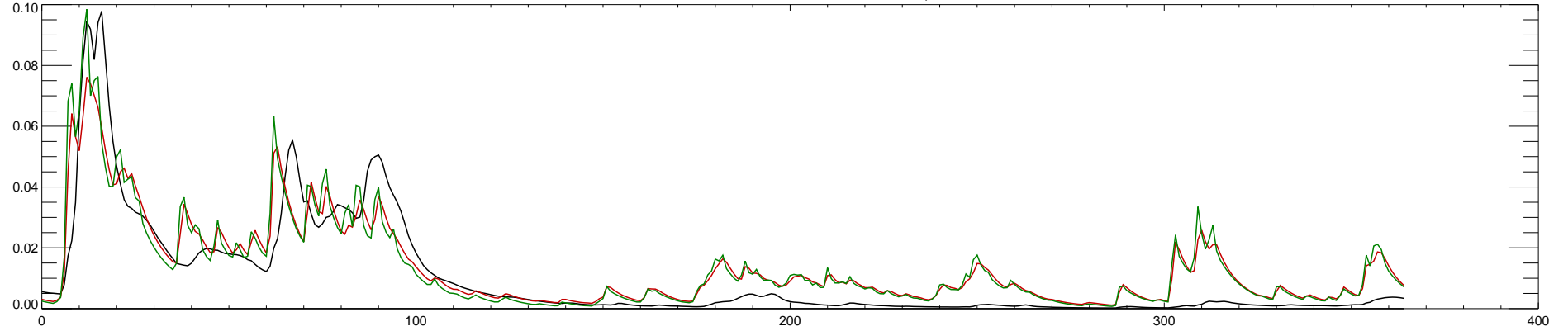
02329000 OCHLOCKONEE RIVER NR HAVANA, FLA. : 1994
