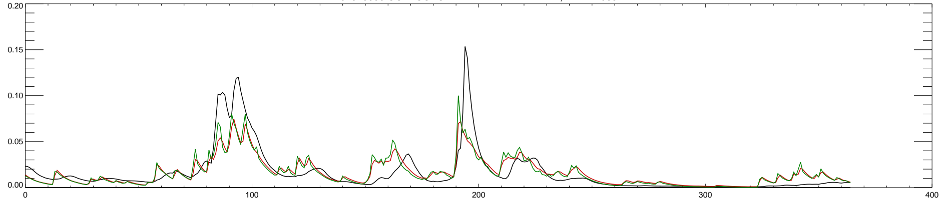
02329000 OCHLOCKONEE RIVER NR HAVANA, FLA. : 2006
