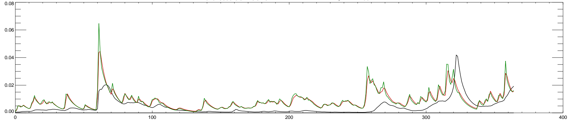
02329000 OCHLOCKONEE RIVER NR HAVANA, FLA. : 2003
