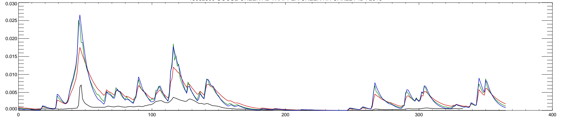
13082500 GOOSE CREEK AB TRAPPER CREEK NR OAKLEY ID : 2016
