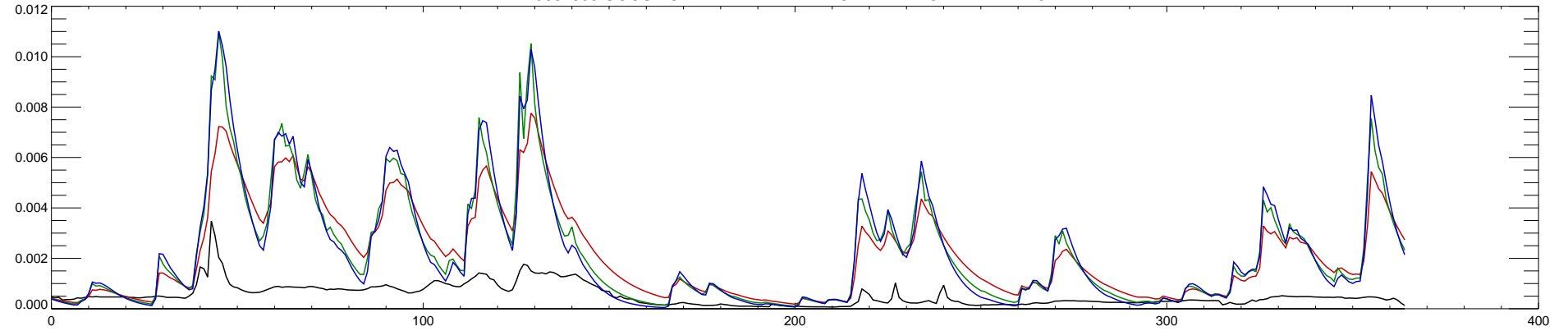
13082500 GOOSE CREEK AB TRAPPER CREEK NR OAKLEY ID : 2015
