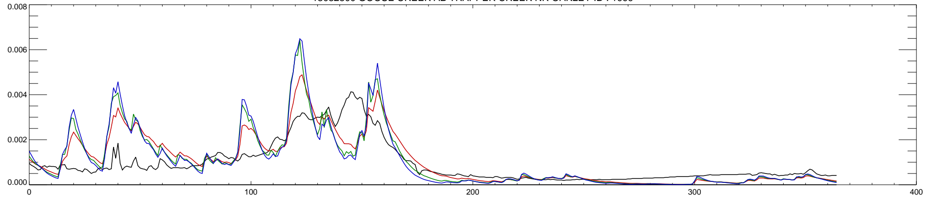
13082500 GOOSE CREEK AB TRAPPER CREEK NR OAKLEY ID : 2000
