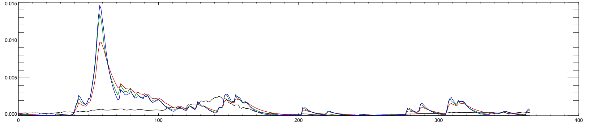
13082500 GOOSE CREEK AB TRAPPER CREEK NR OAKLEY ID : 2009
