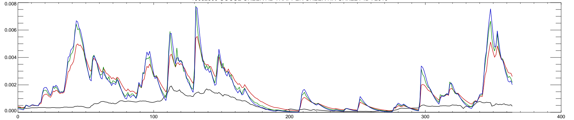
13082500 GOOSE CREEK AB TRAPPER CREEK NR OAKLEY ID : 2010
