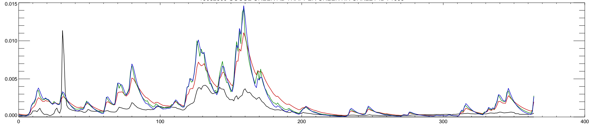
13082500 GOOSE CREEK AB TRAPPER CREEK NR OAKLEY ID : 1995
