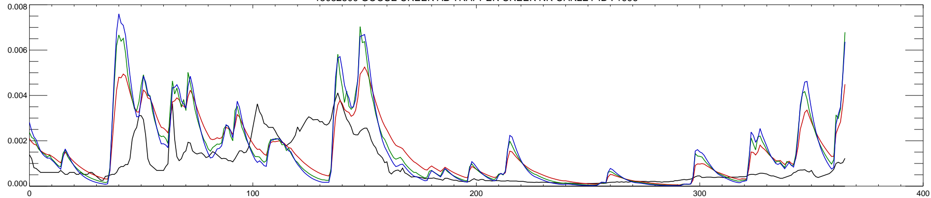
13082500 GOOSE CREEK AB TRAPPER CREEK NR OAKLEY ID : 1997
