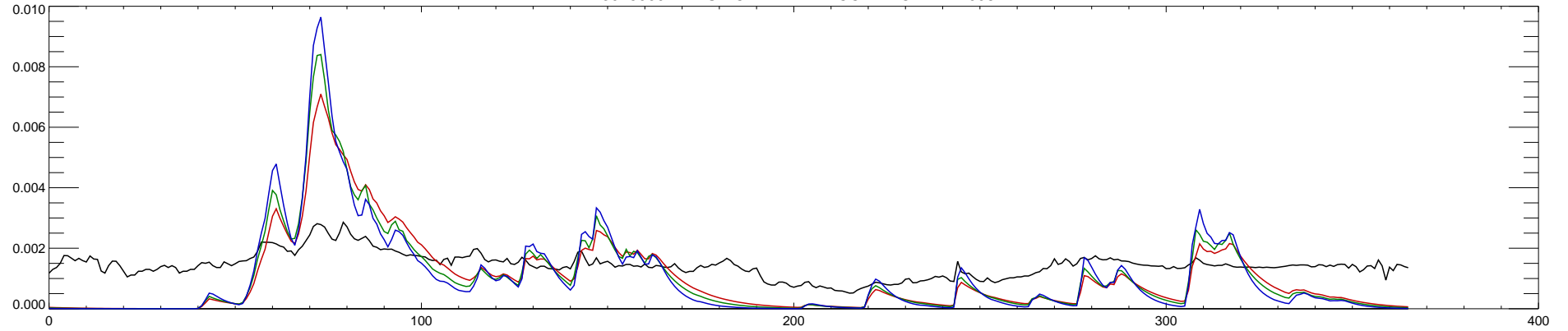
13075000 MARSH CREEK NR MCCAMMON ID : 2009
