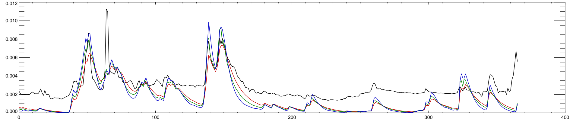
13075000 MARSH CREEK NR MCCAMMON ID : 1997
