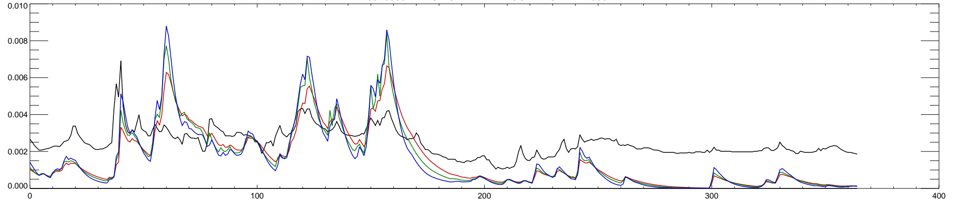
13075000 MARSH CREEK NR MCCAMMON ID : 2000
