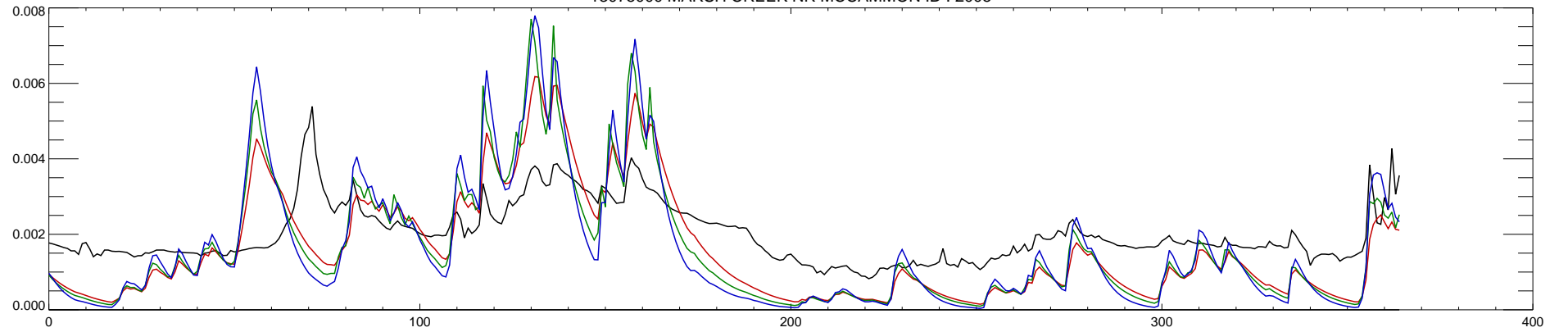
13075000 MARSH CREEK NR MCCAMMON ID : 2006
