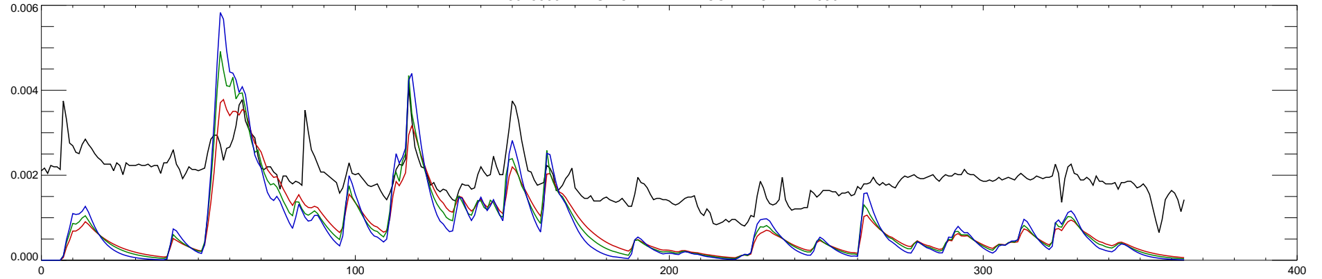
13075000 MARSH CREEK NR MCCAMMON ID : 1991
