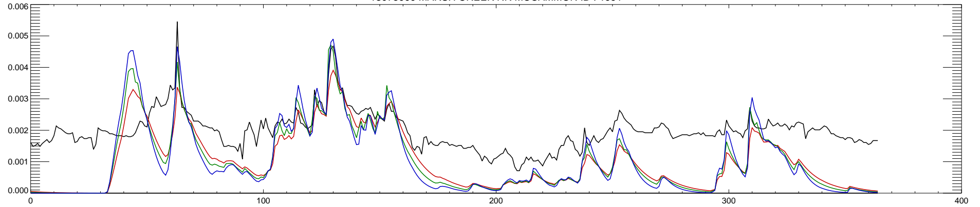
13075000 MARSH CREEK NR MCCAMMON ID : 1992
