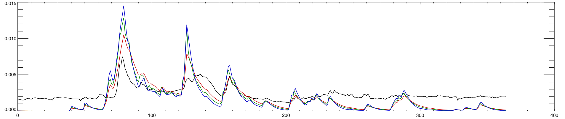
13075000 MARSH CREEK NR MCCAMMON ID : 1994
