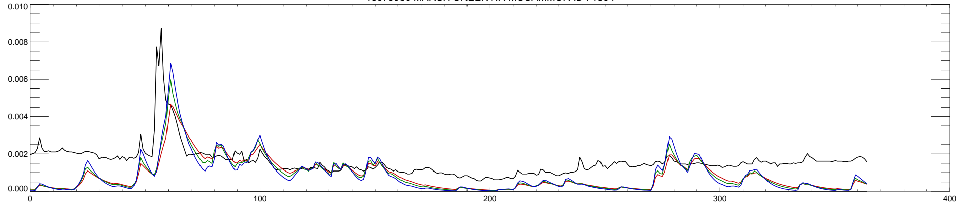
13075000 MARSH CREEK NR MCCAMMON ID : 1995
