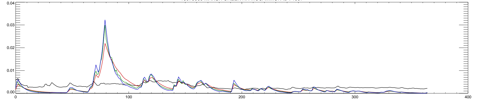
13075000 MARSH CREEK NR MCCAMMON ID : 1998
