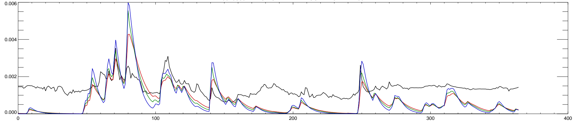
13075000 MARSH CREEK NR MCCAMMON ID : 2003
