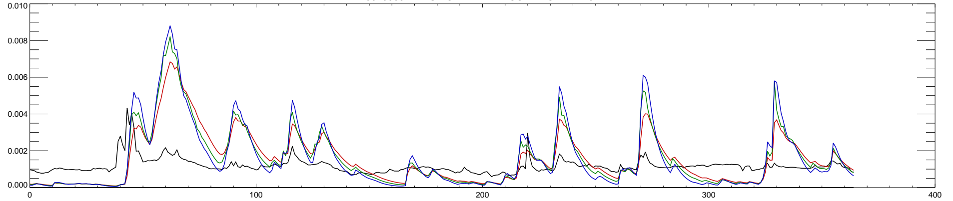
13075000 MARSH CREEK NR MCCAMMON ID : 2015
