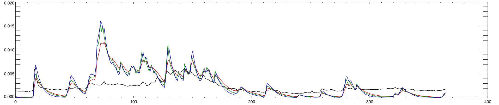
13075000 MARSH CREEK NR MCCAMMON ID : 2012
