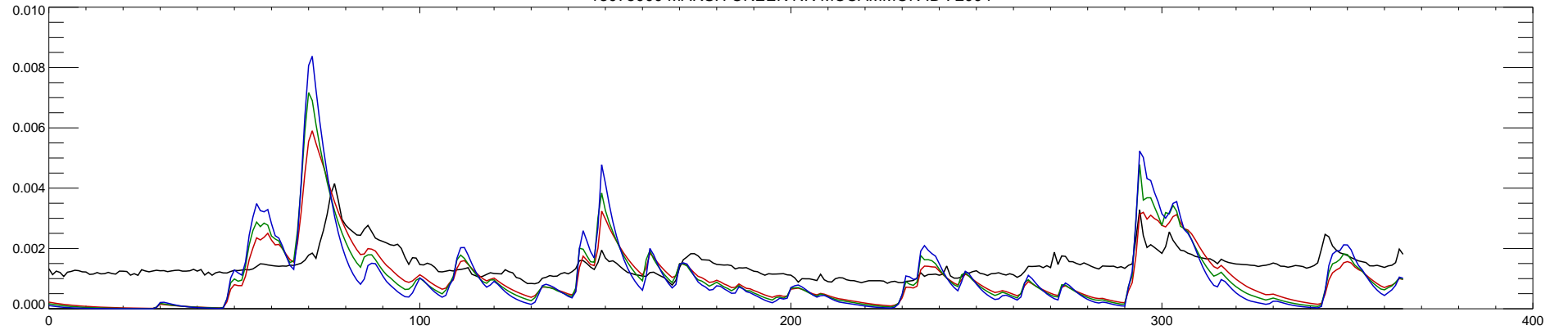
13075000 MARSH CREEK NR MCCAMMON ID : 2004
