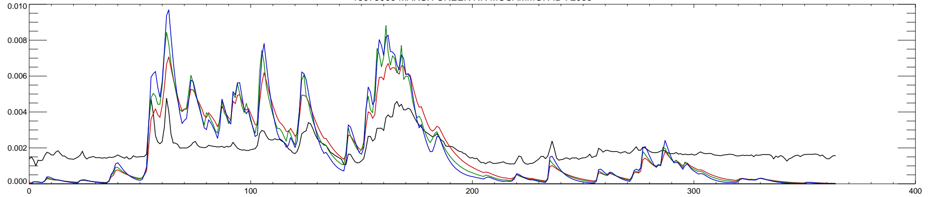
13075000 MARSH CREEK NR MCCAMMON ID : 2010
