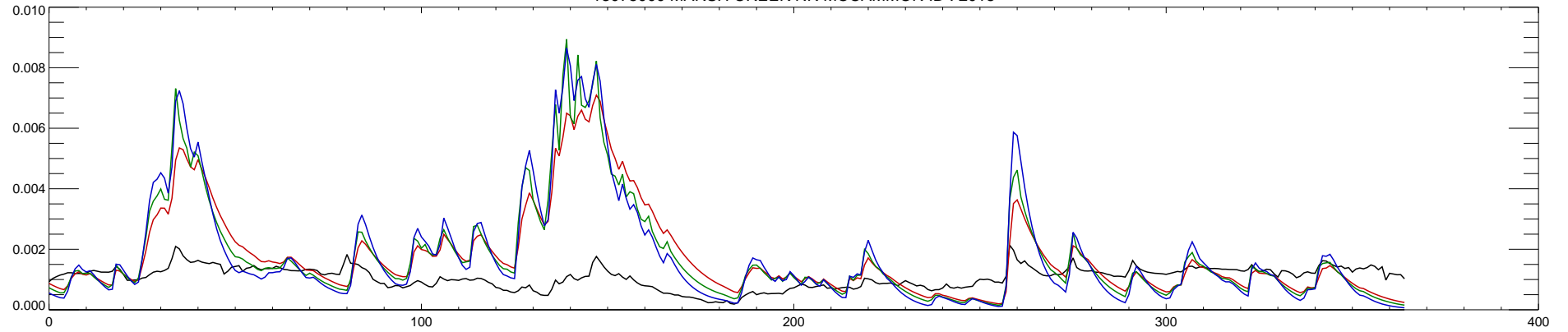
13075000 MARSH CREEK NR MCCAMMON ID : 2016
