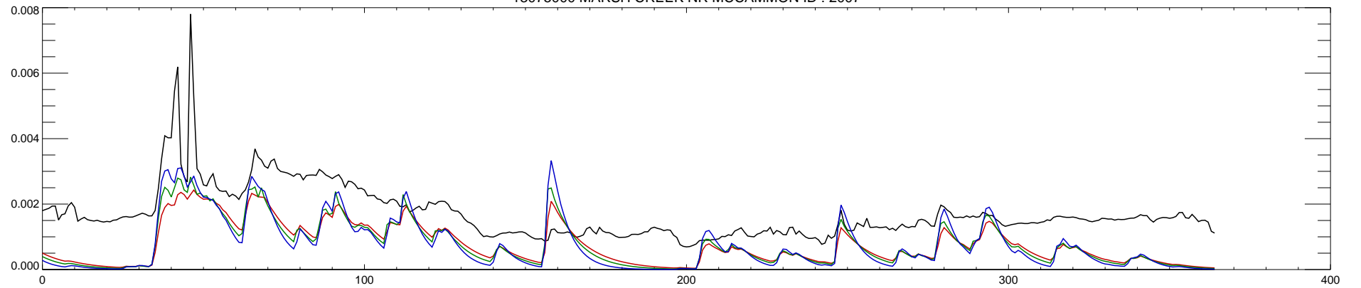
13075000 MARSH CREEK NR MCCAMMON ID : 2007
