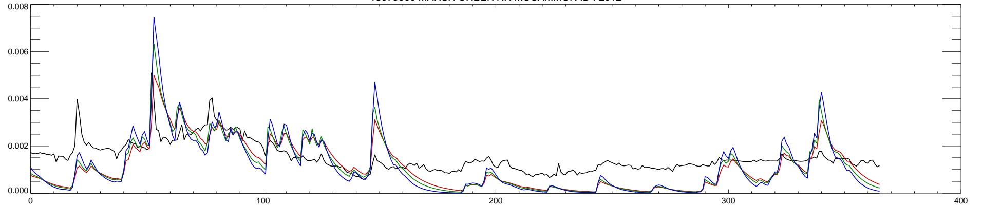
13075000 MARSH CREEK NR MCCAMMON ID : 2013
