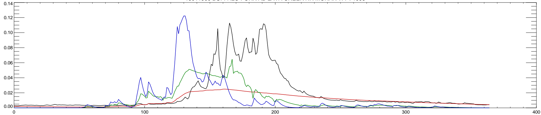
13011900 BUFFALO FORK AB LAVA CREEK NR MORAN WY : 1995
