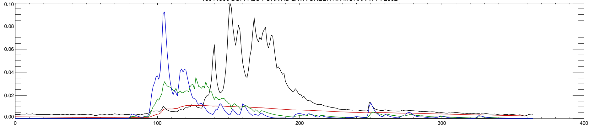
13011900 BUFFALO FORK AB LAVA CREEK NR MORAN WY : 2003
