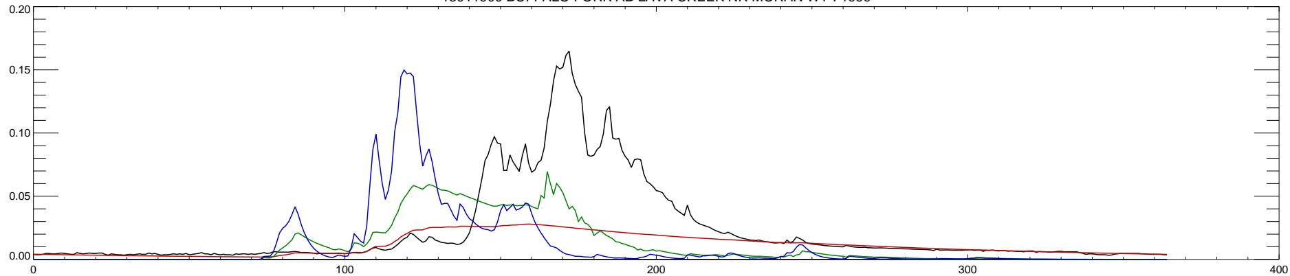
13011900 BUFFALO FORK AB LAVA CREEK NR MORAN WY : 2000
