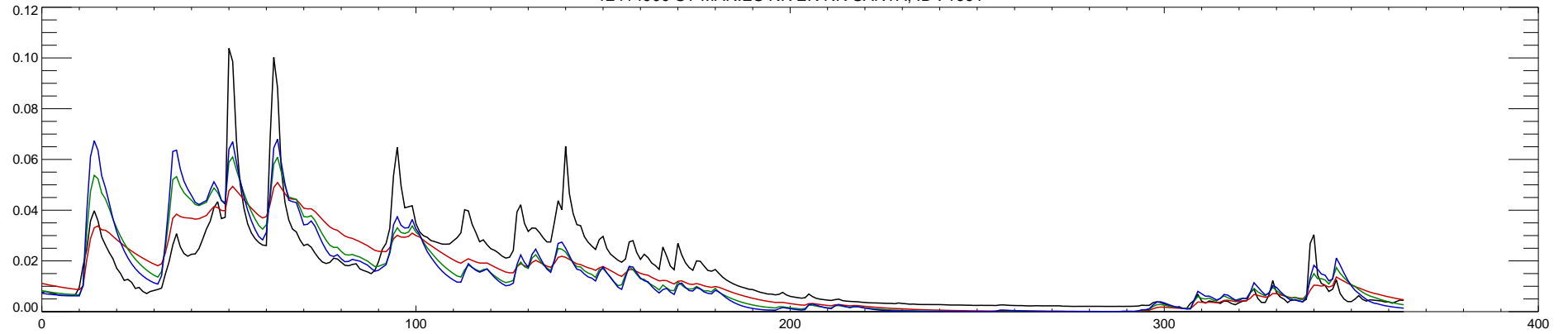
12414900 ST MARIES RIVER NR SANTA, ID : 1992
