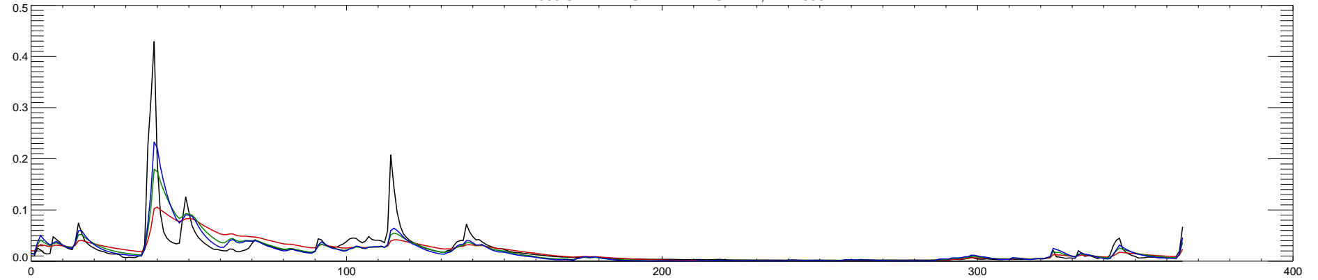
12414900 ST MARIES RIVER NR SANTA, ID : 1997
