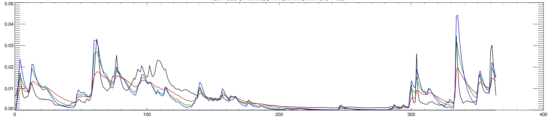
12414900 ST MARIES RIVER NR SANTA, ID : 1995
