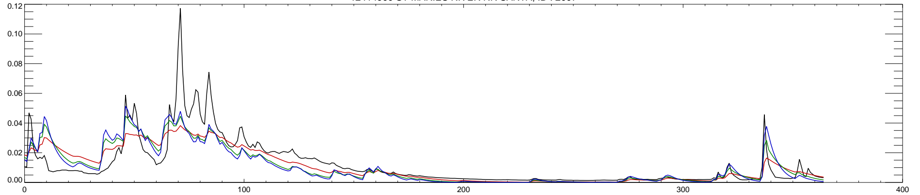
12414900 ST MARIES RIVER NR SANTA, ID : 2007
