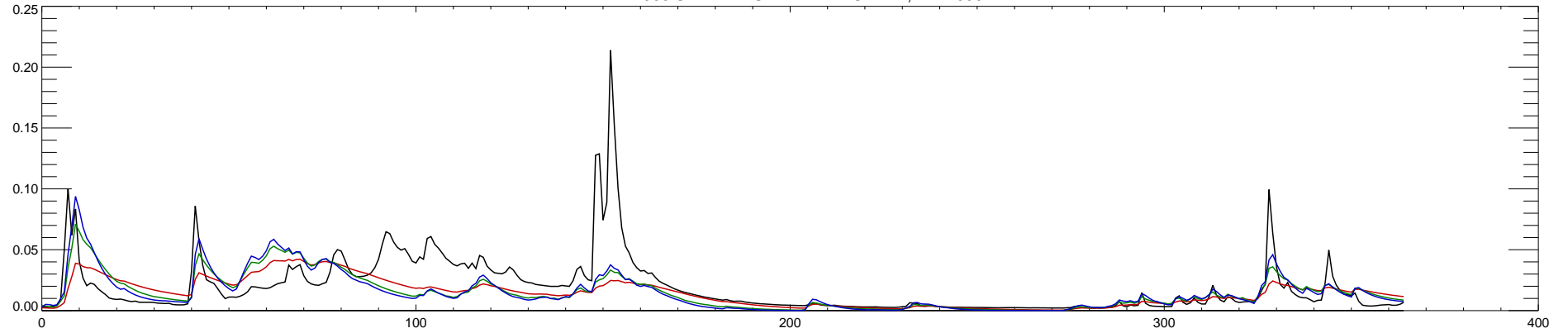
12414900 ST MARIES RIVER NR SANTA, ID : 1991
