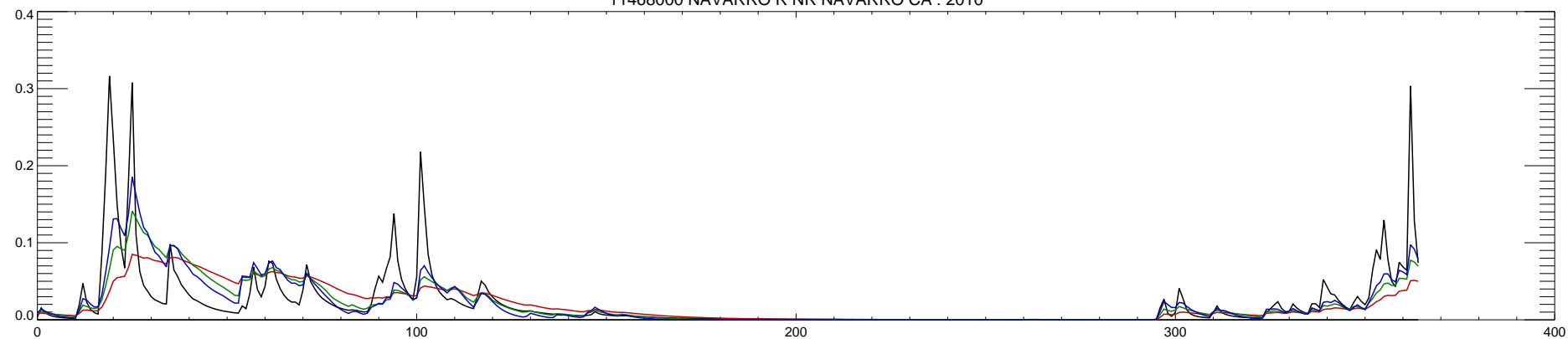
11468000 NAVARRO R NR NAVARRO CA : 2010
