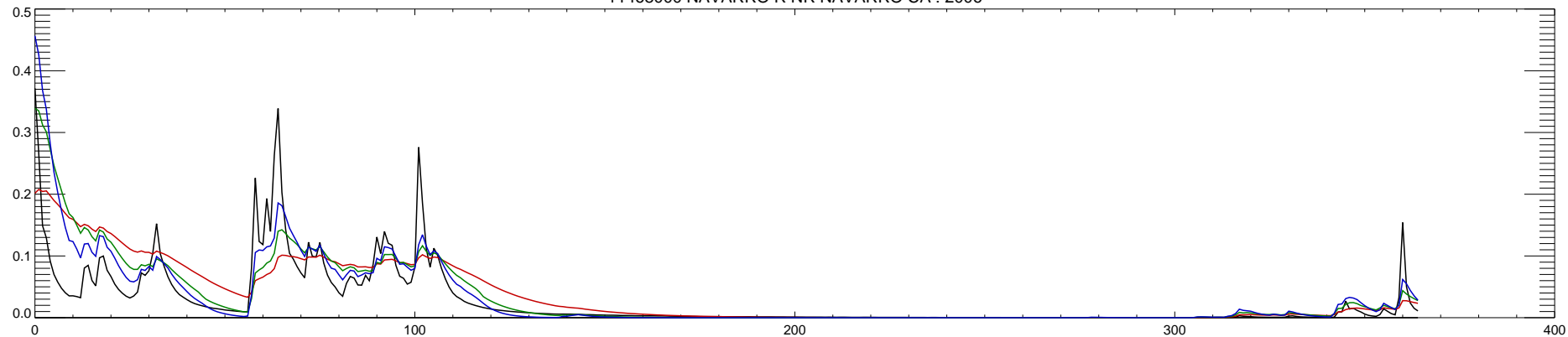
11468000 NAVARRO R NR NAVARRO CA : 2007
