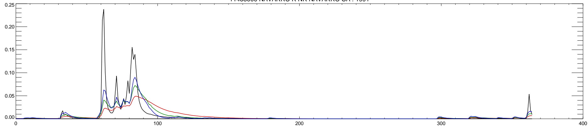
11468000 NAVARRO R NR NAVARRO CA : 1992
