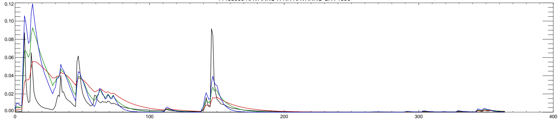
11468000 NAVARRO R NR NAVARRO CA : 1991
