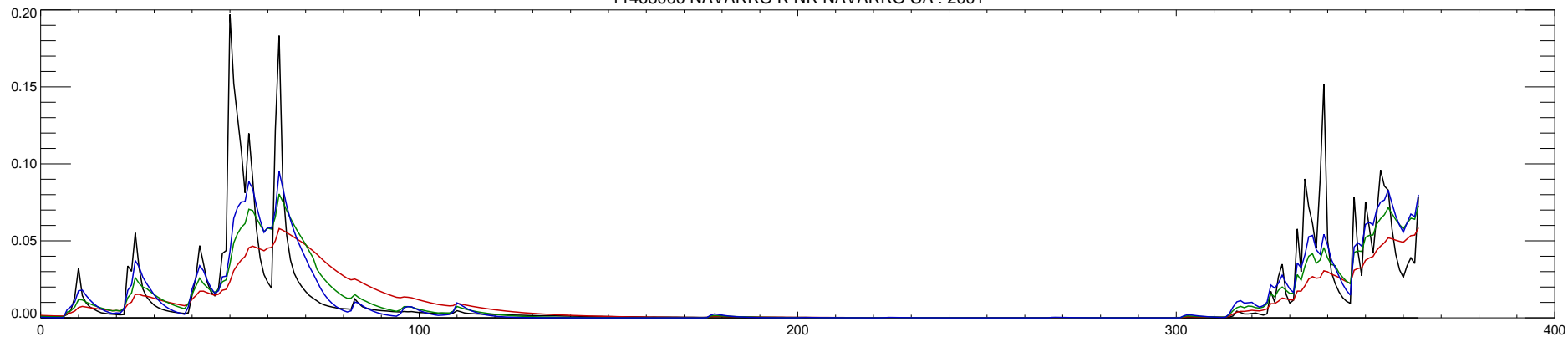
11468000 NAVARRO R NR NAVARRO CA : 2001
