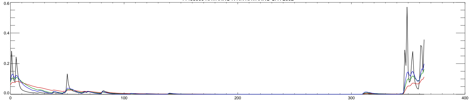
11468000 NAVARRO R NR NAVARRO CA : 2003
