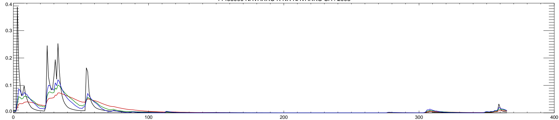
11468000 NAVARRO R NR NAVARRO CA : 2009
