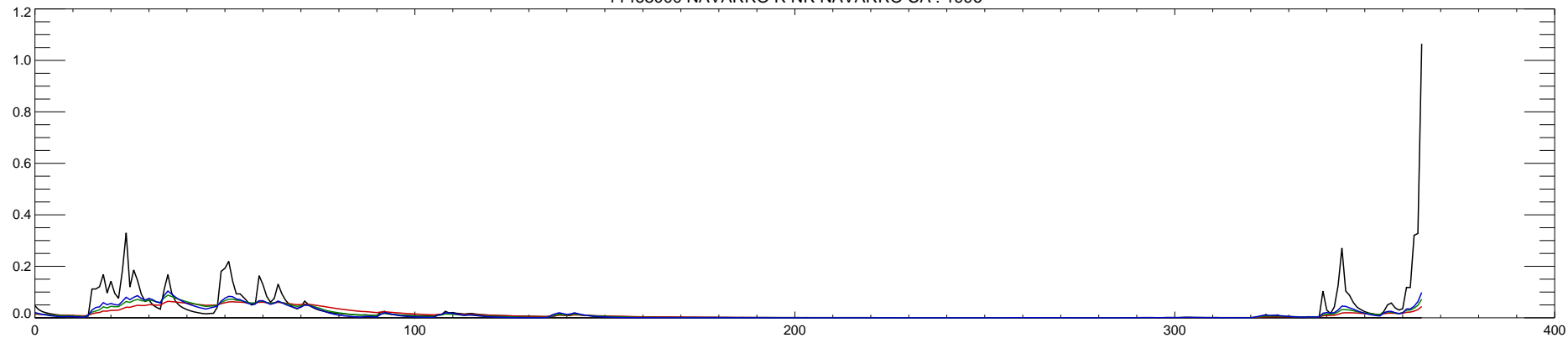
11468000 NAVARRO R NR NAVARRO CA : 1997
