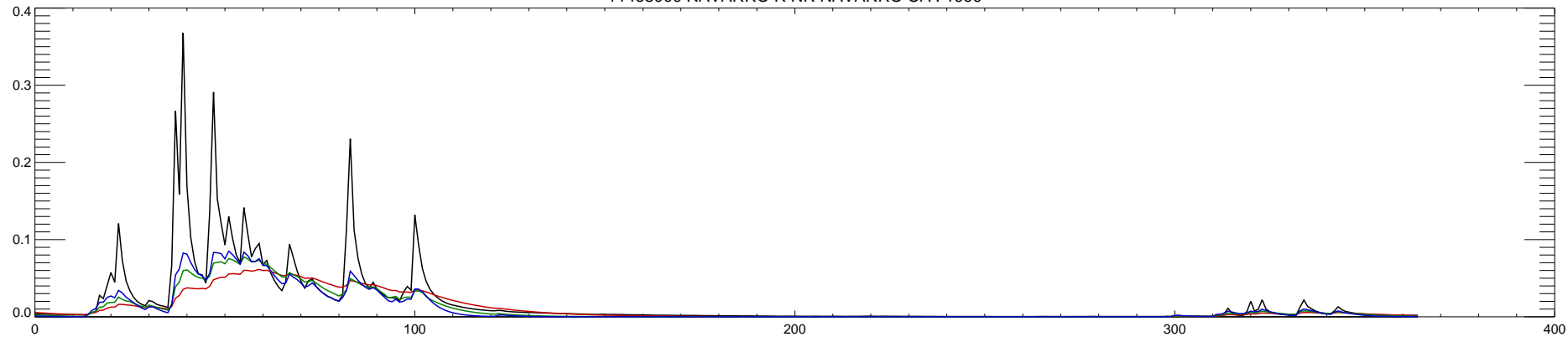
11468000 NAVARRO R NR NAVARRO CA : 2000
