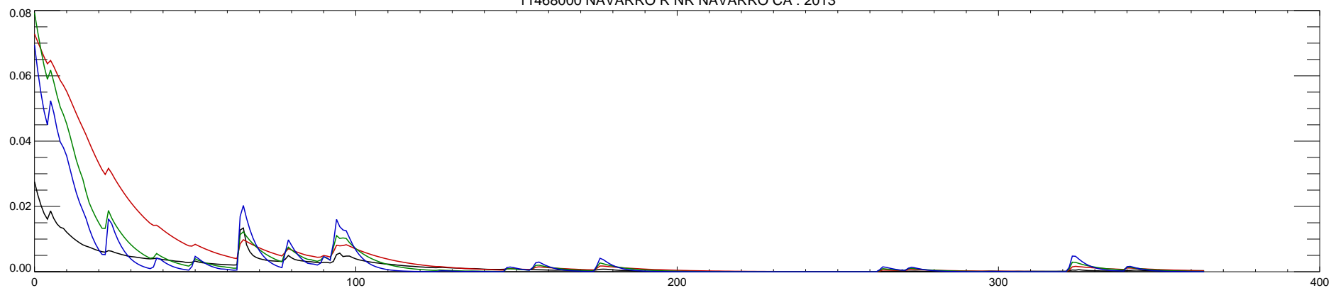
11468000 NAVARRO R NR NAVARRO CA : 2013
