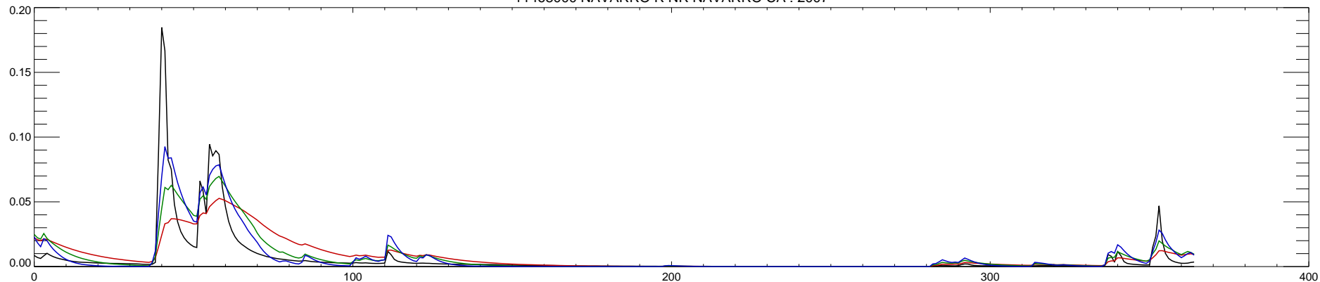
11468000 NAVARRO R NR NAVARRO CA : 2007
