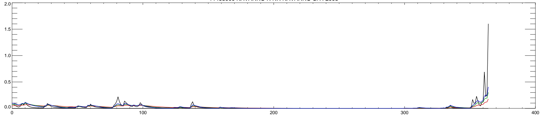
11468000 NAVARRO R NR NAVARRO CA : 2006
