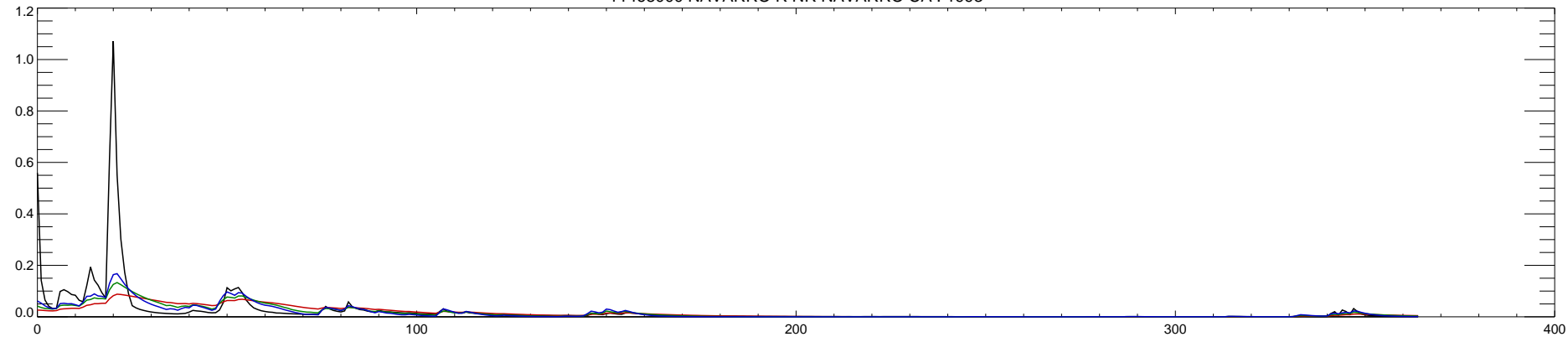
11468000 NAVARRO R NR NAVARRO CA : 1994
