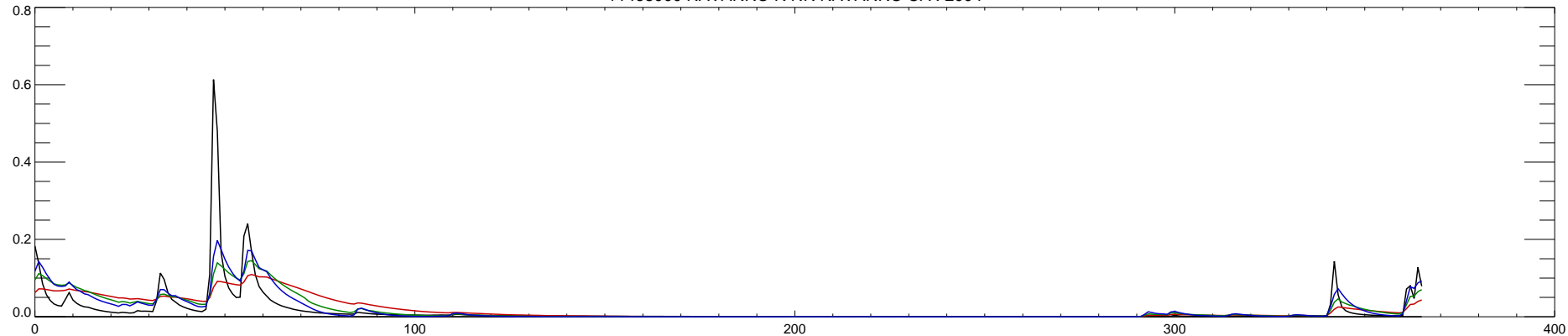
11468000 NAVARRO R NR NAVARRO CA : 2004
