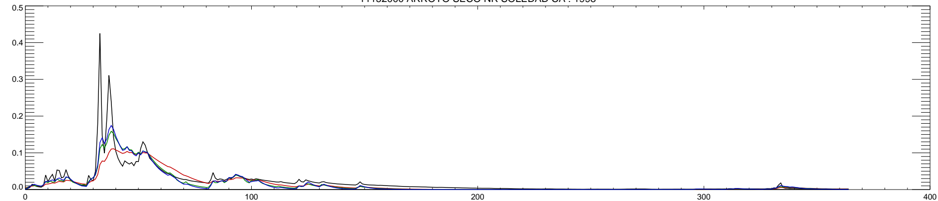
11152000 ARROYO SECO NR SOLEDAD CA : 1998
