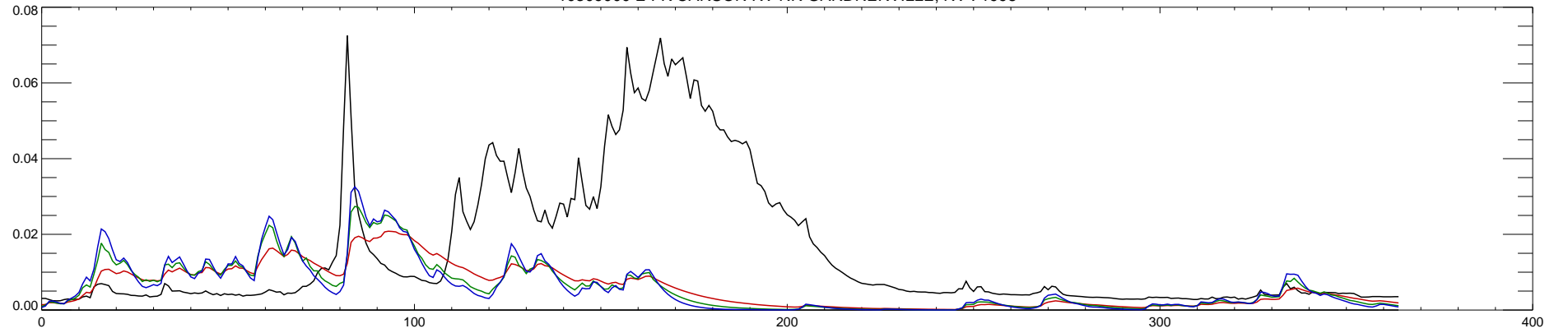
10309000 E FK CARSON RV NR GARDNERVILLE, NV : 1998
