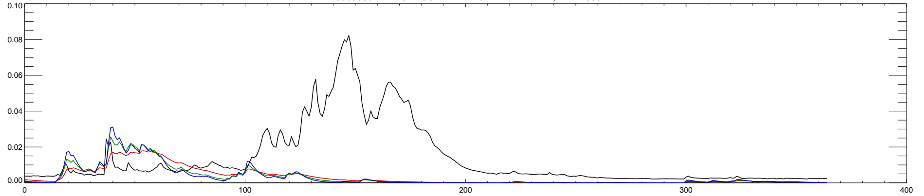
10309000 E FK CARSON RV NR GARDNERVILLE, NV : 2000
