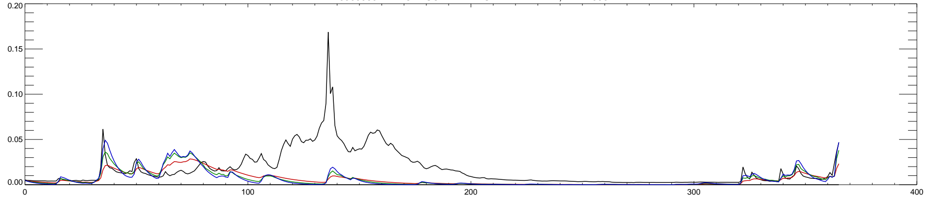
10309000 E FK CARSON RV NR GARDNERVILLE, NV : 1997
