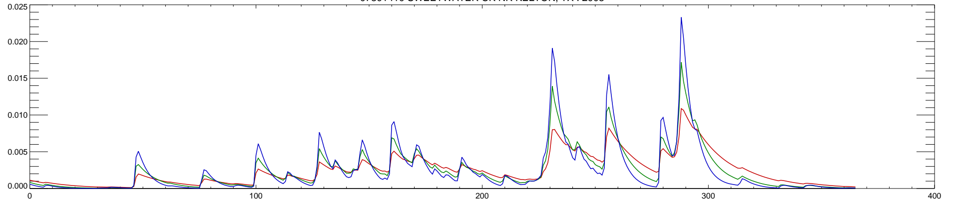
07301410 SWEETWATER CK NR KELTON, TX : 2009
