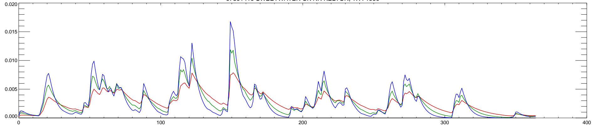
07301410 SWEETWATER CK NR KELTON, TX : 1991
