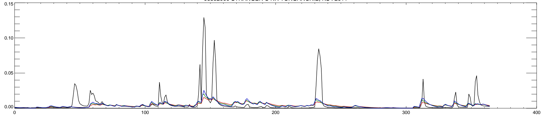
06892000 STRANGER C NR TONGANOXIE, KS : 2012
