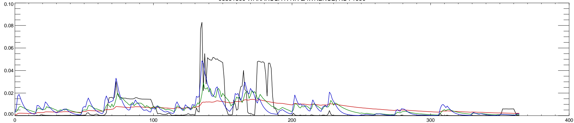
06891500 WAKARUSA R NR LAWRENCE, KS : 1991
