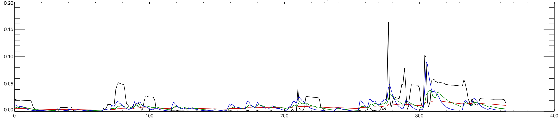
06891500 WAKARUSA R NR LAWRENCE, KS : 1998
