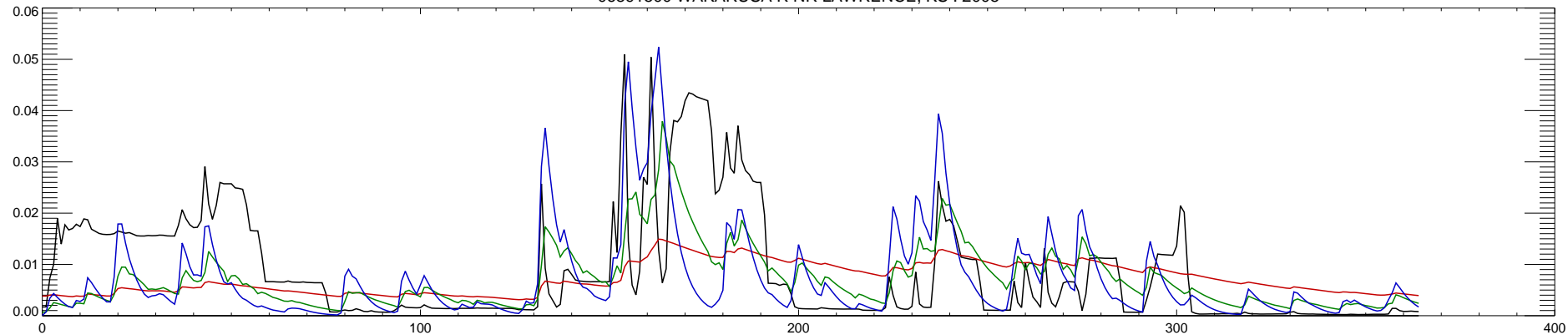
06891500 WAKARUSA R NR LAWRENCE, KS : 2006
