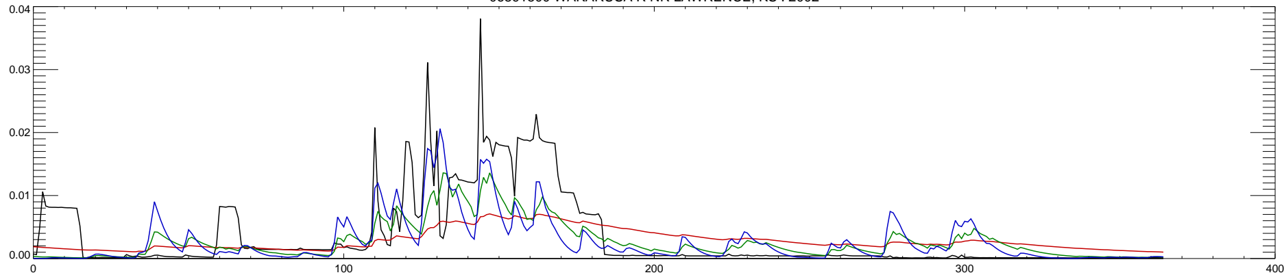
06891500 WAKARUSA R NR LAWRENCE, KS : 2003
