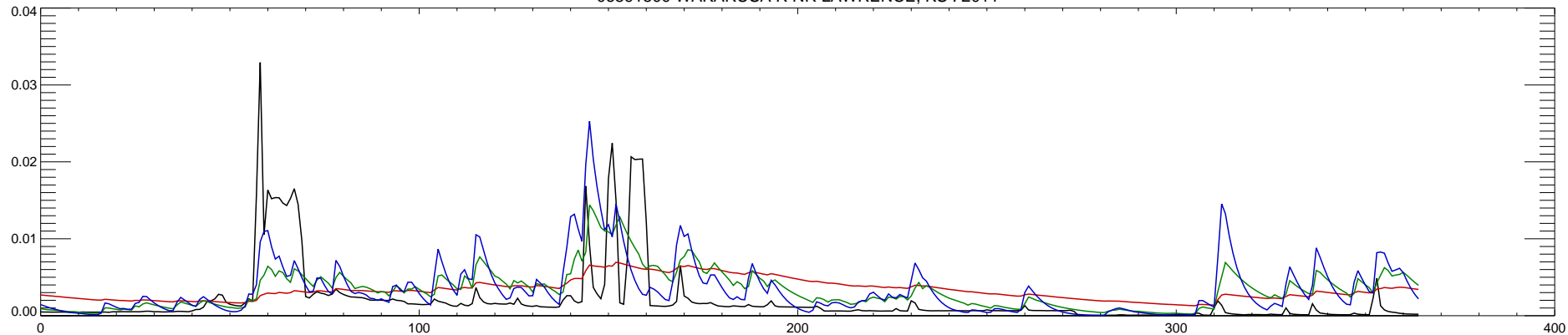
06891500 WAKARUSA R NR LAWRENCE, KS : 2012
