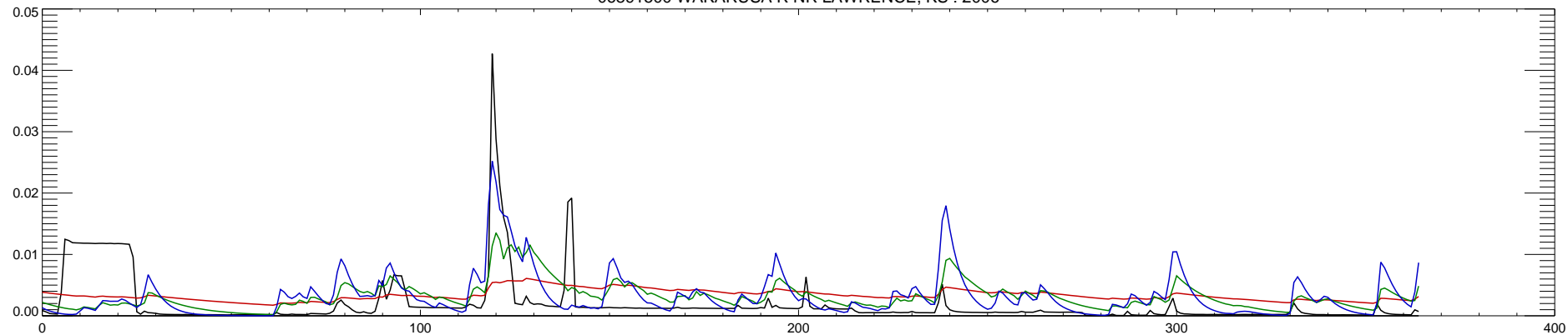
06891500 WAKARUSA R NR LAWRENCE, KS : 2007
