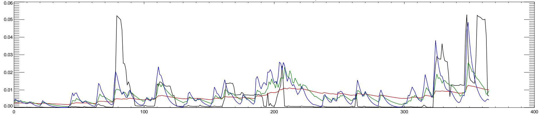
06891500 WAKARUSA R NR LAWRENCE, KS : 1992
