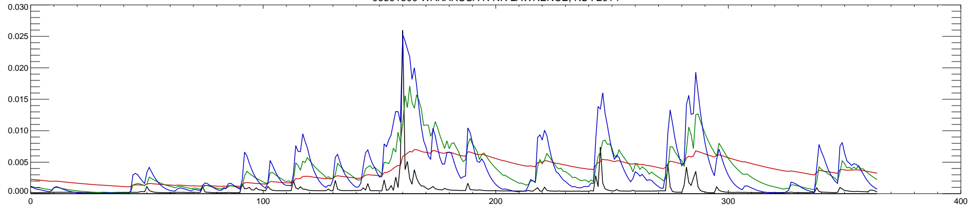
06891500 WAKARUSA R NR LAWRENCE, KS : 2015
