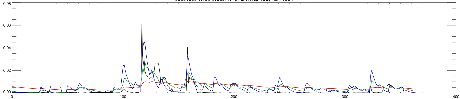
06891500 WAKARUSA R NR LAWRENCE, KS : 1995
