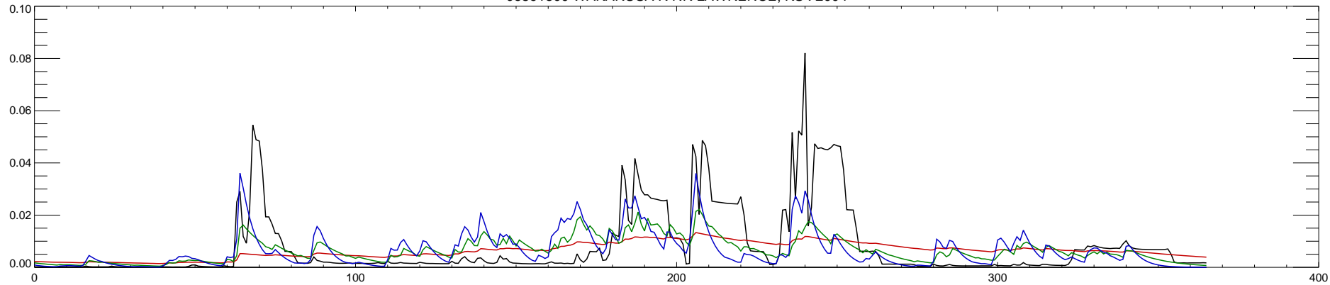
06891500 WAKARUSA R NR LAWRENCE, KS : 2004
