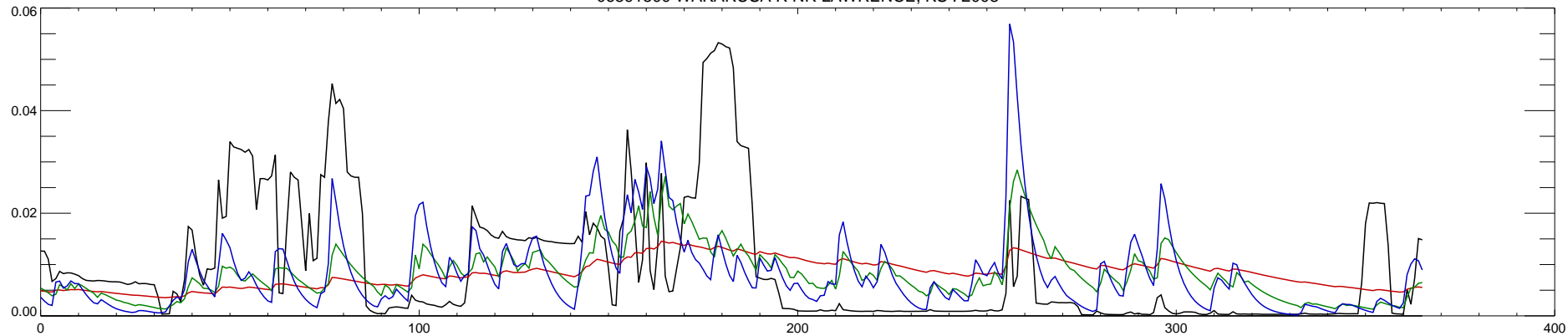
06891500 WAKARUSA R NR LAWRENCE, KS : 2009
