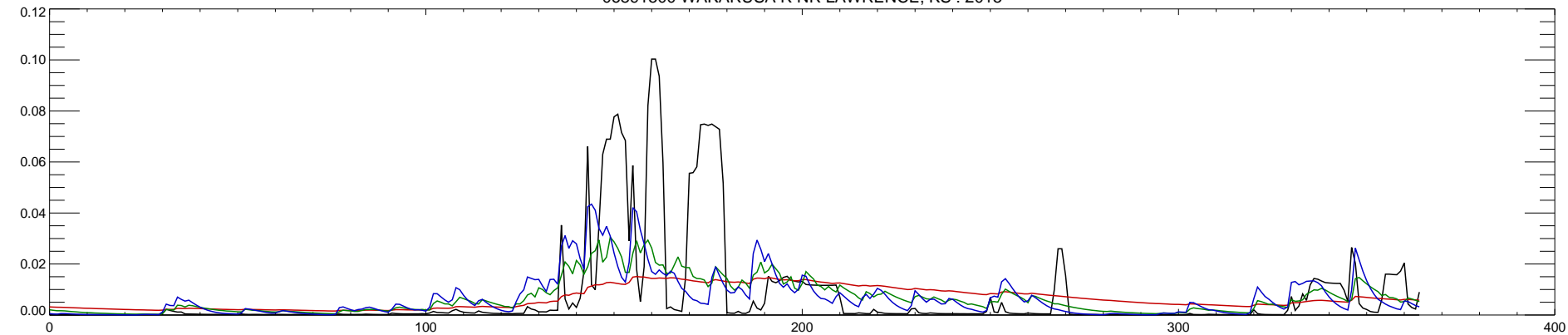
06891500 WAKARUSA R NR LAWRENCE, KS : 2016
