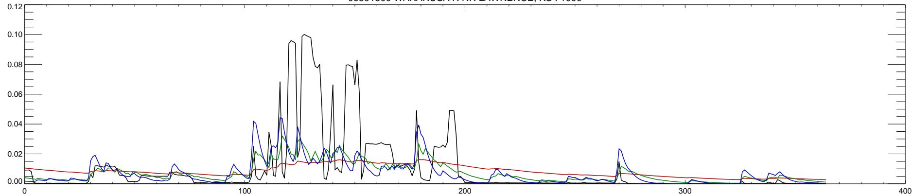
06891500 WAKARUSA R NR LAWRENCE, KS : 2000
