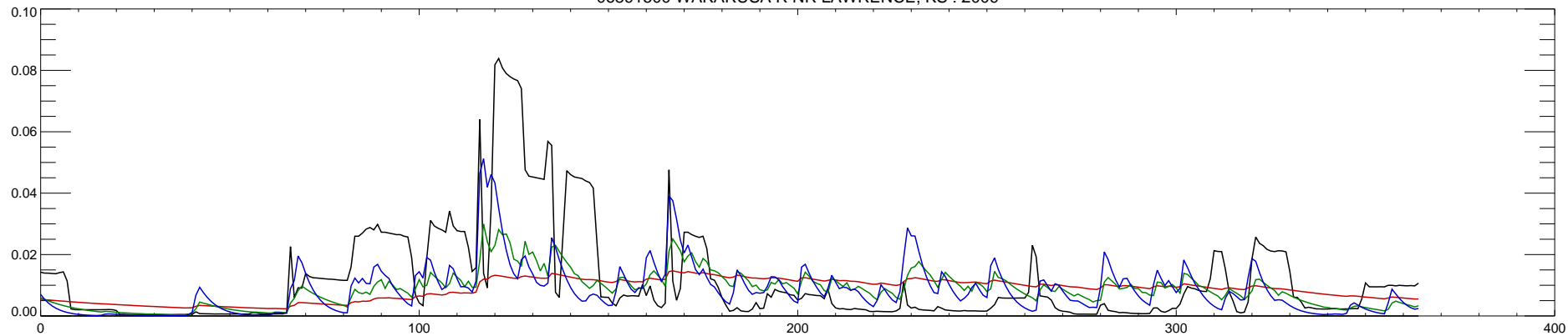
06891500 WAKARUSA R NR LAWRENCE, KS : 2010
