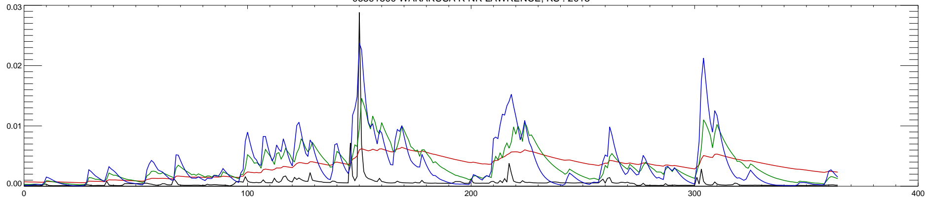
06891500 WAKARUSA R NR LAWRENCE, KS : 2013
