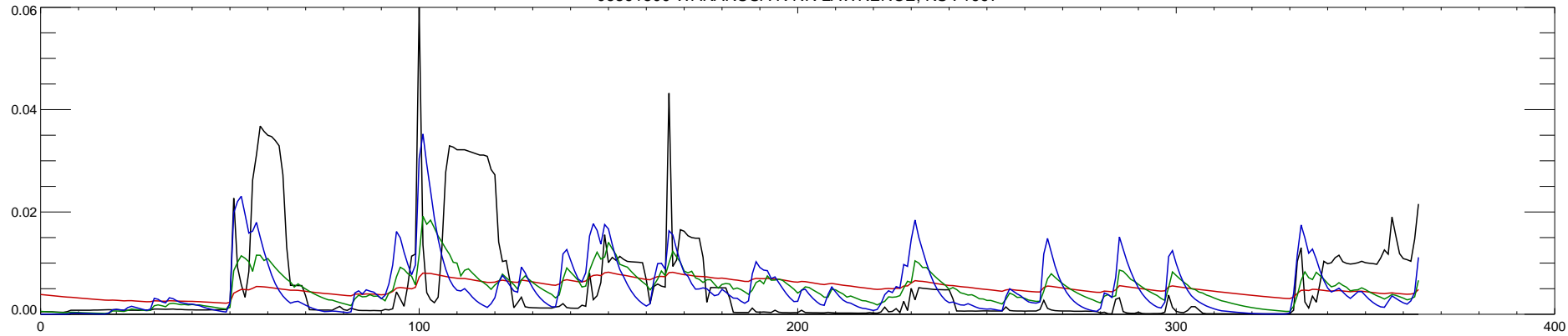
06891500 WAKARUSA R NR LAWRENCE, KS : 1998
