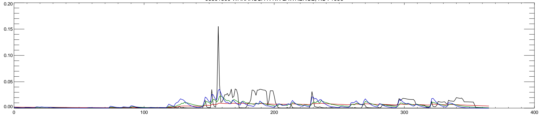
06891500 WAKARUSA R NR LAWRENCE, KS : 1997
