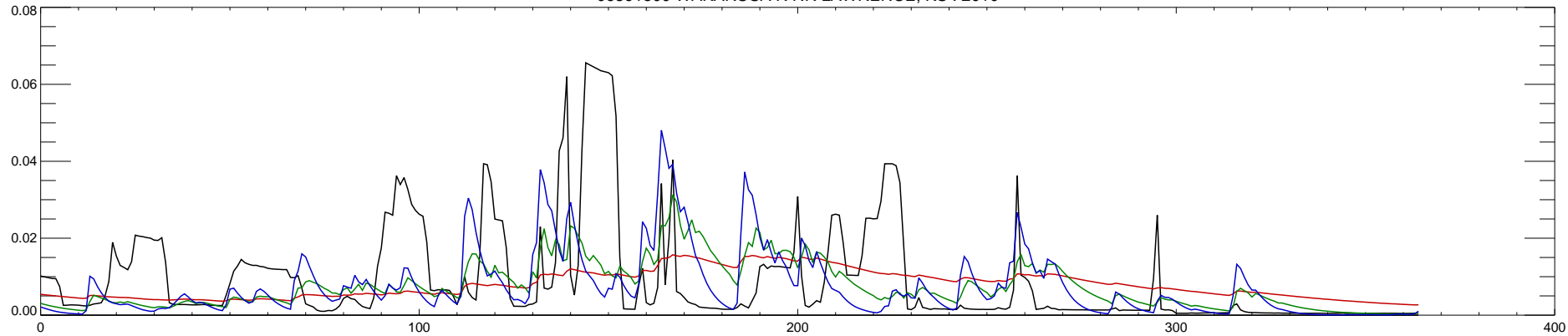
06891500 WAKARUSA R NR LAWRENCE, KS : 2010
