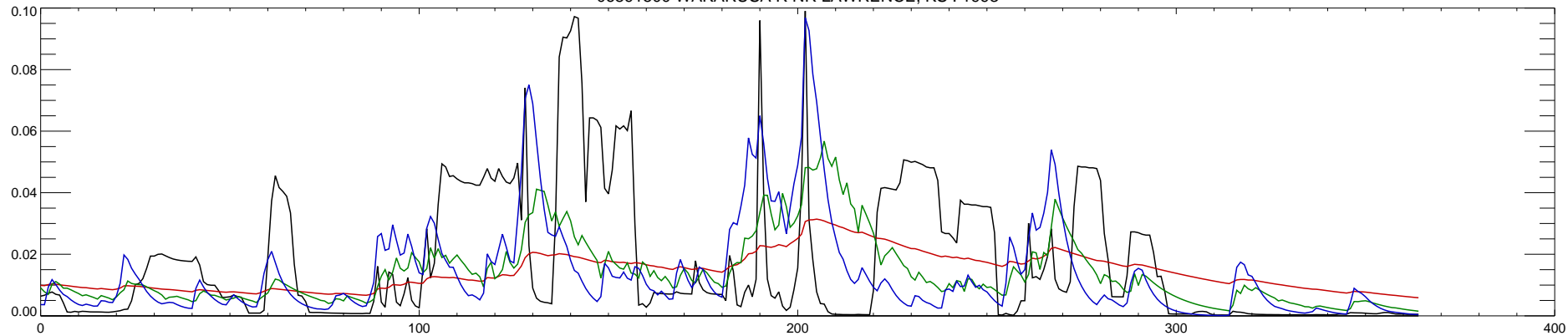
06891500 WAKARUSA R NR LAWRENCE, KS : 1994
