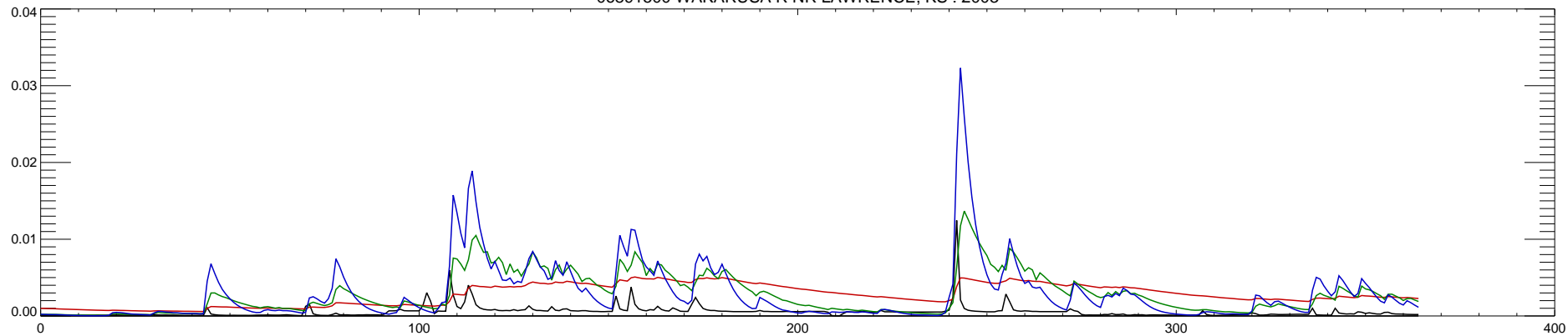
06891500 WAKARUSA R NR LAWRENCE, KS : 2004
