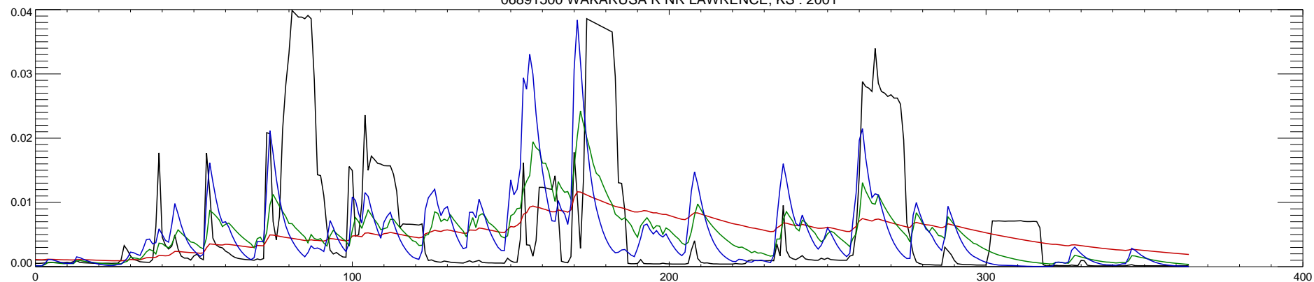
06891500 WAKARUSA R NR LAWRENCE, KS : 2001
