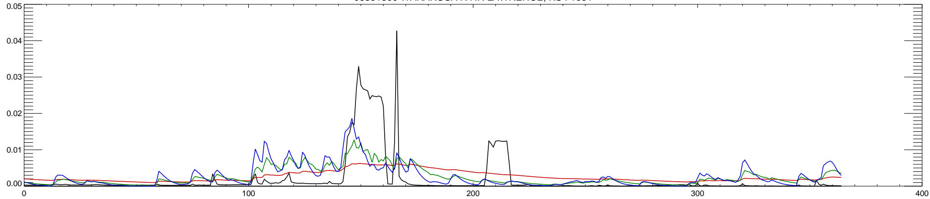
06891500 WAKARUSA R NR LAWRENCE, KS : 1992
