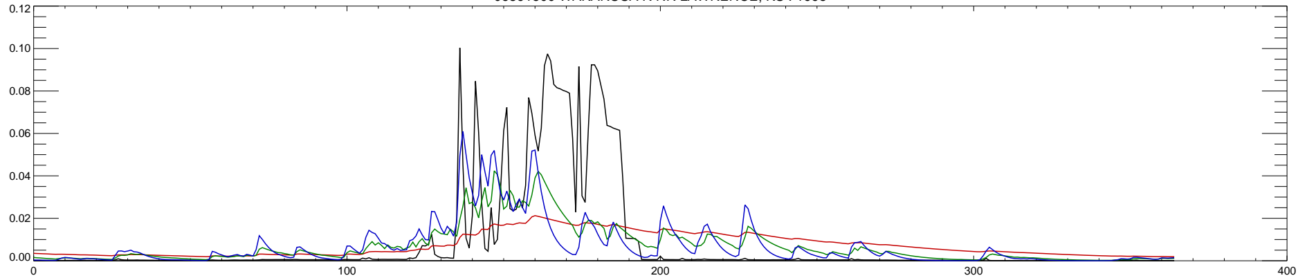
06891500 WAKARUSA R NR LAWRENCE, KS : 1995
