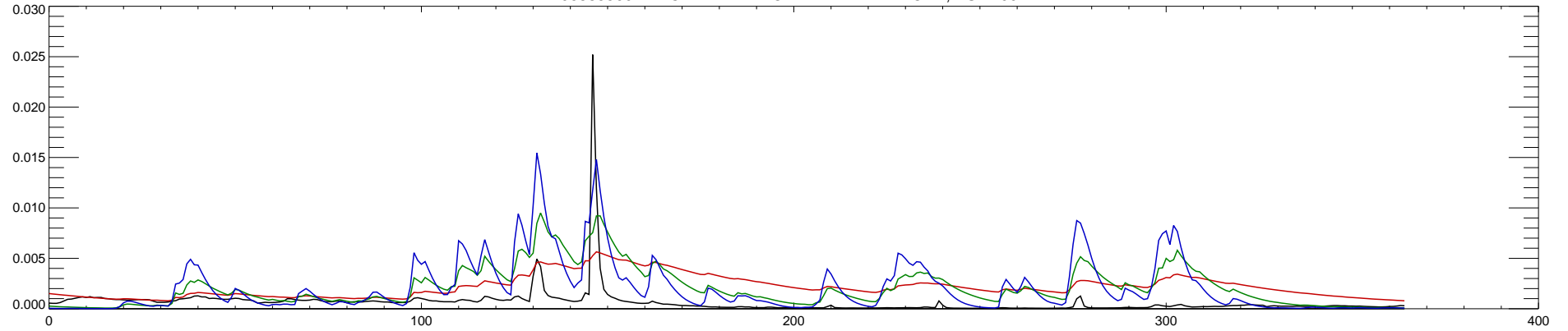
06885500 BLACK VERMILLION R NR FRANKFORT, KS : 2003
