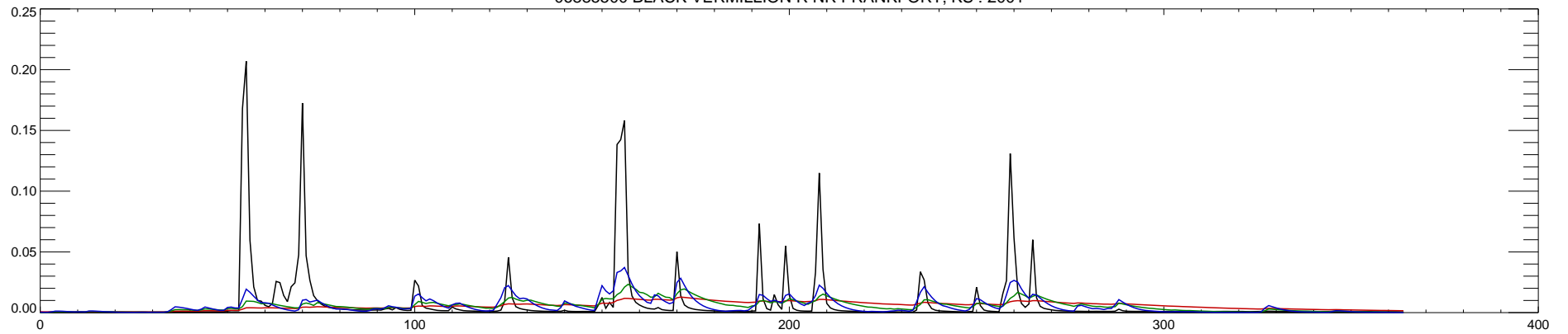
06885500 BLACK VERMILLION R NR FRANKFORT, KS : 2001
