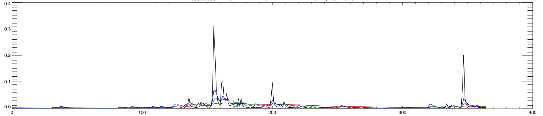
06885500 BLACK VERMILLION R NR FRANKFORT, KS : 2016
