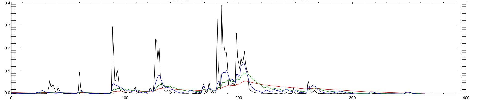
06885500 BLACK VERMILLION R NR FRANKFORT, KS : 1994
