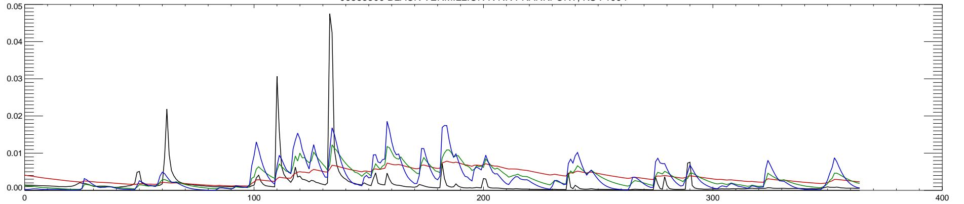
06885500 BLACK VERMILLION R NR FRANKFORT, KS : 1995
