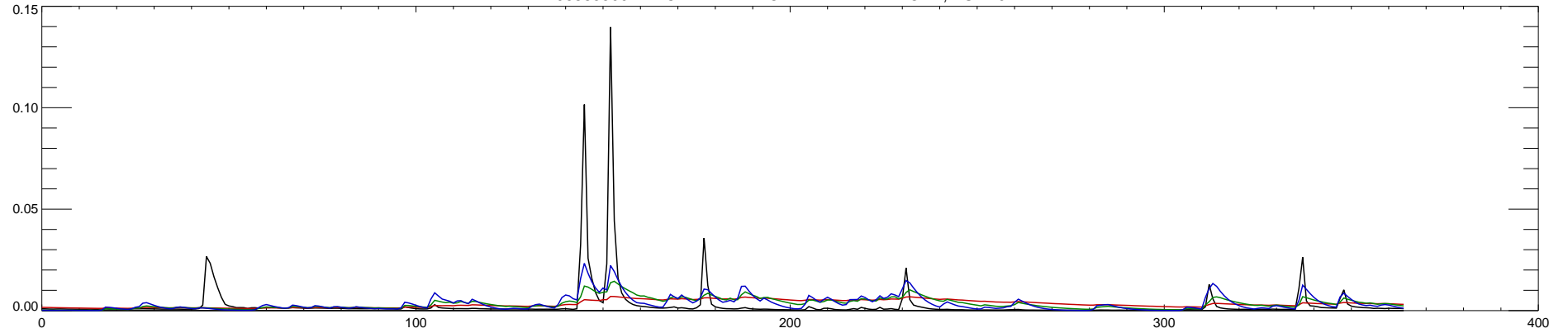
06885500 BLACK VERMILLION R NR FRANKFORT, KS : 2012
