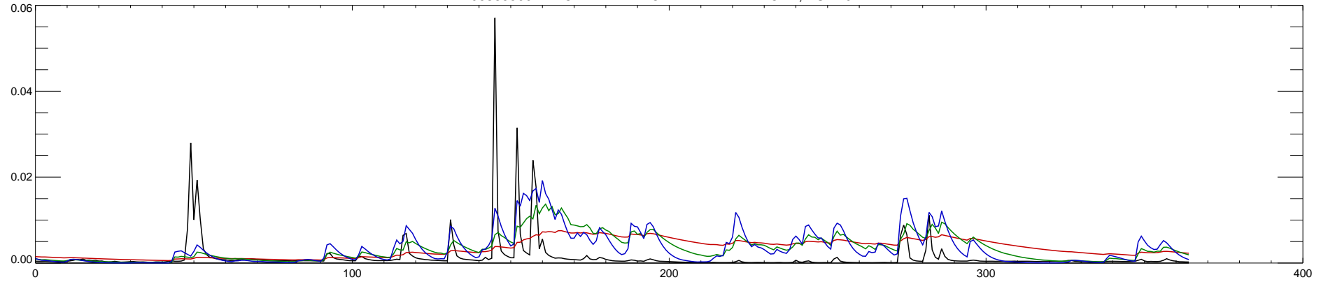
06885500 BLACK VERMILLION R NR FRANKFORT, KS : 2015
