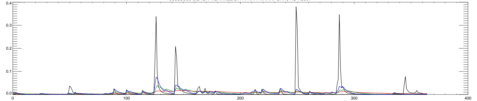
06885500 BLACK VERMILLION R NR FRANKFORT, KS : 2007
