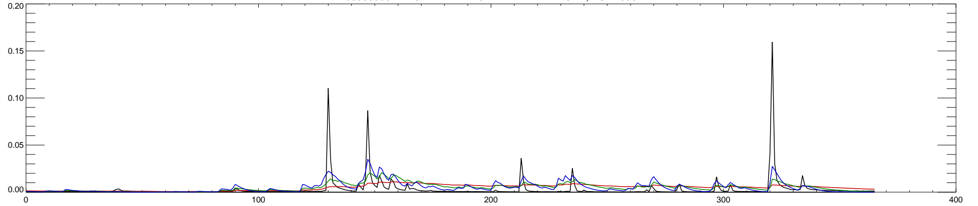
06885500 BLACK VERMILLION R NR FRANKFORT, KS : 1997
