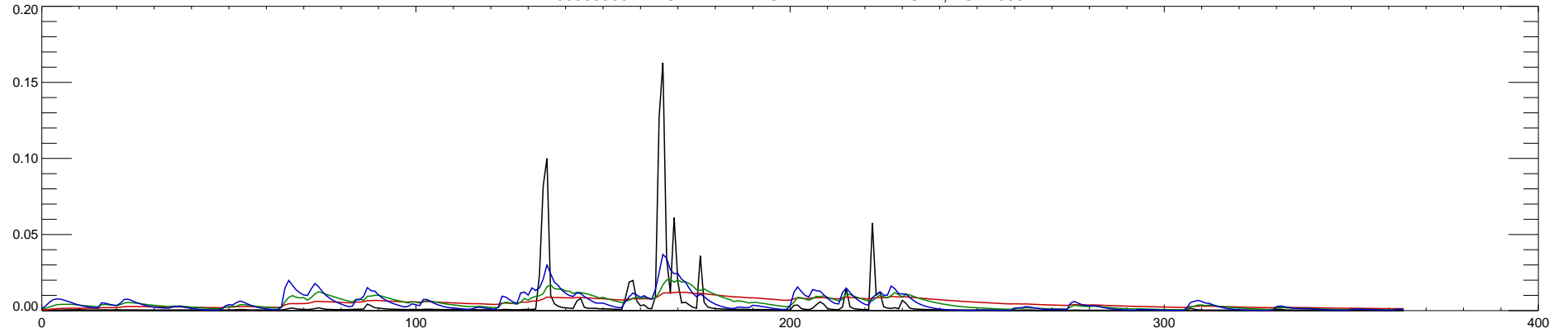
06885500 BLACK VERMILLION R NR FRANKFORT, KS : 1991
