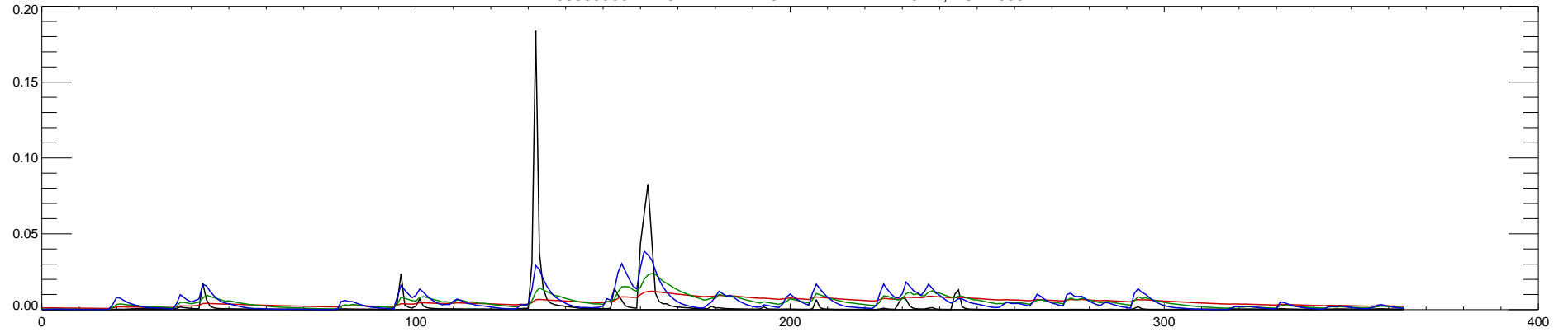
06885500 BLACK VERMILLION R NR FRANKFORT, KS : 2006
