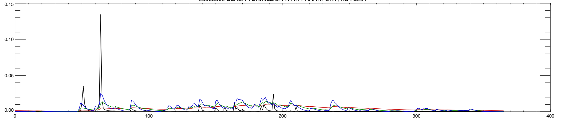
06885500 BLACK VERMILLION R NR FRANKFORT, KS : 2004
