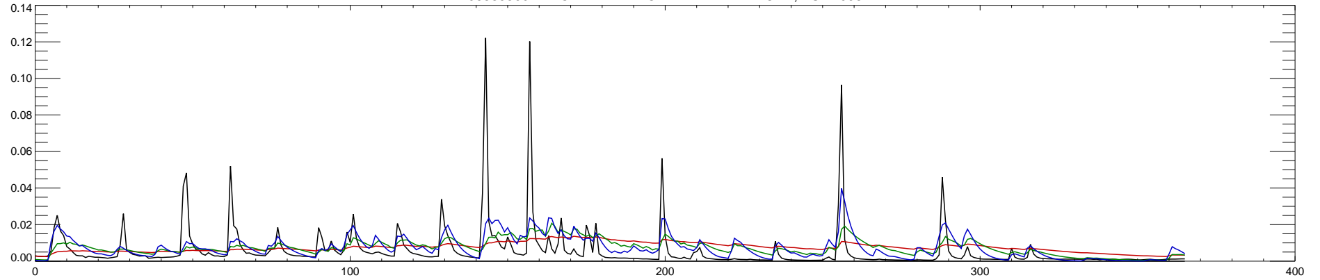
06885500 BLACK VERMILLION R NR FRANKFORT, KS : 2009
