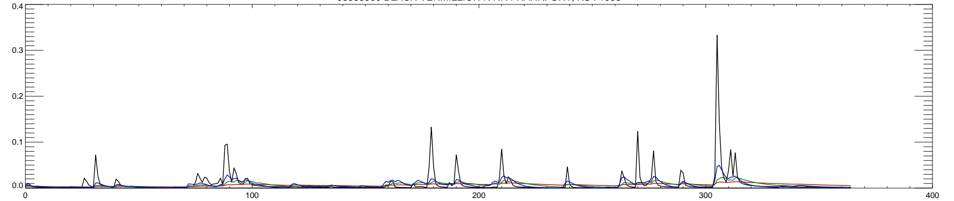
06885500 BLACK VERMILLION R NR FRANKFORT, KS : 1998
