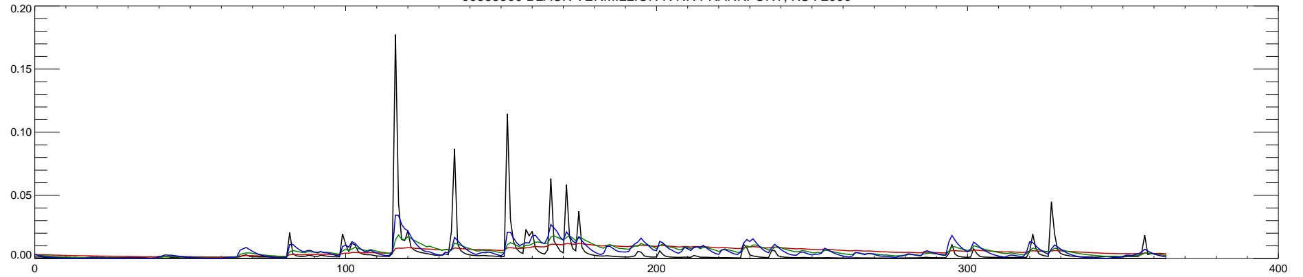
06885500 BLACK VERMILLION R NR FRANKFORT, KS : 2010
