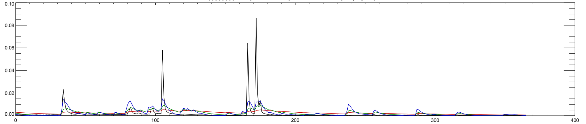
06885500 BLACK VERMILLION R NR FRANKFORT, KS : 2013
