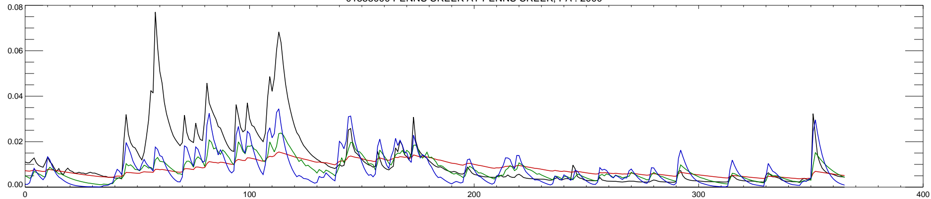
01555000 PENNS CREEK AT PENNS CREEK, PA : 2001
