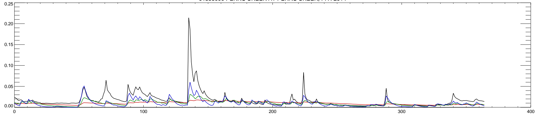
01555000 PENNS CREEK AT PENNS CREEK, PA : 2015
