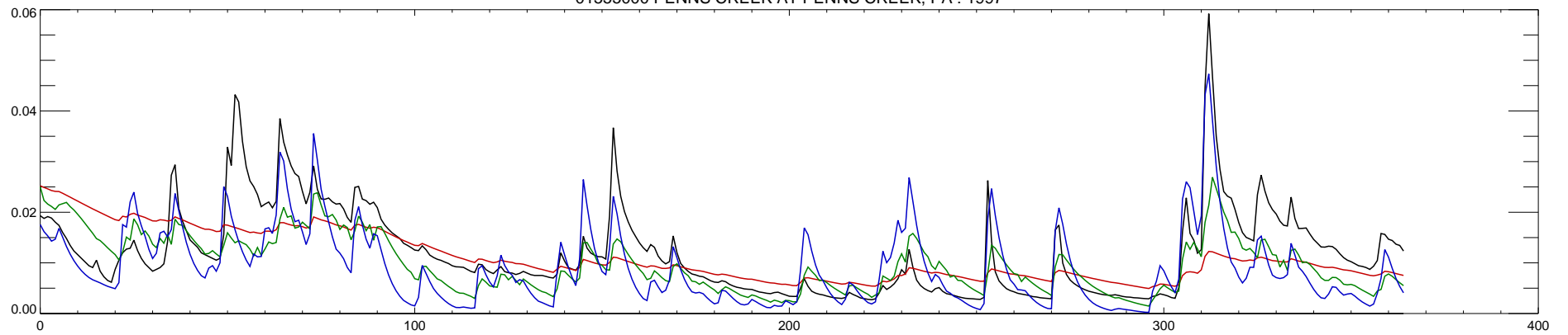
01555000 PENNS CREEK AT PENNS CREEK, PA : 1998
