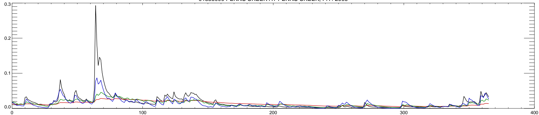
01555000 PENNS CREEK AT PENNS CREEK, PA : 2009
