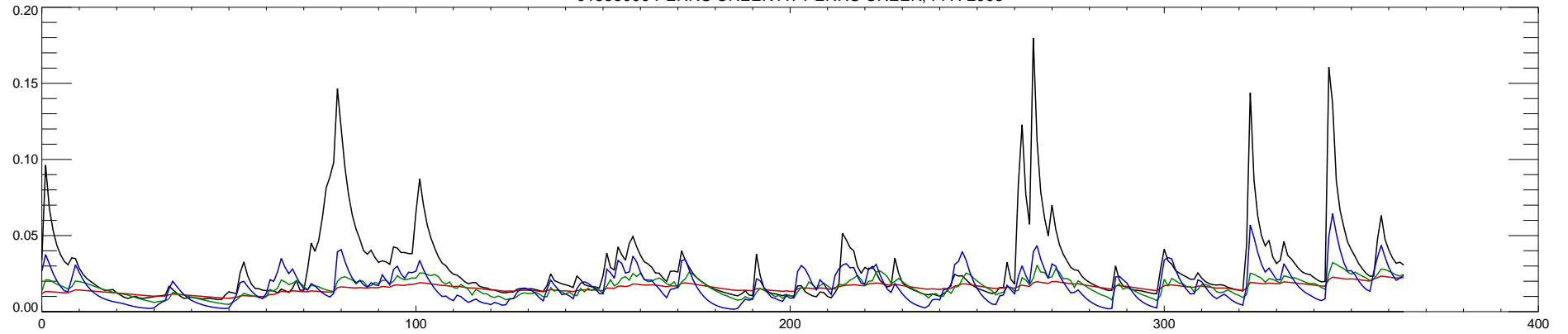
01555000 PENNS CREEK AT PENNS CREEK, PA : 2004
