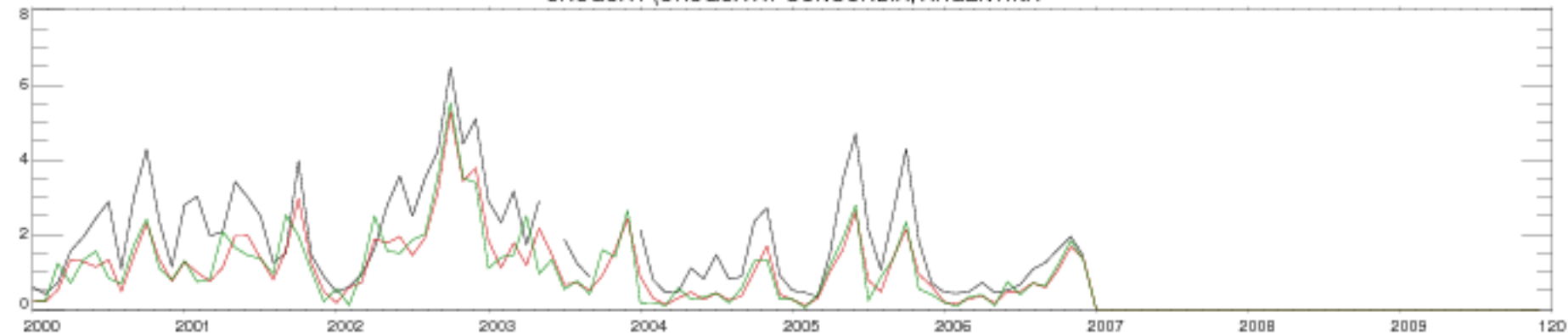
URUGUAY (URUGUA AT CONCORDIA, ARGENTINA)
