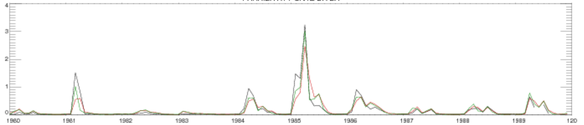
PARAIBA AT PONTE DA BA
