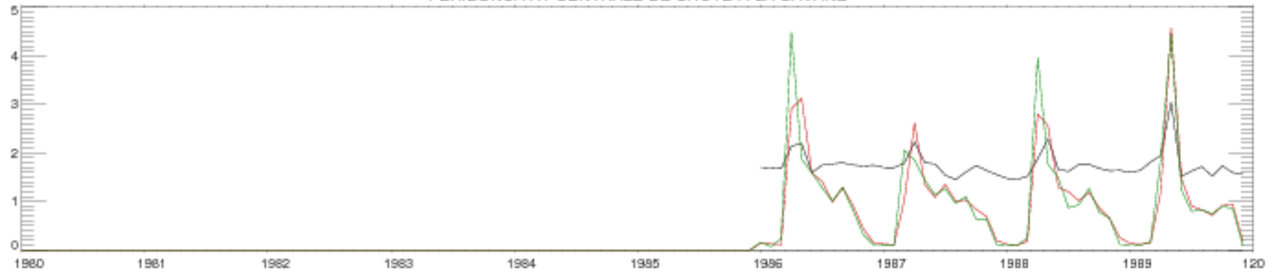
PERIBONCA AT CENTRALE DE CHUTE-A-LA-SAVANE
