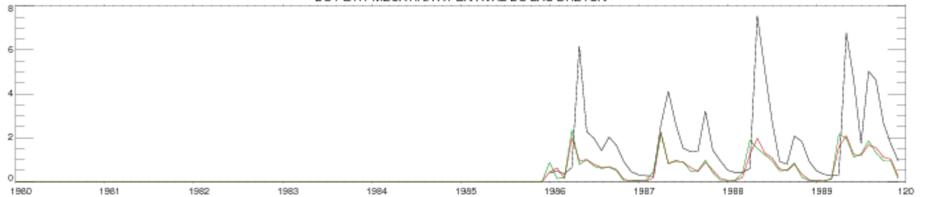
DU PETIT MECATINA AT EN AVAL DU LAC BRETON
