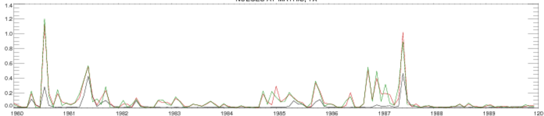
NUECES AT MATHIS, TX
