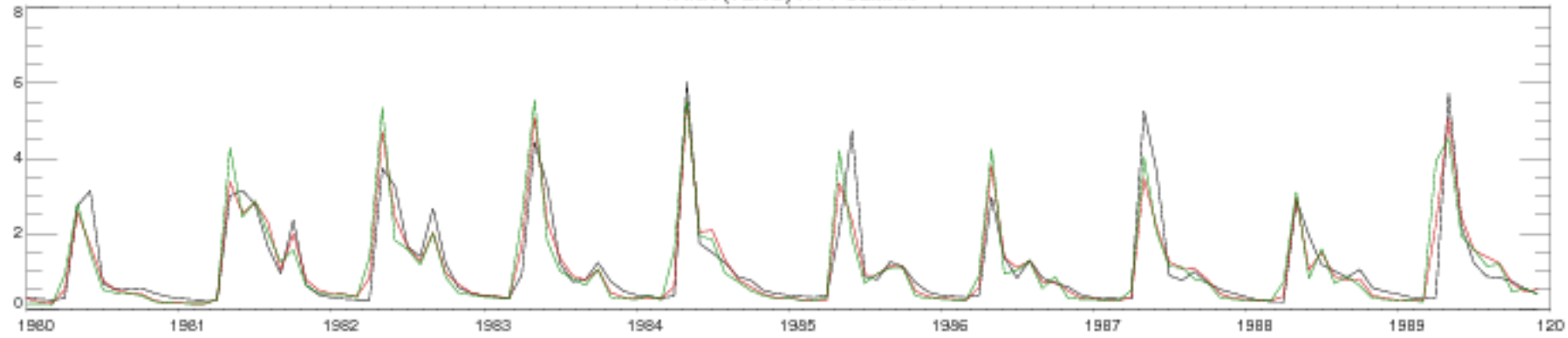
TANA (TENO) AT POLMAK
