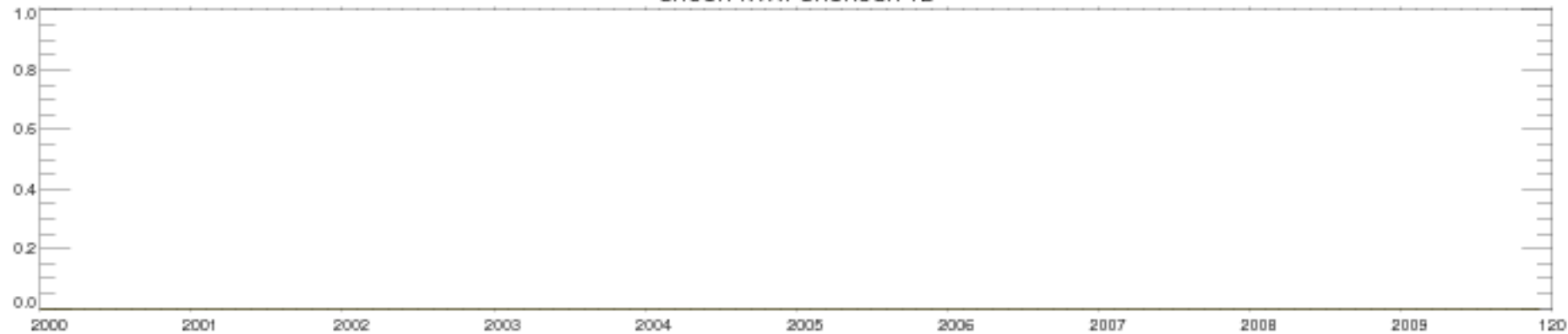
SHUCH'YA AT SHCHUCH'YE
