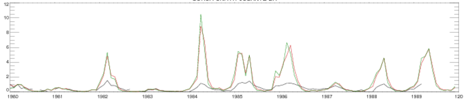
CURUA-UNA AT JUSANTE DA
