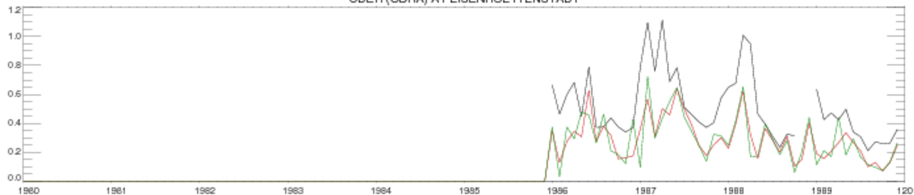
ODER (ODRA) AT EISENHUETTENSTADT
