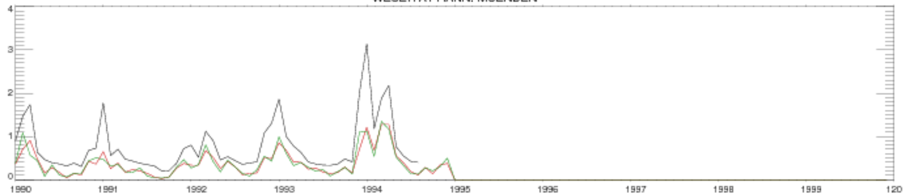
WESER AT HANN.-MUENDEN
