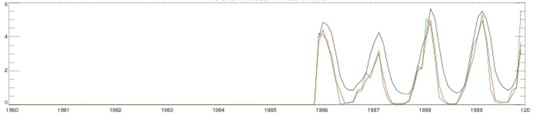
RIO SAO MANOEL AT TRES MARIAS
