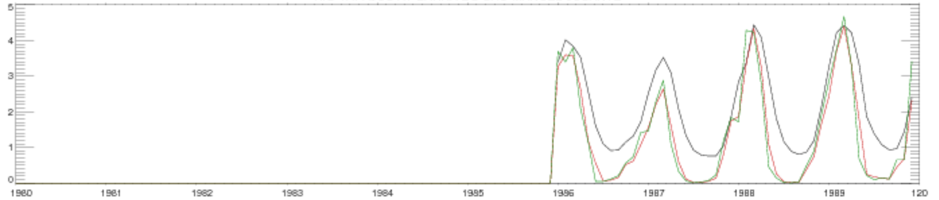
RIO TAPAJOS AT BARRA DO SAO MANUEL-JUSANTE
