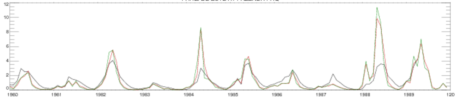
PARce DE ESTE AT FAZENDA PAQ
