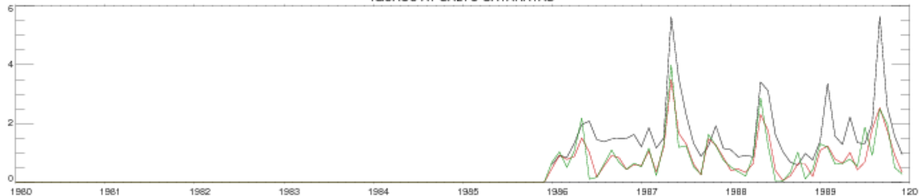
IGUACU AT SALTO CATARATAS
