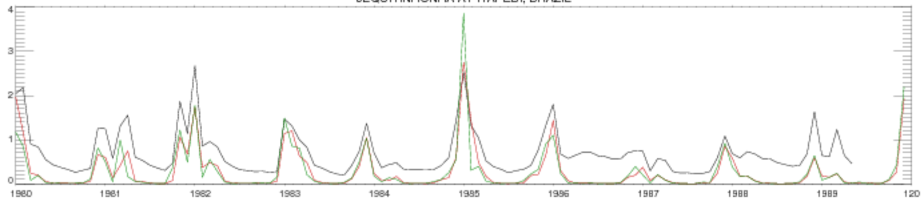
JEQUITINHONHA AT ITAPEBI, BRAZIL
