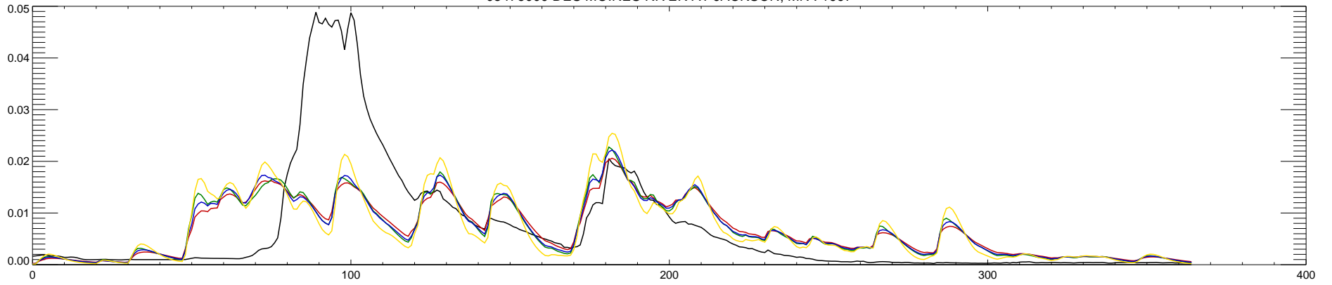
05476000 DES MOINES RIVER AT JACKSON, MN : 1998
