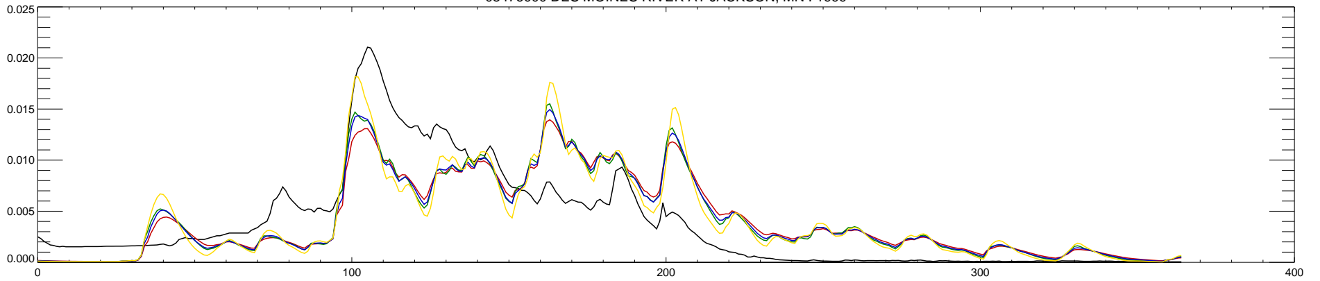
05476000 DES MOINES RIVER AT JACKSON, MN : 2000
