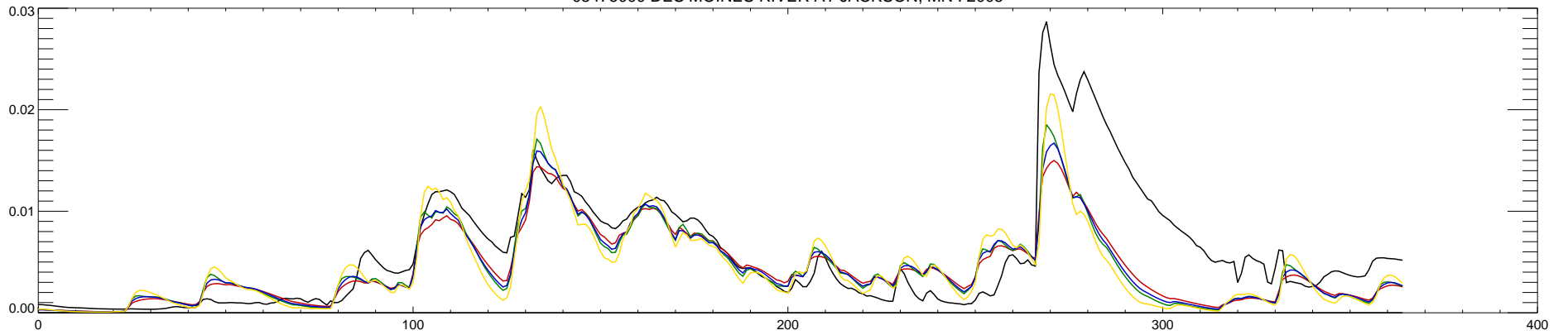
05476000 DES MOINES RIVER AT JACKSON, MN : 2006
