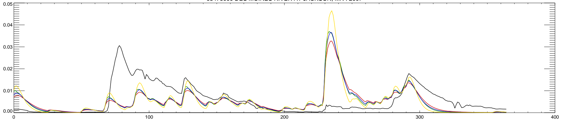
05476000 DES MOINES RIVER AT JACKSON, MN : 2007
