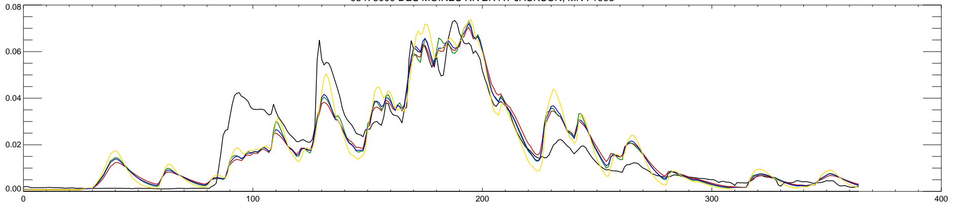
05476000 DES MOINES RIVER AT JACKSON, MN : 1994
