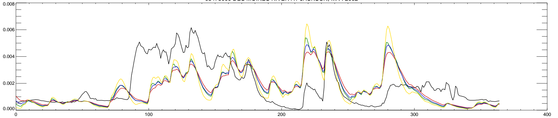
05476000 DES MOINES RIVER AT JACKSON, MN : 2003
