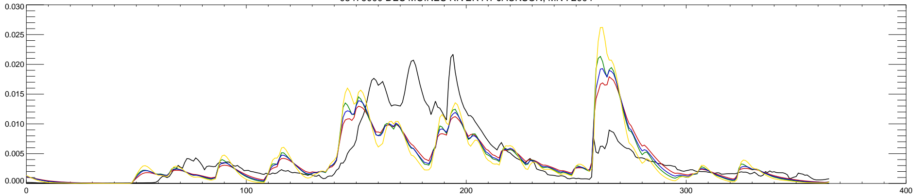
05476000 DES MOINES RIVER AT JACKSON, MN : 2004
