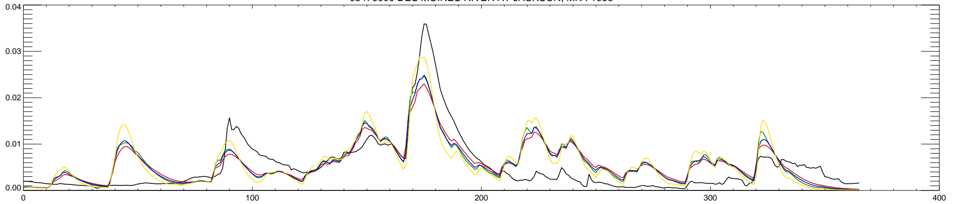
05476000 DES MOINES RIVER AT JACKSON, MN : 1997
