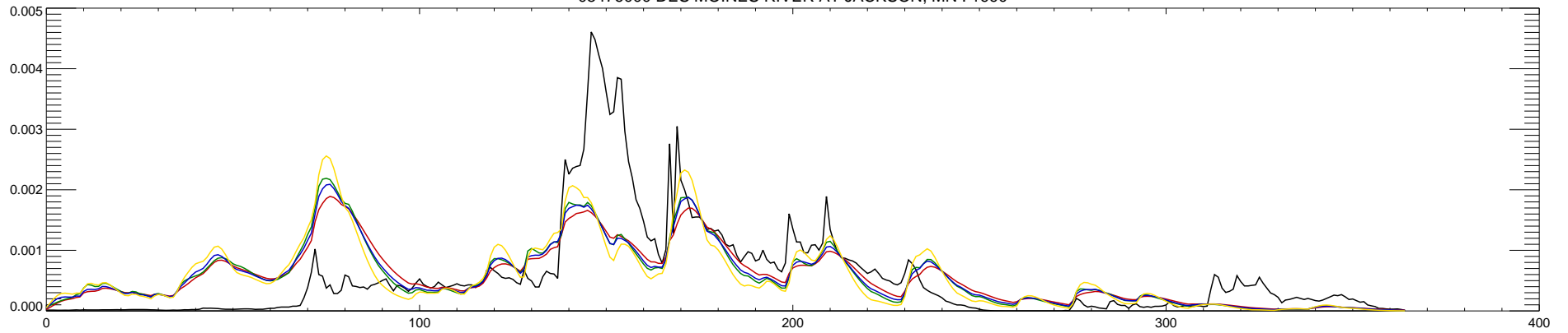
05476000 DES MOINES RIVER AT JACKSON, MN : 1991
