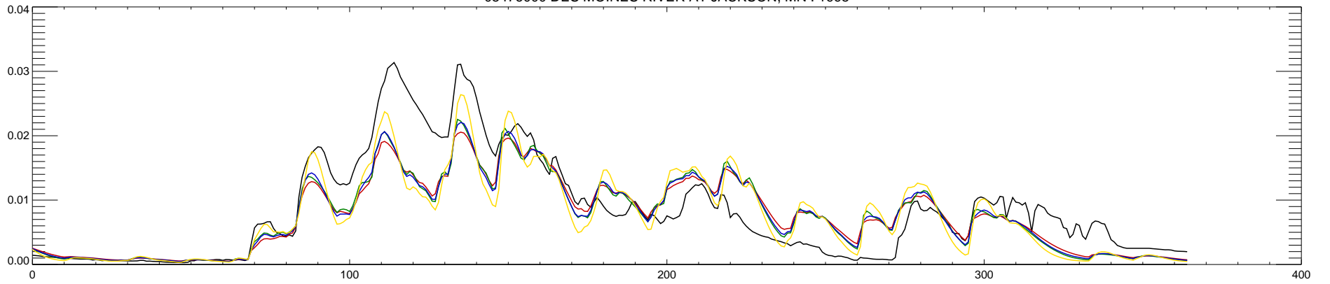
05476000 DES MOINES RIVER AT JACKSON, MN : 1995
