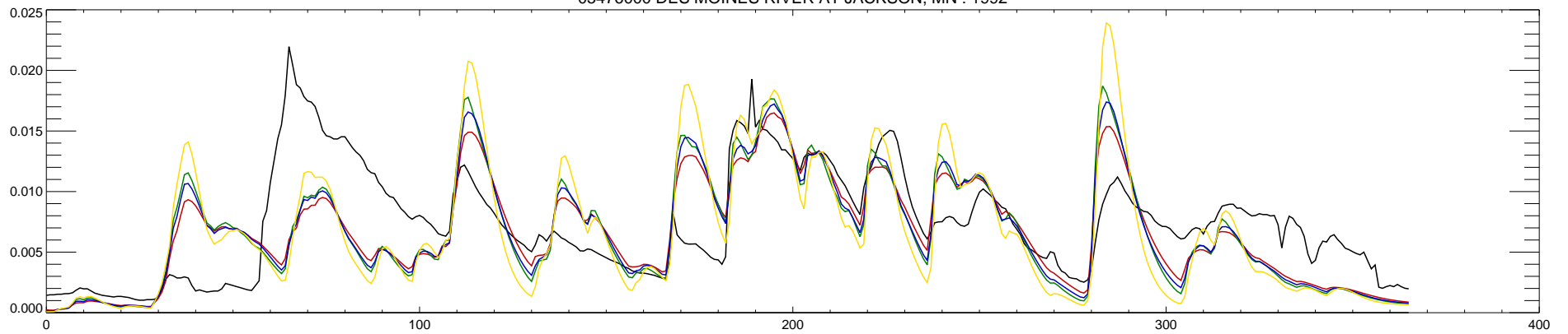
05476000 DES MOINES RIVER AT JACKSON, MN : 1992
