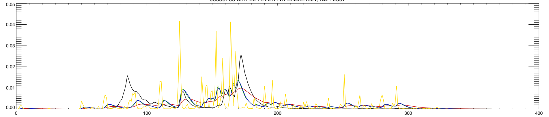
05059700 MAPLE RIVER NR ENDERLIN, ND : 2007
