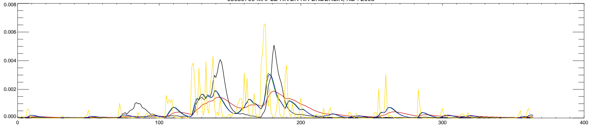
05059700 MAPLE RIVER NR ENDERLIN, ND : 2004
