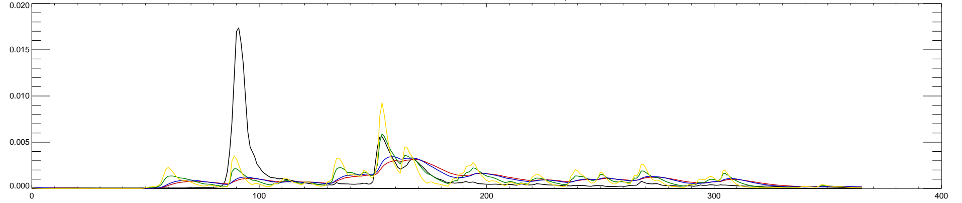
05056000 SHEYENNE RIVER NR WARWICK, ND : 2004
