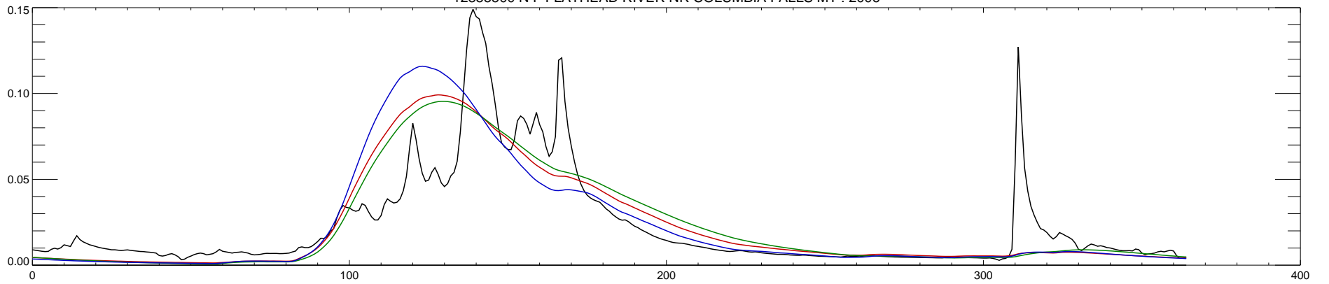
12355500 N F FLATHEAD RIVER NR COLUMBIA FALLS MT : 2007
