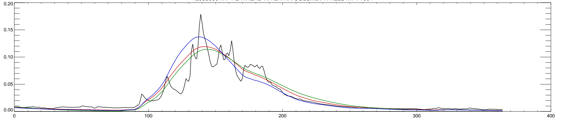
12355500 N F FLATHEAD RIVER NR COLUMBIA FALLS MT : 1992
