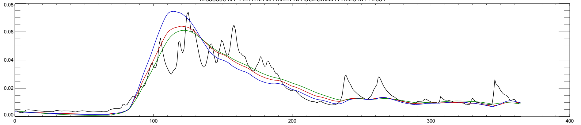
12355500 N F FLATHEAD RIVER NR COLUMBIA FALLS MT : 2004
