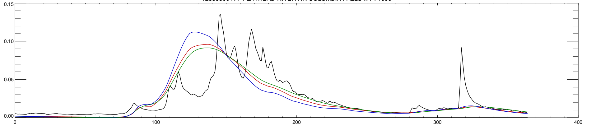
12355500 N F FLATHEAD RIVER NR COLUMBIA FALLS MT : 2000
