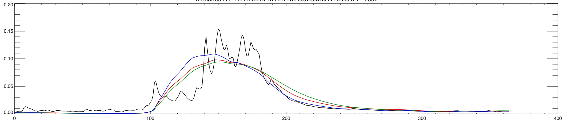
12355500 N F FLATHEAD RIVER NR COLUMBIA FALLS MT : 2003
