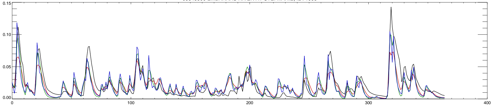
03345500 EMBARRAS RIVER AT STE. MARIE, IL : 1994
