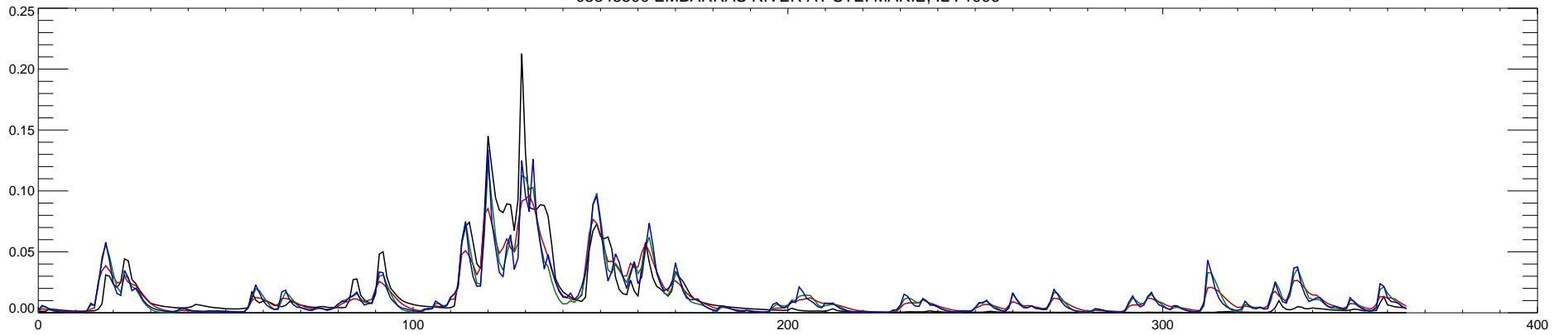
03345500 EMBARRAS RIVER AT STE. MARIE, IL : 1997
