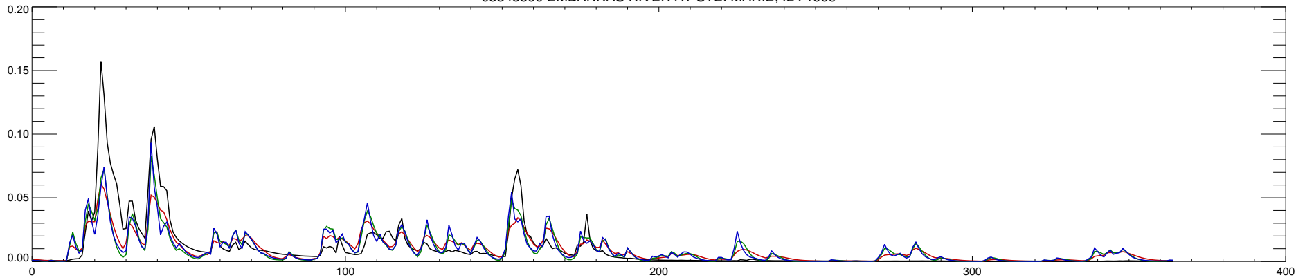
03345500 EMBARRAS RIVER AT STE. MARIE, IL : 2000
