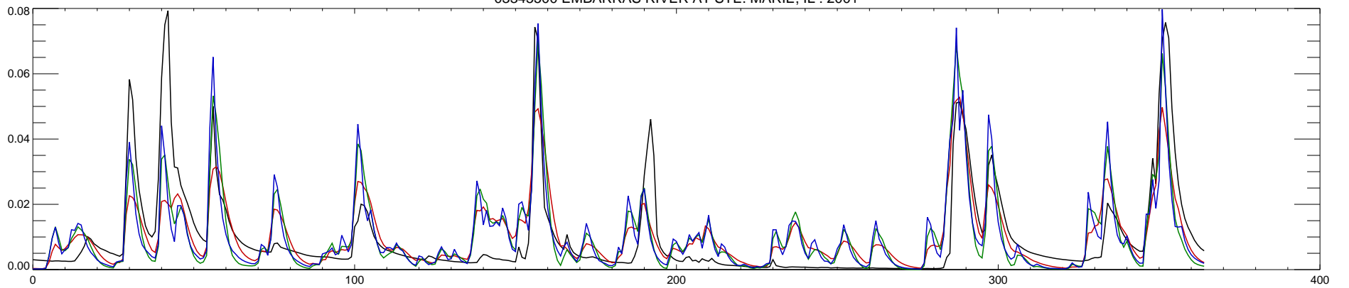
03345500 EMBARRAS RIVER AT STE. MARIE, IL : 2001
