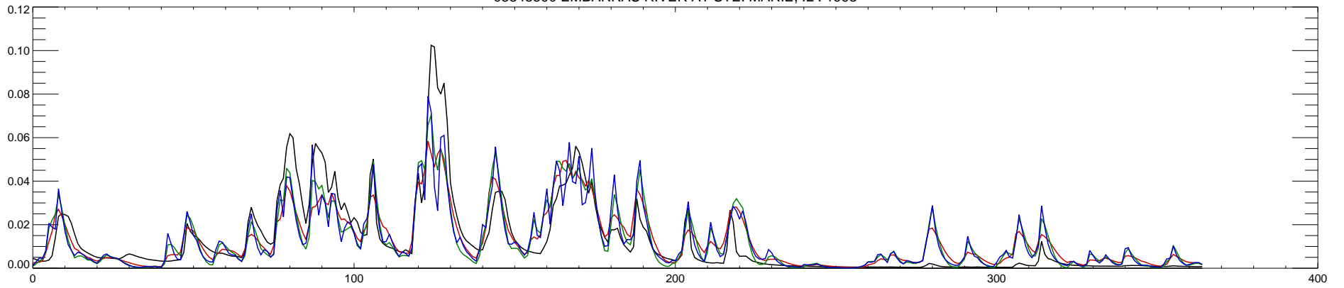
03345500 EMBARRAS RIVER AT STE. MARIE, IL : 1998
