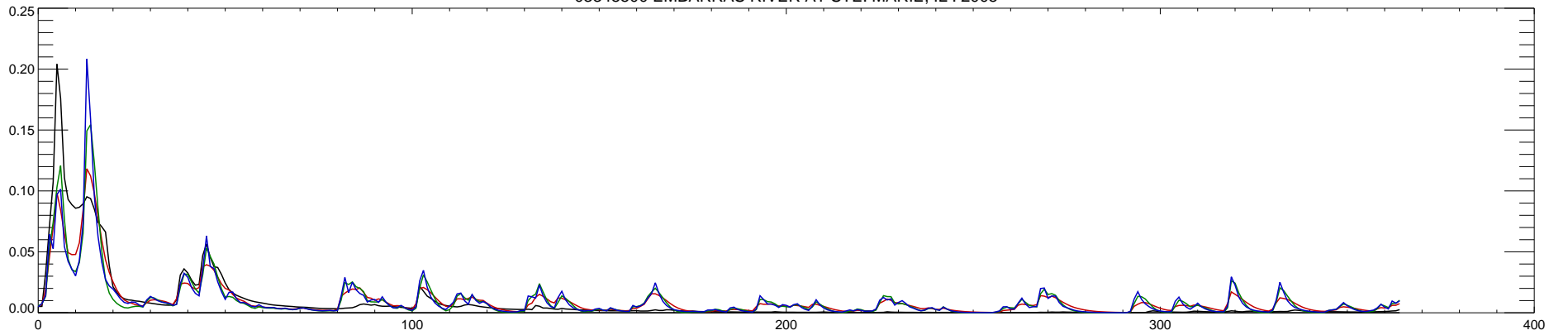
03345500 EMBARRAS RIVER AT STE. MARIE, IL : 2006
