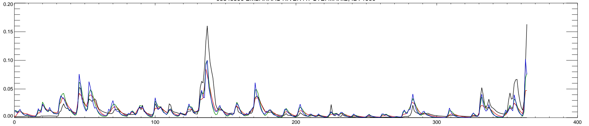
03345500 EMBARRAS RIVER AT STE. MARIE, IL : 1991
