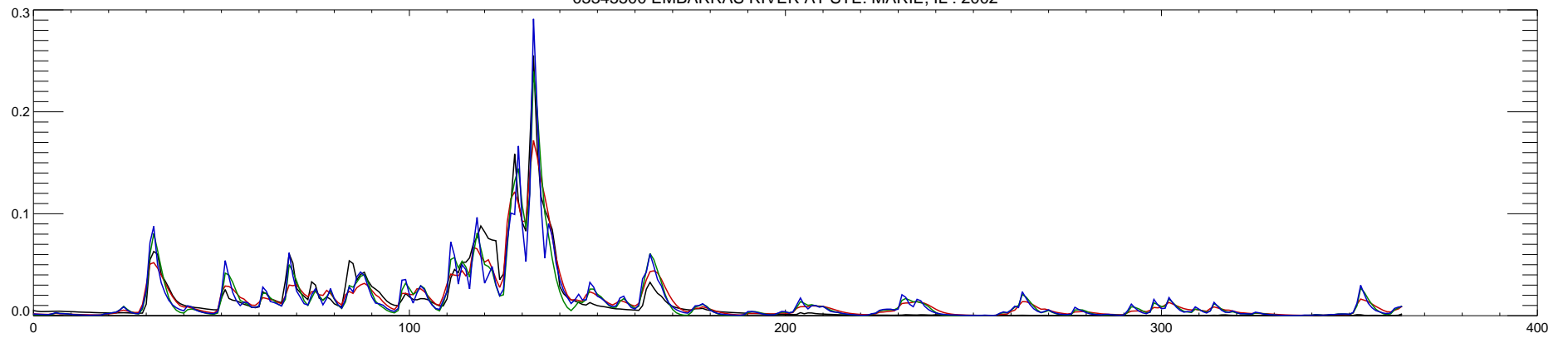
03345500 EMBARRAS RIVER AT STE. MARIE, IL : 2003
