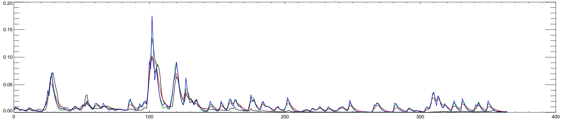
03345500 EMBARRAS RIVER AT STE. MARIE, IL : 1995
