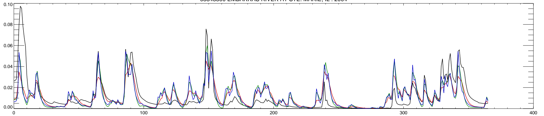
03345500 EMBARRAS RIVER AT STE. MARIE, IL : 2004
