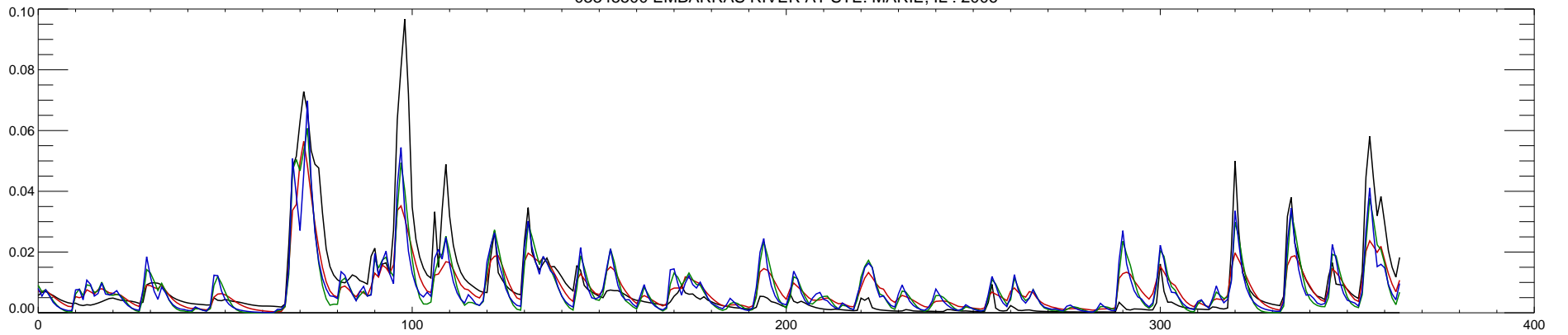
03345500 EMBARRAS RIVER AT STE. MARIE, IL : 2007
