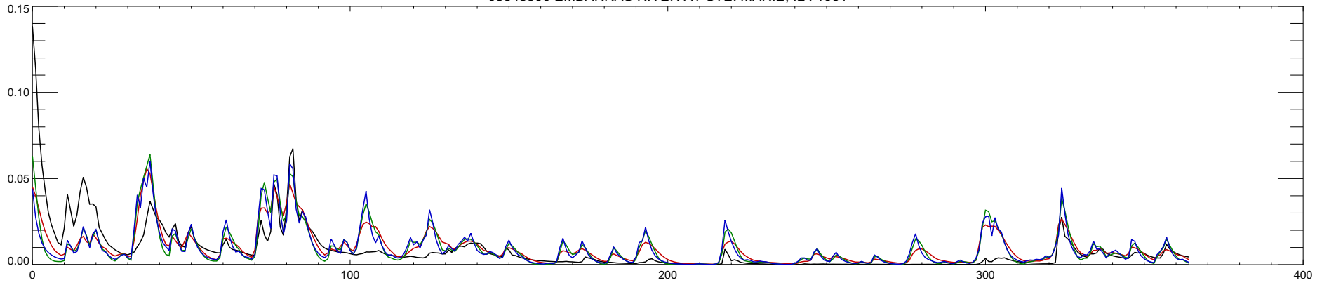
03345500 EMBARRAS RIVER AT STE. MARIE, IL : 1992
