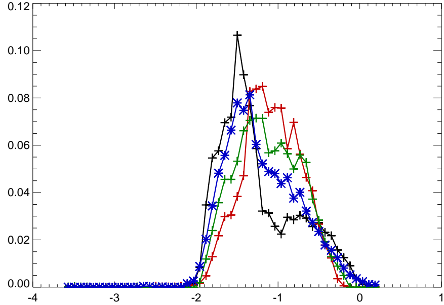
13168500 BRUNEAU RIVER NR HOT SPRING ID
