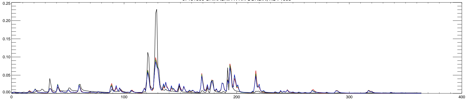
07151500 CHIKASKIA R NR CORBIN, KS : 1994
