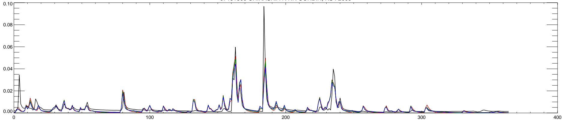
07151500 CHIKASKIA R NR CORBIN, KS : 2006
