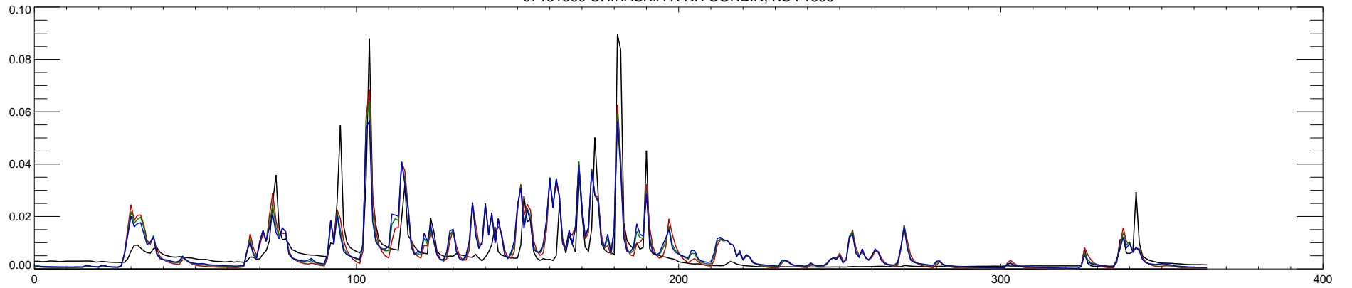
07151500 CHIKASKIA R NR CORBIN, KS : 2000
