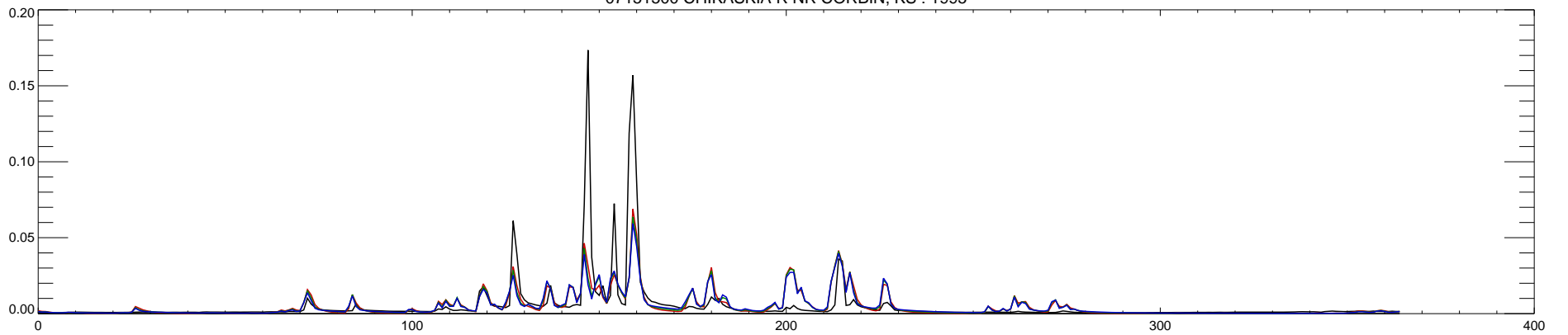
07151500 CHIKASKIA R NR CORBIN, KS : 1995
