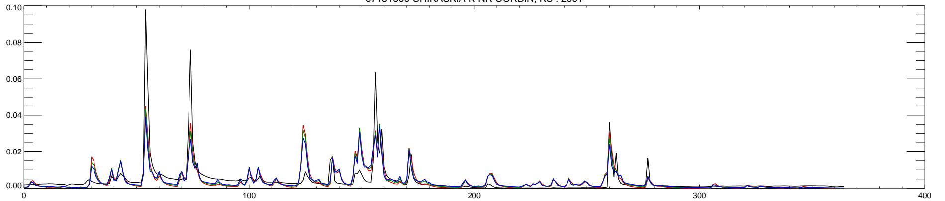
07151500 CHIKASKIA R NR CORBIN, KS : 2001
