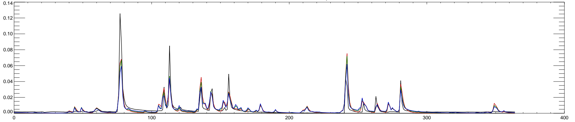
07151500 CHIKASKIA R NR CORBIN, KS : 2004
