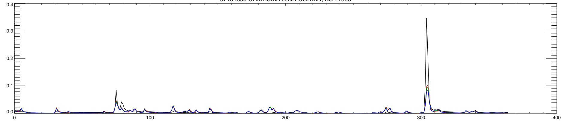
07151500 CHIKASKIA R NR CORBIN, KS : 1998
