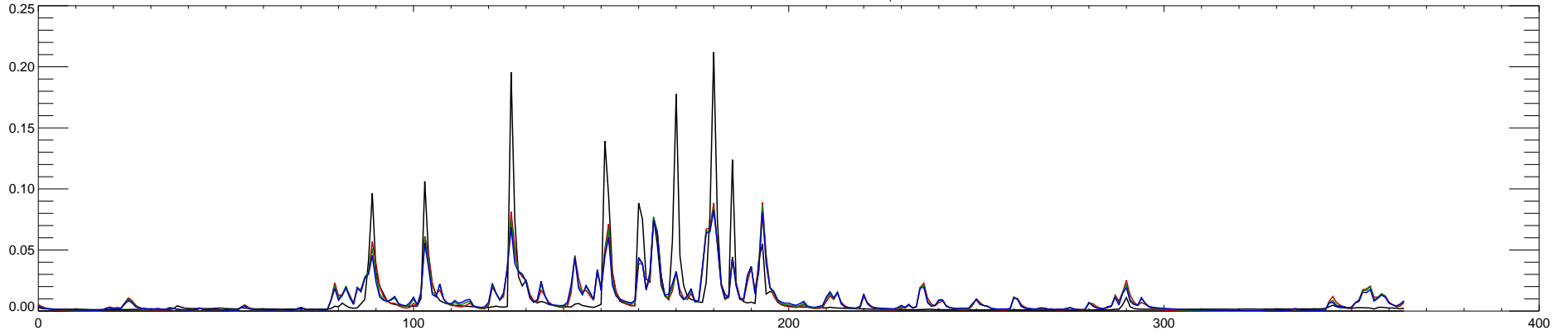
07151500 CHIKASKIA R NR CORBIN, KS : 2007
