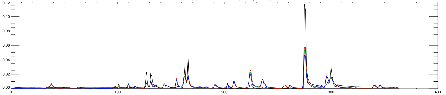
07151500 CHIKASKIA R NR CORBIN, KS : 2003
