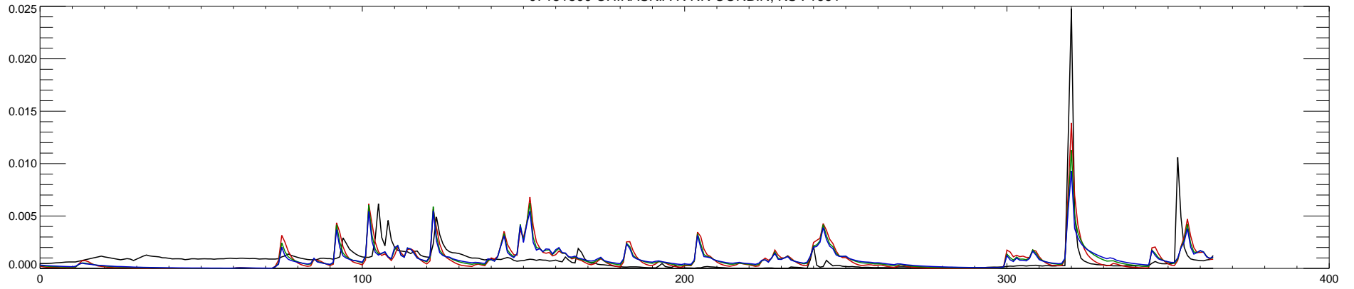
07151500 CHIKASKIA R NR CORBIN, KS : 1992
