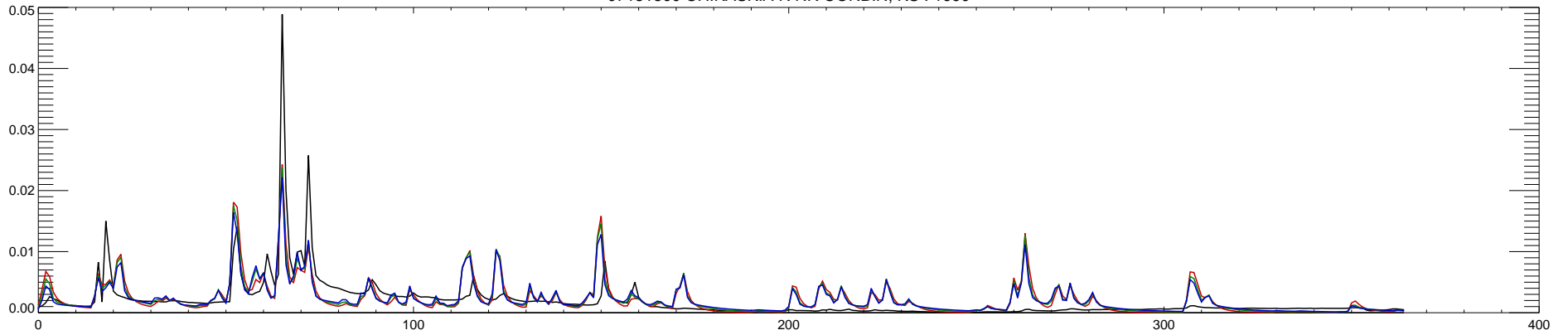
07151500 CHIKASKIA R NR CORBIN, KS : 1991
