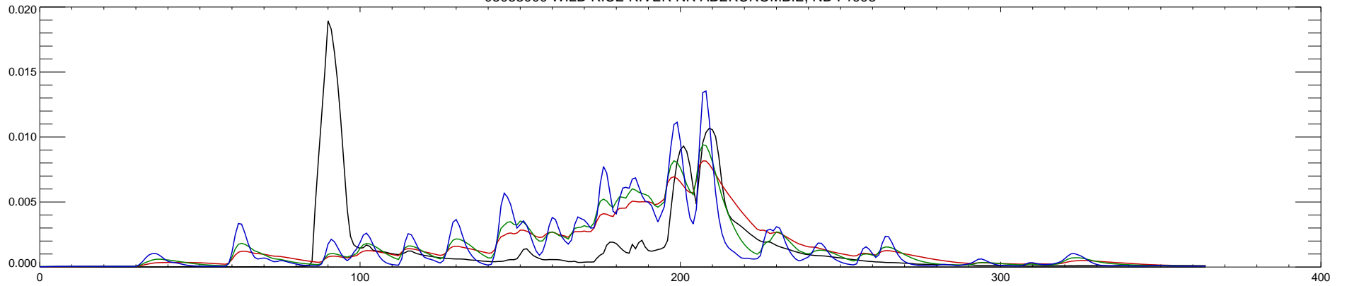
05053000 WILD RICE RIVER NR ABERCROMBIE, ND : 1994
