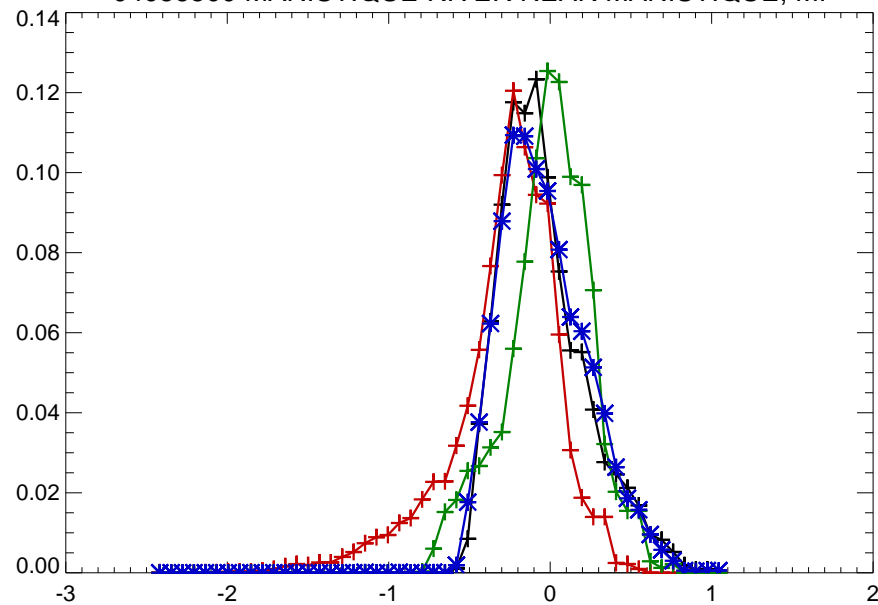
04056500 MANISTIQUE RIVER NEAR MANISTIQUE, MI
