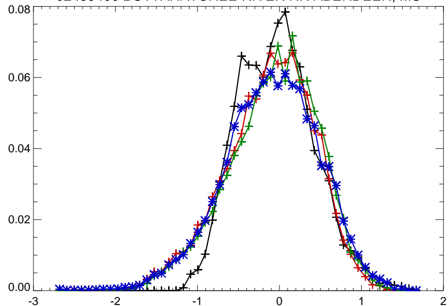
02439400 BUTTAHATCHEE RIVER NR ABERDEEN, MS
