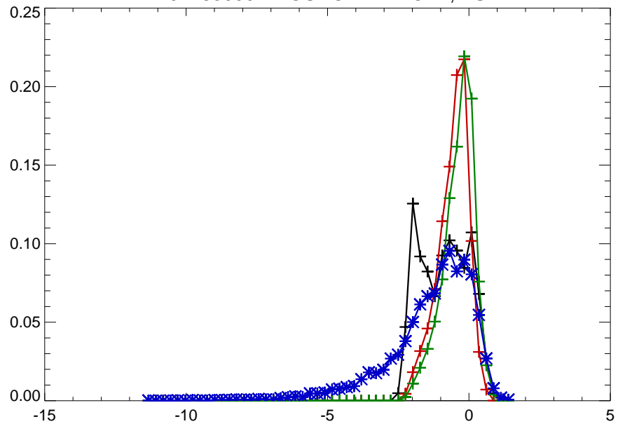
07183000 NEOSHO R NR IOLA, KS
