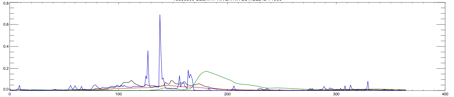
13336500 SELWAY RIVER NR LOWELL ID : 1991
