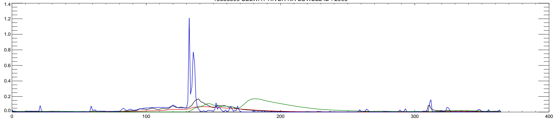
13336500 SELWAY RIVER NR LOWELL ID : 2007
