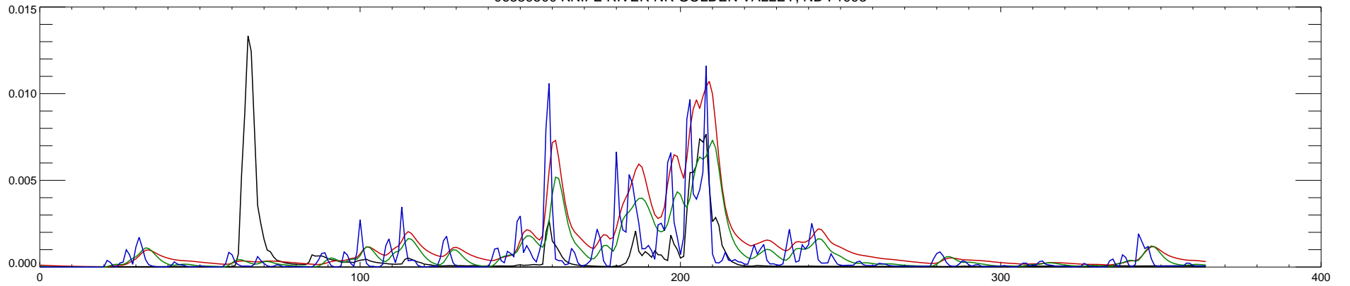
06339500 KNIFE RIVER NR GOLDEN VALLEY, ND : 1994
