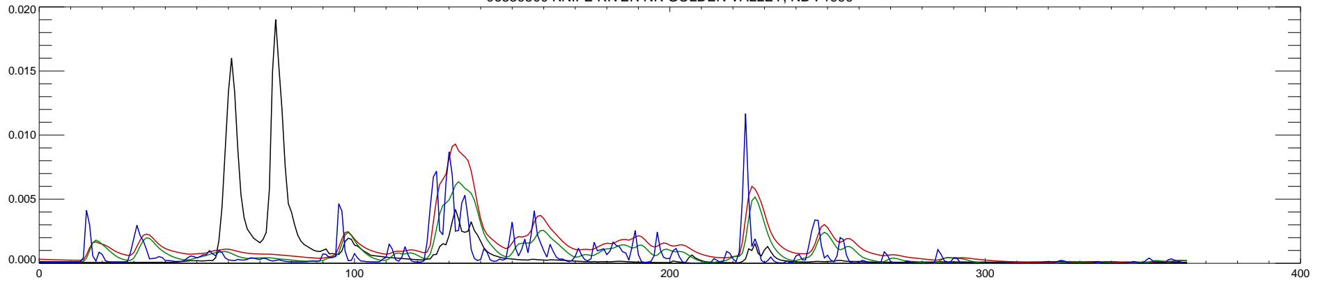
06339500 KNIFE RIVER NR GOLDEN VALLEY, ND : 2000
