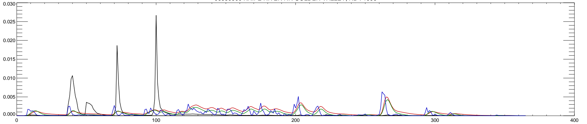
06339500 KNIFE RIVER NR GOLDEN VALLEY, ND : 1997
