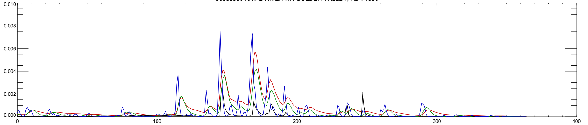
06339500 KNIFE RIVER NR GOLDEN VALLEY, ND : 1991
