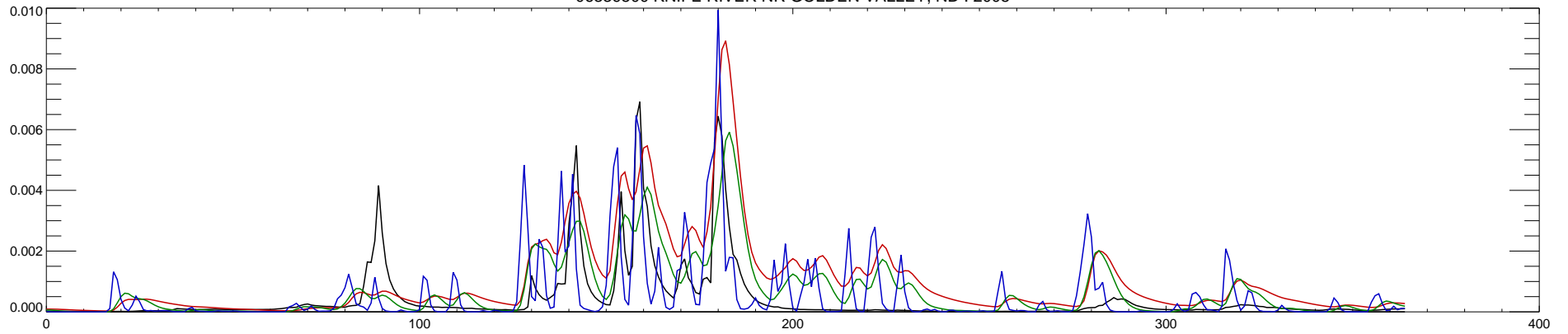
06339500 KNIFE RIVER NR GOLDEN VALLEY, ND : 2006
