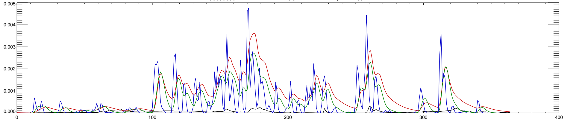
06339500 KNIFE RIVER NR GOLDEN VALLEY, ND : 1992
