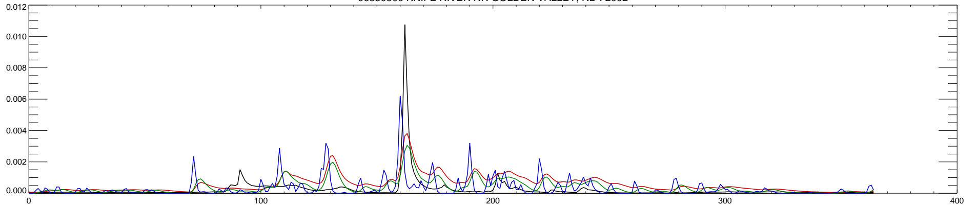
06339500 KNIFE RIVER NR GOLDEN VALLEY, ND : 2003
