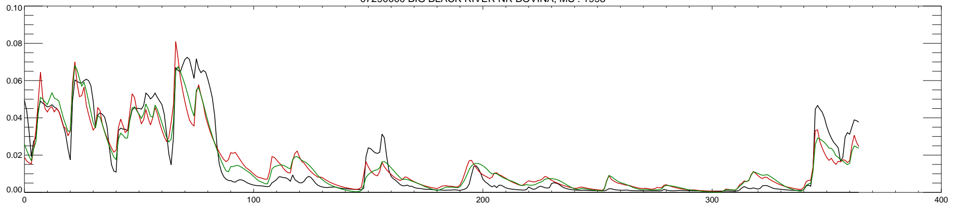
07290000 BIG BLACK RIVER NR BOVINA, MS : 1999
