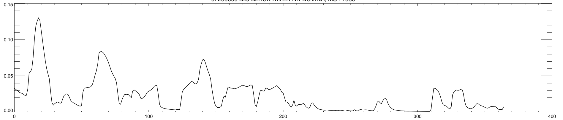
07290000 BIG BLACK RIVER NR BOVINA, MS : 1990
