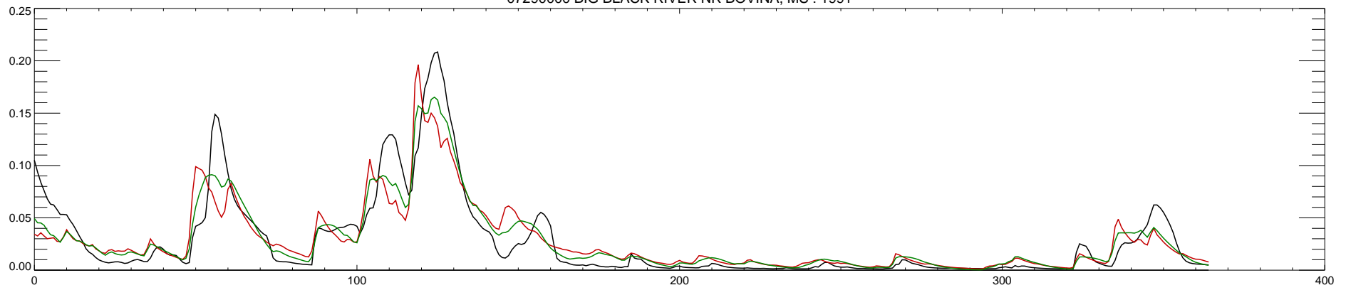
07290000 BIG BLACK RIVER NR BOVINA, MS : 1991
