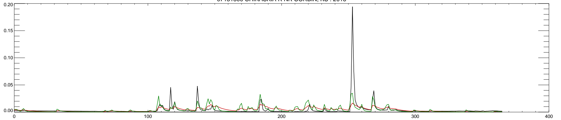
07151500 CHIKASKIA R NR CORBIN, KS : 2016
