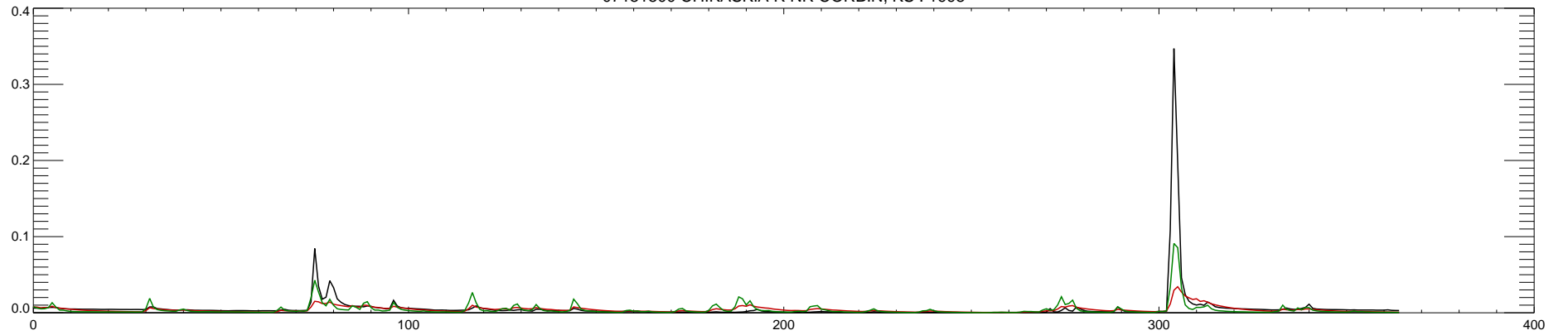
07151500 CHIKASKIA R NR CORBIN, KS : 1999
