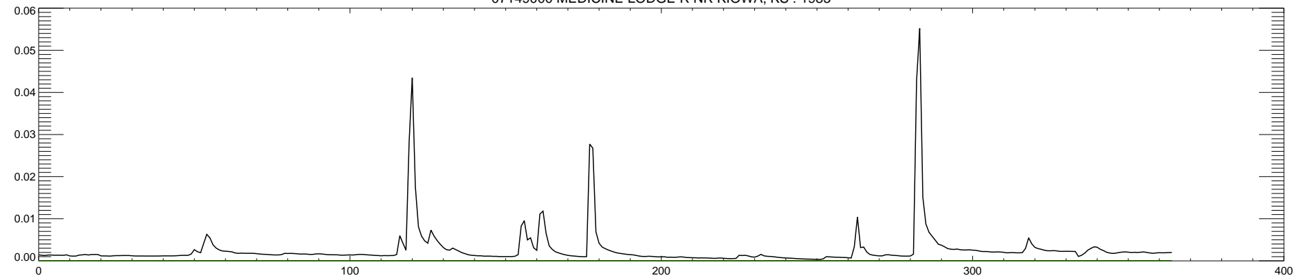
07149000 MEDICINE LODGE R NR KIOWA, KS : 1985
