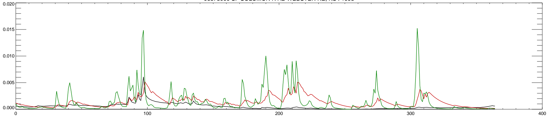
06873000 SF SOLOMON R AB WEBSTER RE, KS : 1999
