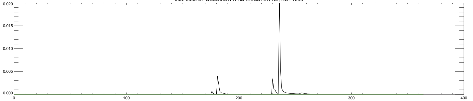
06873000 SF SOLOMON R AB WEBSTER RE, KS : 1990
