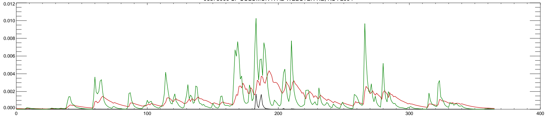
06873000 SF SOLOMON R AB WEBSTER RE, KS : 2005
