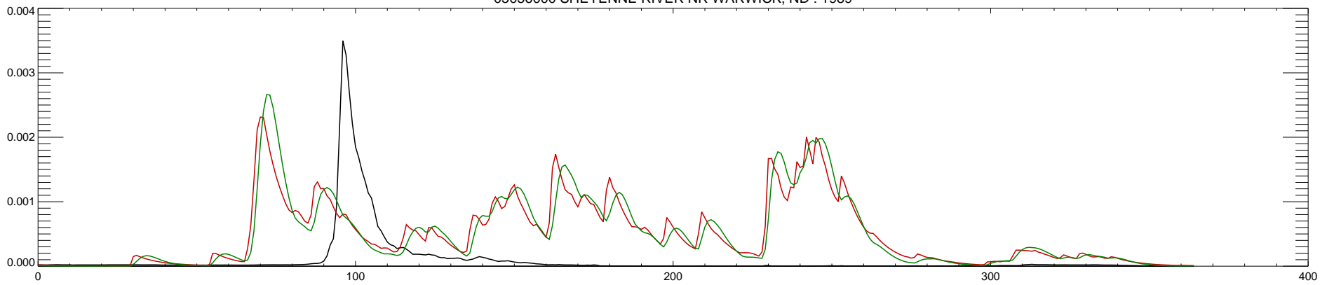
05056000 SHEYENNE RIVER NR WARWICK, ND : 1990
