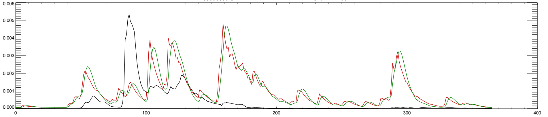
05056000 SHEYENNE RIVER NR WARWICK, ND : 1985
