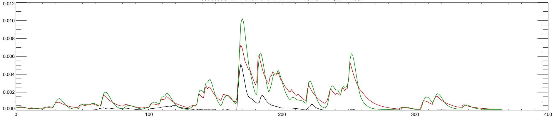
05053000 WILD RICE RIVER NR ABERCROMBIE, ND : 1993
