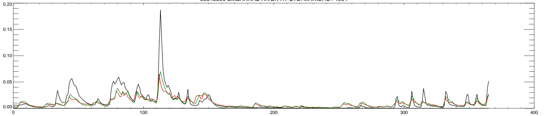
03345500 EMBARRAS RIVER AT STE. MARIE, IL : 1985
