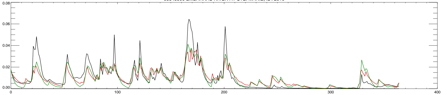
03345500 EMBARRAS RIVER AT STE. MARIE, IL : 2011
