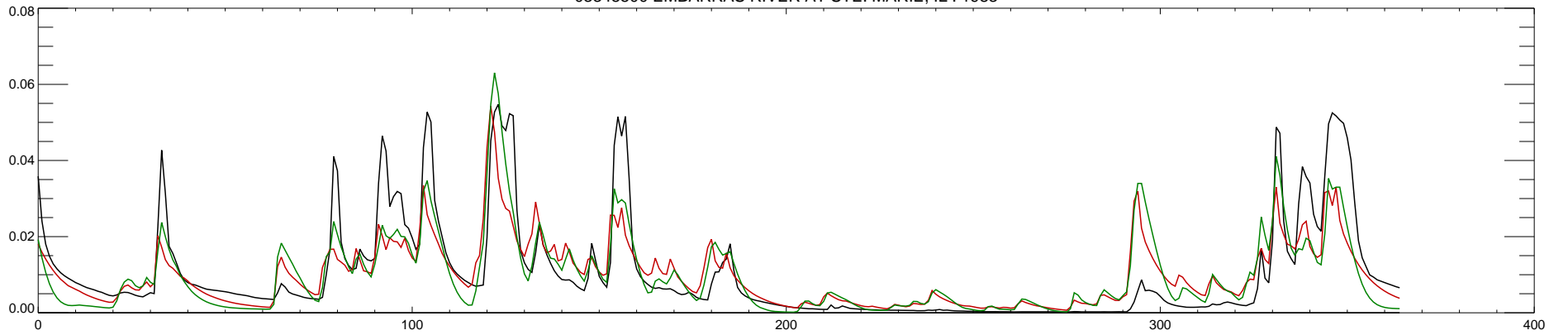
03345500 EMBARRAS RIVER AT STE. MARIE, IL : 1984
