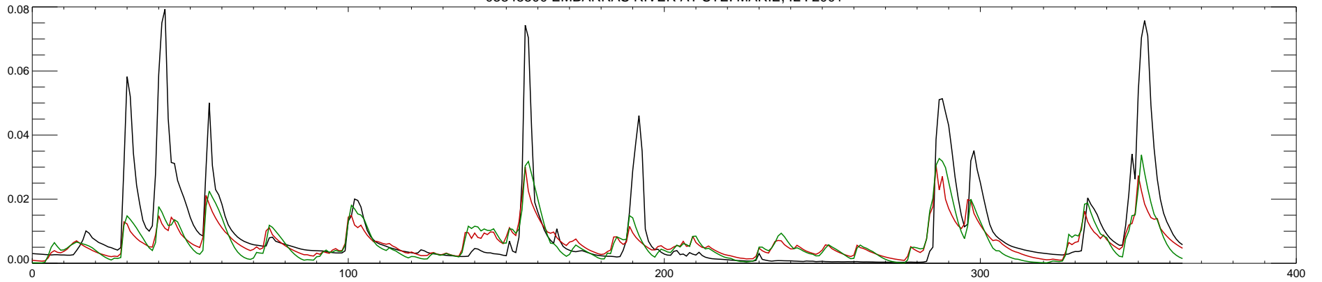
03345500 EMBARRAS RIVER AT STE. MARIE, IL : 2002
