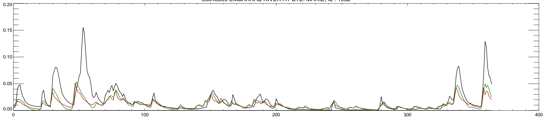
03345500 EMBARRAS RIVER AT STE. MARIE, IL : 1982
