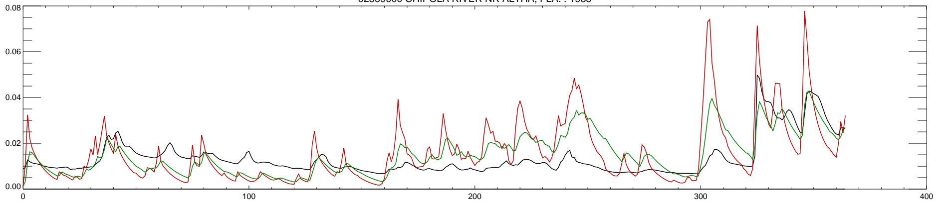
02359000 CHIPOLA RIVER NR ALTHA, FLA. : 1985
