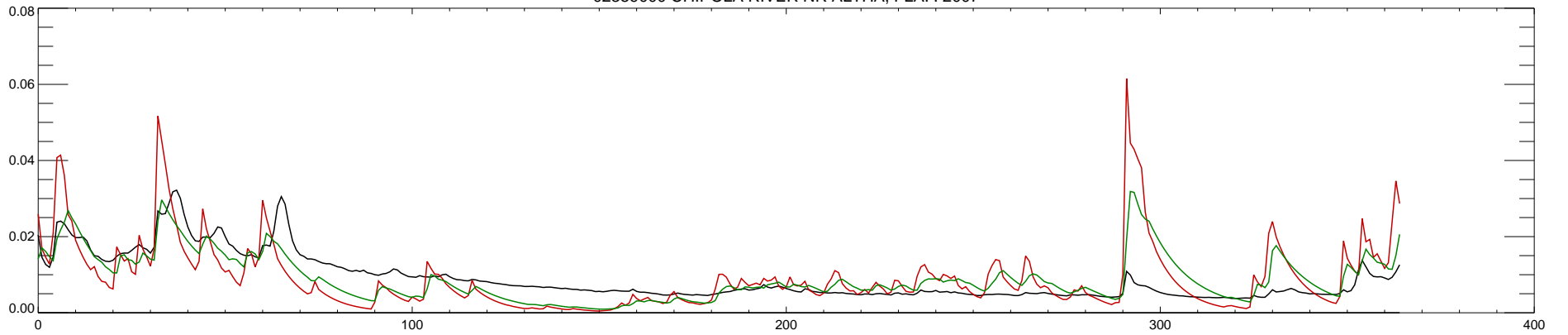
02359000 CHIPOLA RIVER NR ALTHA, FLA. : 2008
