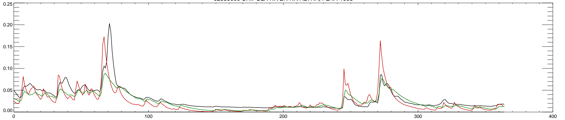
02359000 CHIPOLA RIVER NR ALTHA, FLA. : 1999
