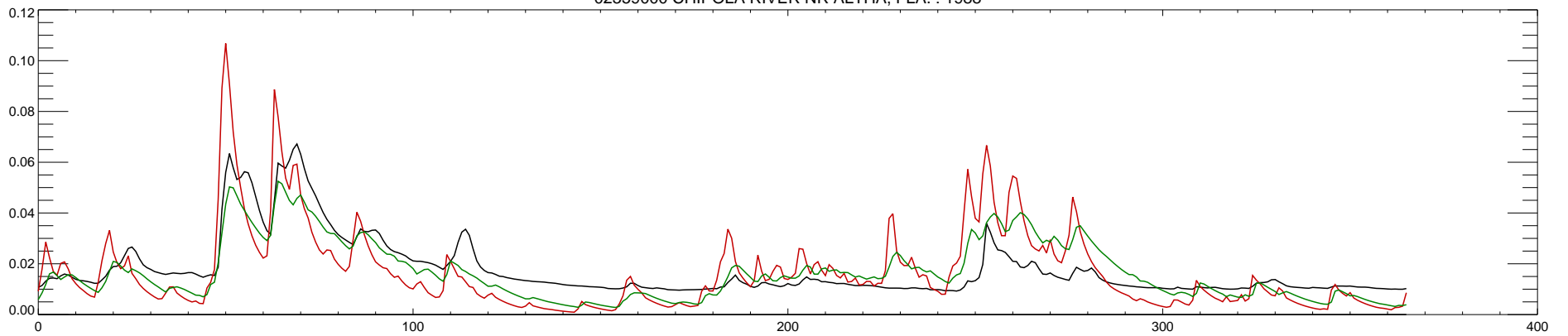
02359000 CHIPOLA RIVER NR ALTHA, FLA. : 1988
