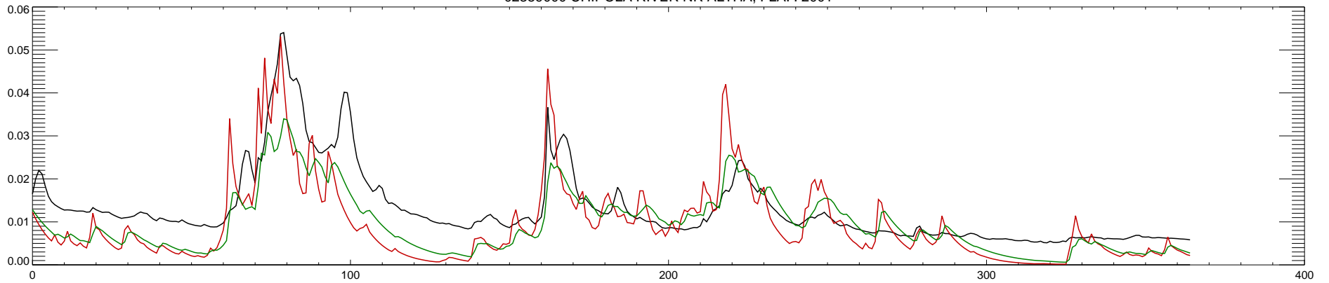
02359000 CHIPOLA RIVER NR ALTHA, FLA. : 2002
