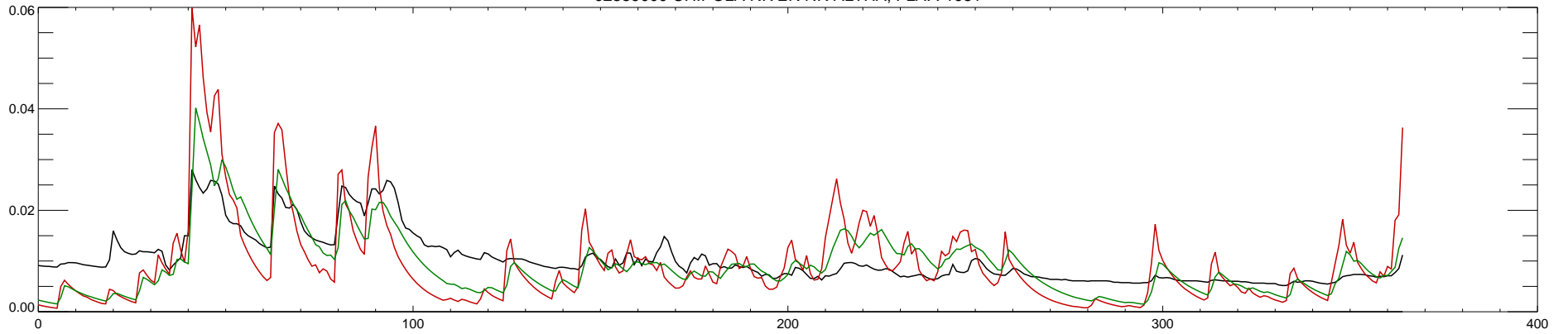
02359000 CHIPOLA RIVER NR ALTHA, FLA. : 1982
