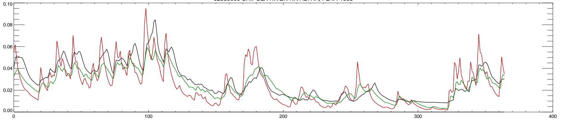
02359000 CHIPOLA RIVER NR ALTHA, FLA. : 1984
