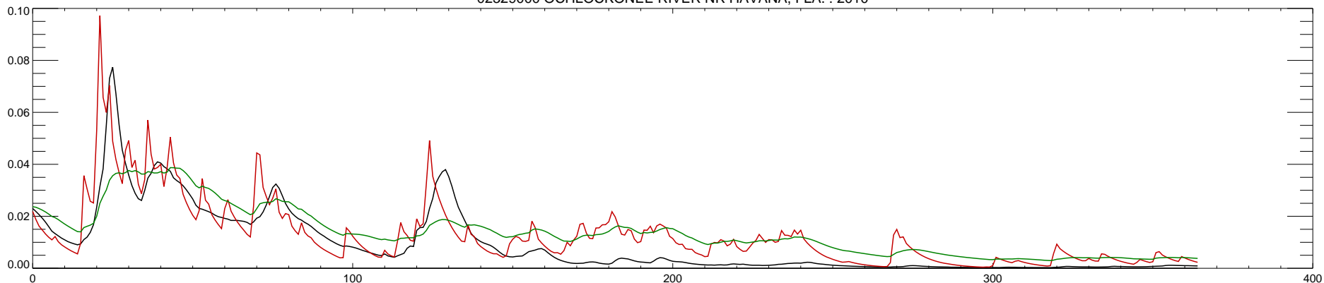
02329000 OCHLOCKONEE RIVER NR HAVANA, FLA. : 2011
