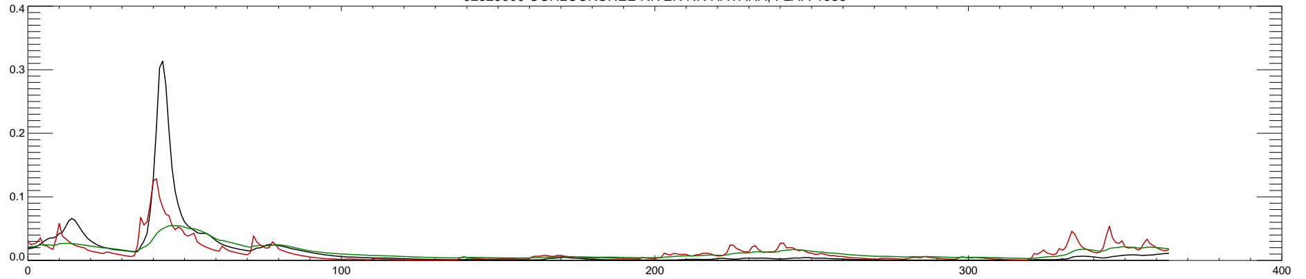
02329000 OCHLOCKONEE RIVER NR HAVANA, FLA. : 1987
