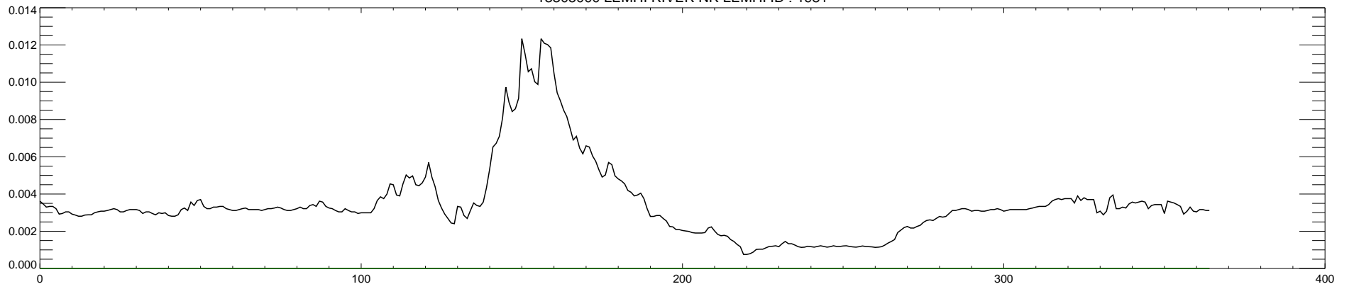
13305000 LEMHI RIVER NR LEMHI ID : 1982
