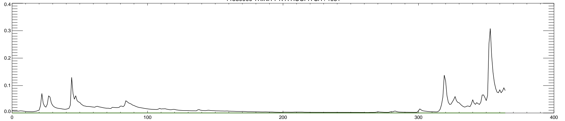
11530000 TRINITY R A HOOPA CA : 1982
