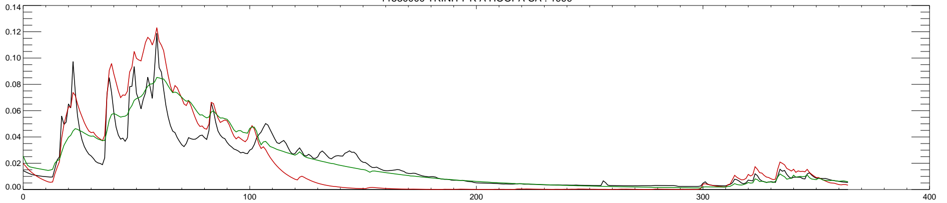
11530000 TRINITY R A HOOPA CA : 2000
