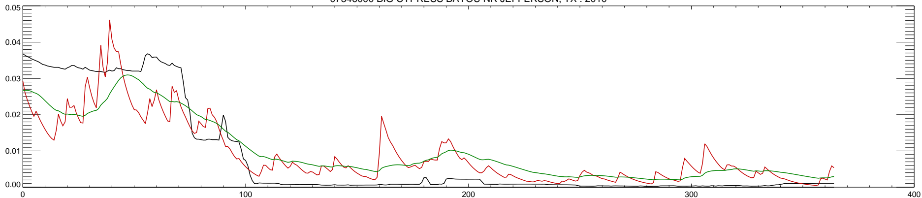
07346000 BIG CYPRESS BAYOU NR JEFFERSON, TX : 2011
