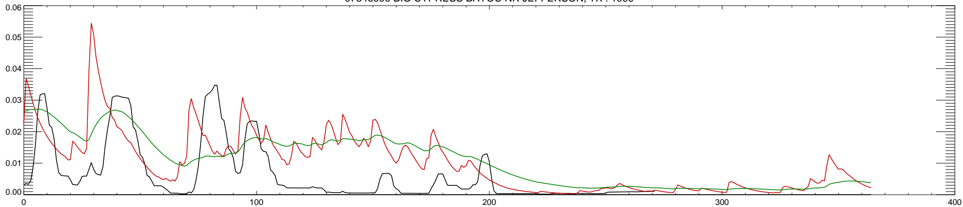
07346000 BIG CYPRESS BAYOU NR JEFFERSON, TX : 2000
