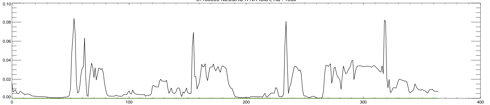
07183000 NEOSHO R NR IOLA, KS : 1985
