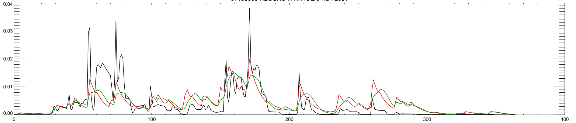
07183000 NEOSHO R NR IOLA, KS : 2002
