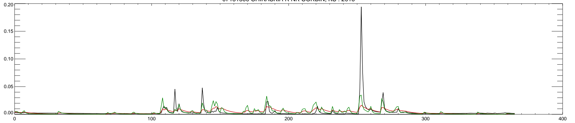
07151500 CHIKASKIA R NR CORBIN, KS : 2016
