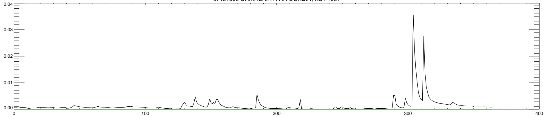
07151500 CHIKASKIA R NR CORBIN, KS : 1982
