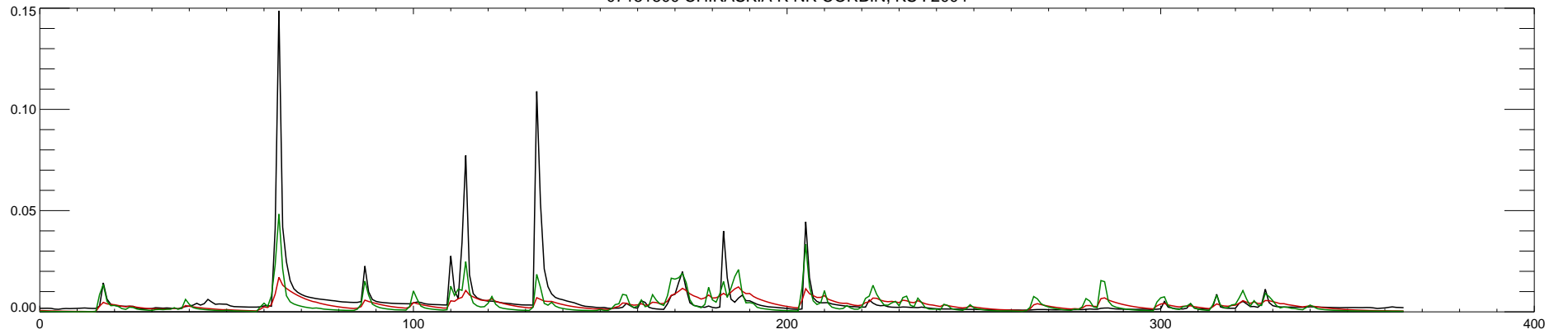
07151500 CHIKASKIA R NR CORBIN, KS : 2005
