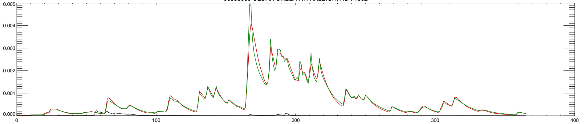
06353000 CEDAR CREEK NR RALEIGH, ND : 1993
