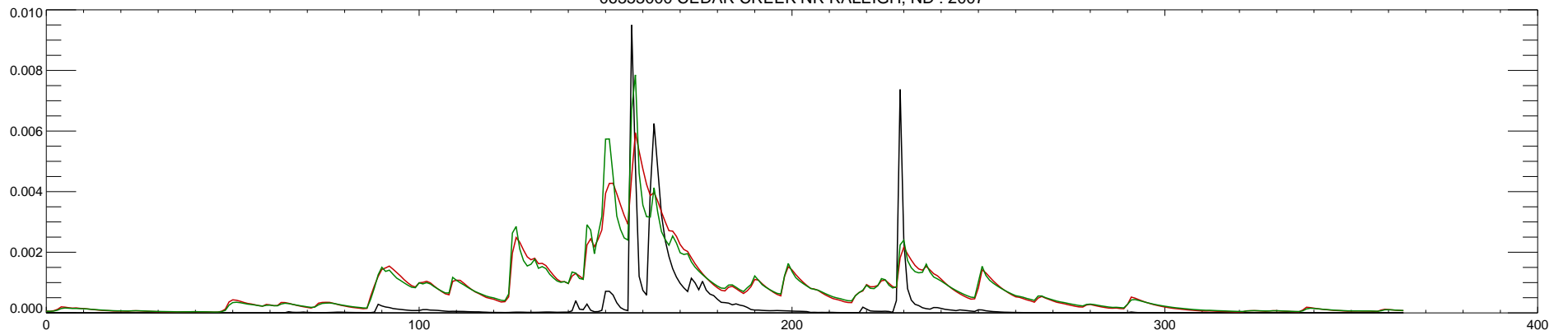
06353000 CEDAR CREEK NR RALEIGH, ND : 2008
