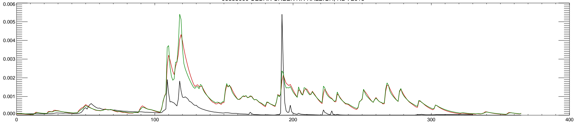
06353000 CEDAR CREEK NR RALEIGH, ND : 2016
