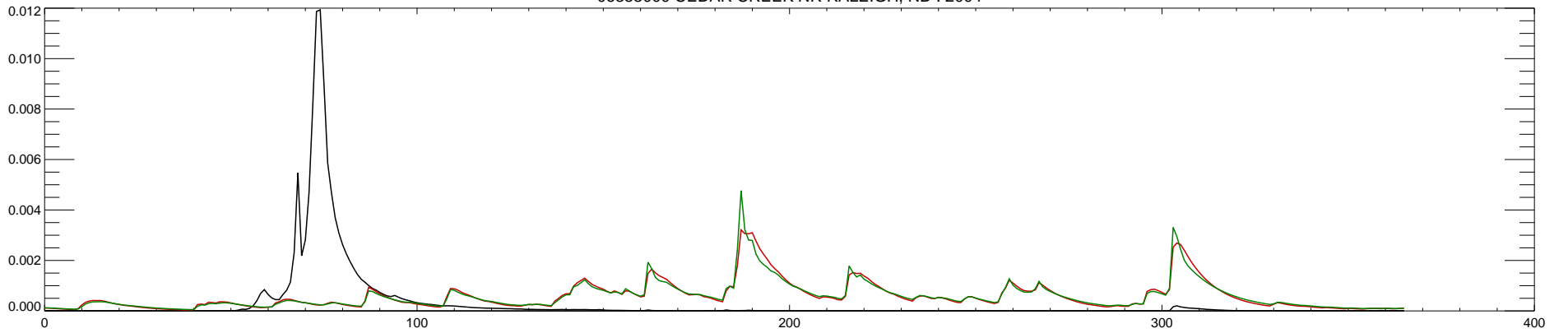
06353000 CEDAR CREEK NR RALEIGH, ND : 2005
