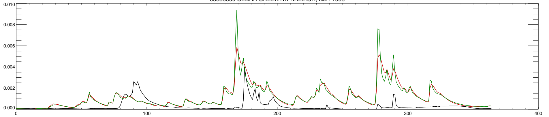
06353000 CEDAR CREEK NR RALEIGH, ND : 1999
