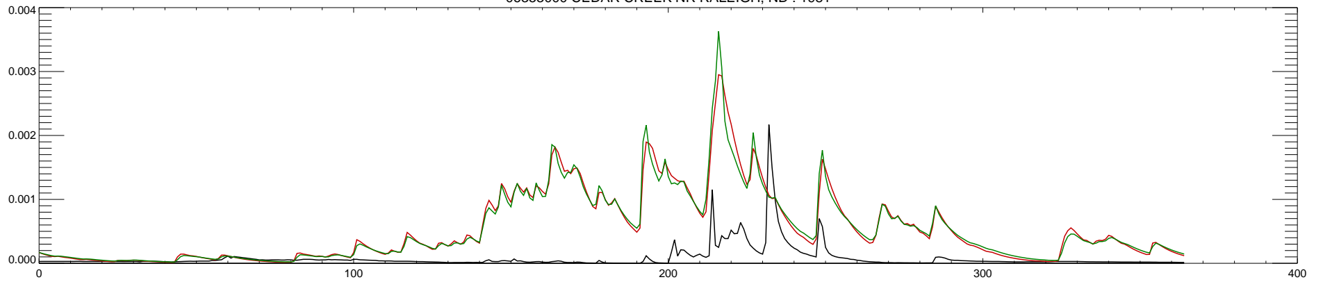
06353000 CEDAR CREEK NR RALEIGH, ND : 1982
