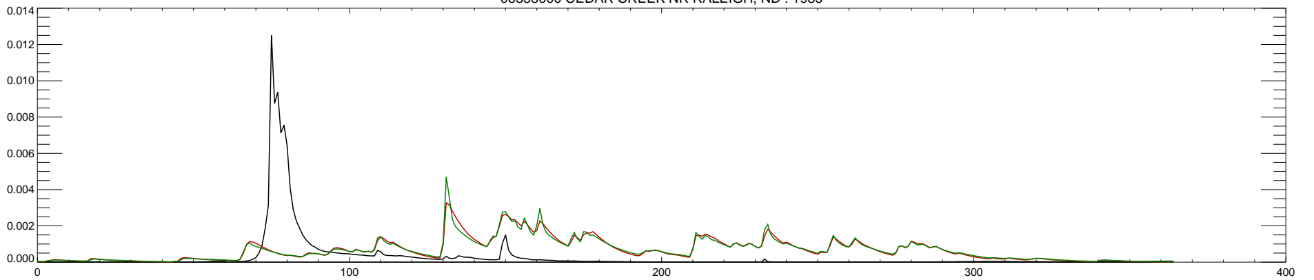
06353000 CEDAR CREEK NR RALEIGH, ND : 1985
