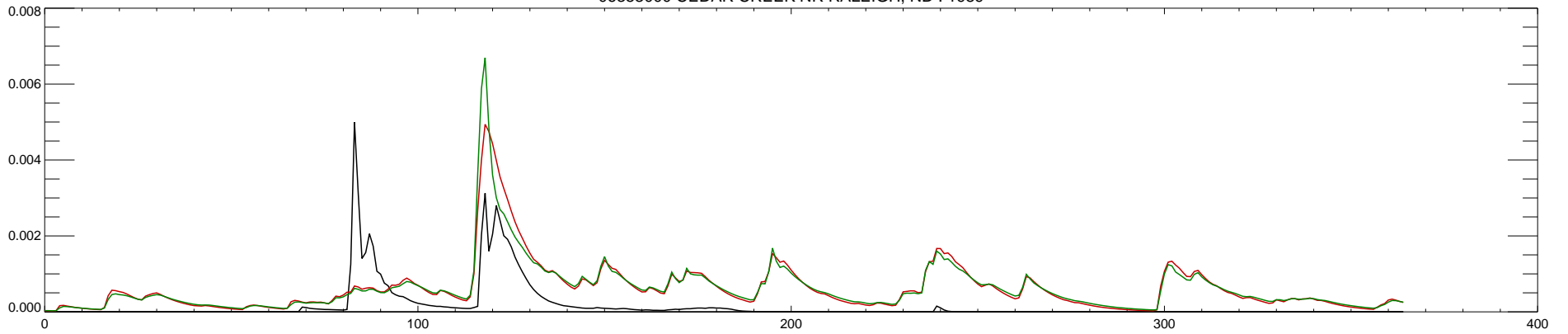
06353000 CEDAR CREEK NR RALEIGH, ND : 1990
