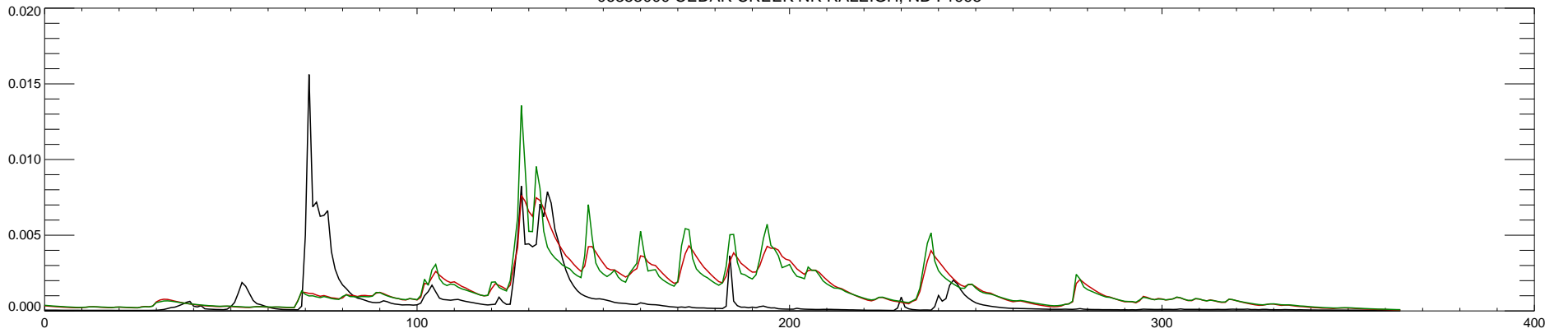
06353000 CEDAR CREEK NR RALEIGH, ND : 1996
