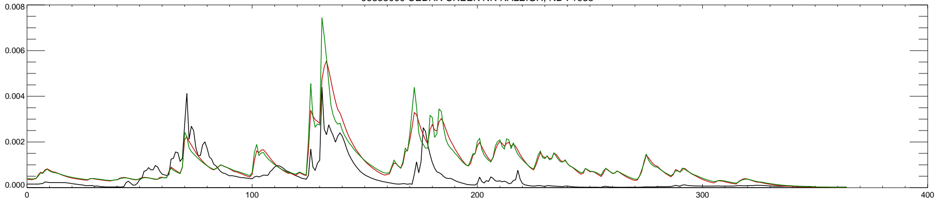
06353000 CEDAR CREEK NR RALEIGH, ND : 1984
