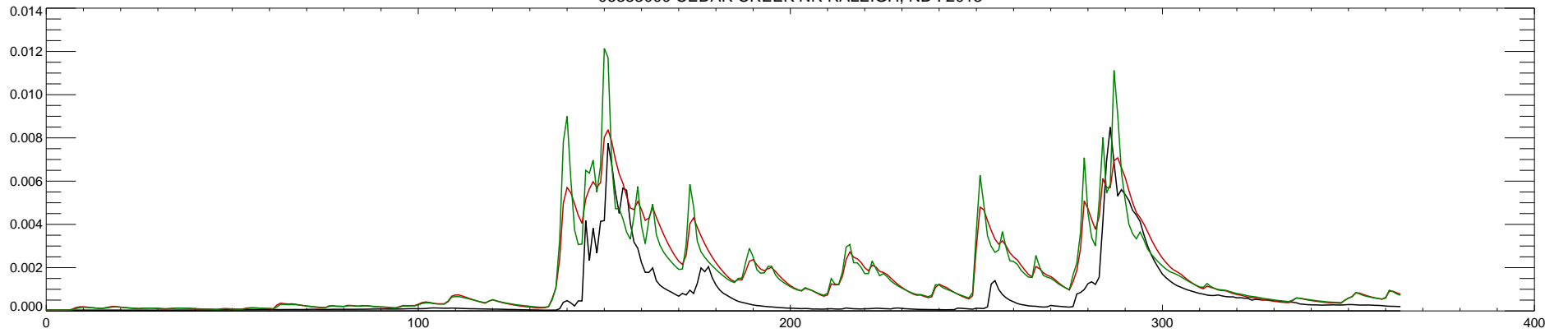
06353000 CEDAR CREEK NR RALEIGH, ND : 2014
