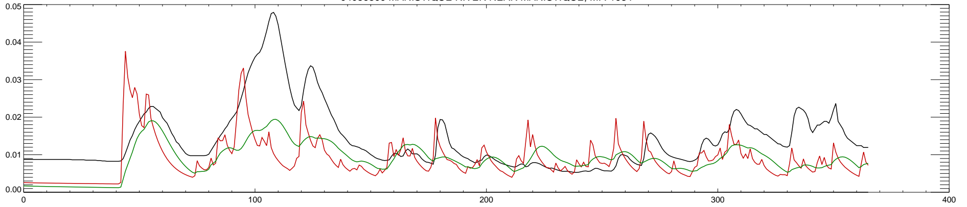
04056500 MANISTIQUE RIVER NEAR MANISTIQUE, MI : 1985
