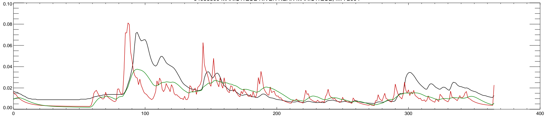
04056500 MANISTIQUE RIVER NEAR MANISTIQUE, MI : 2005
