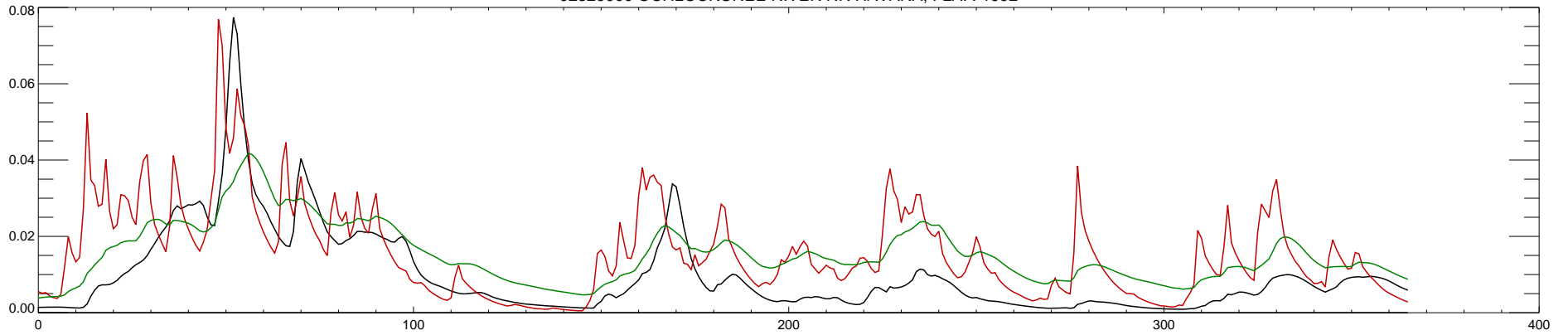
02329000 OCHLOCKONEE RIVER NR HAVANA, FLA. : 1993
